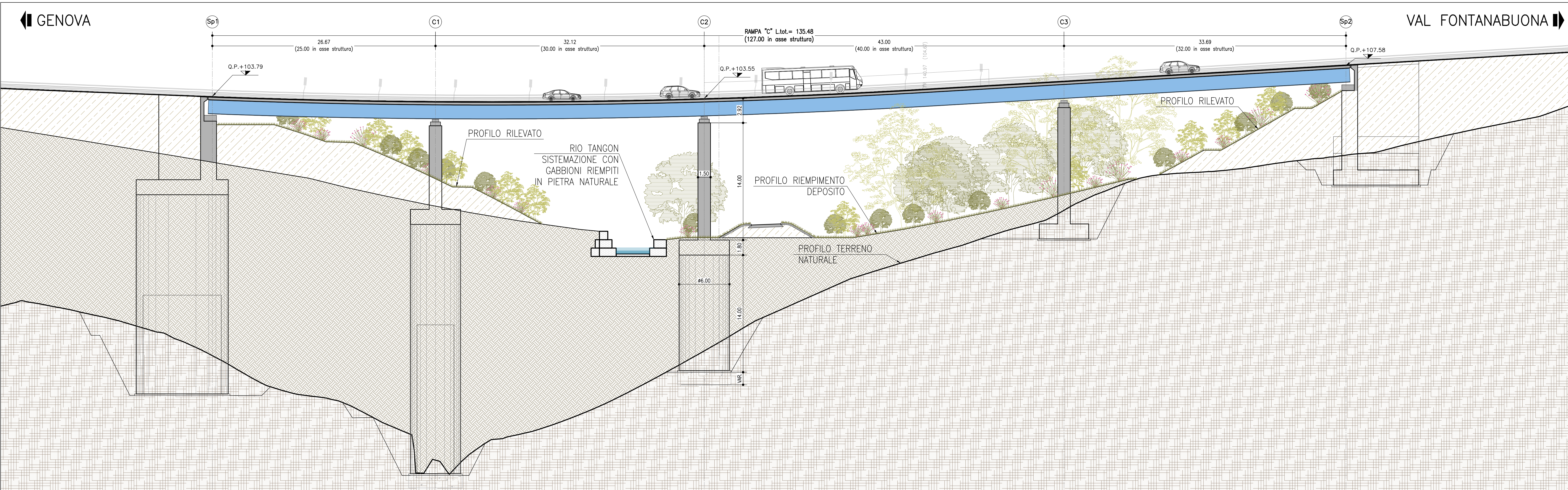
Prospetto A-A' (lato nord) - Scala 1:200
