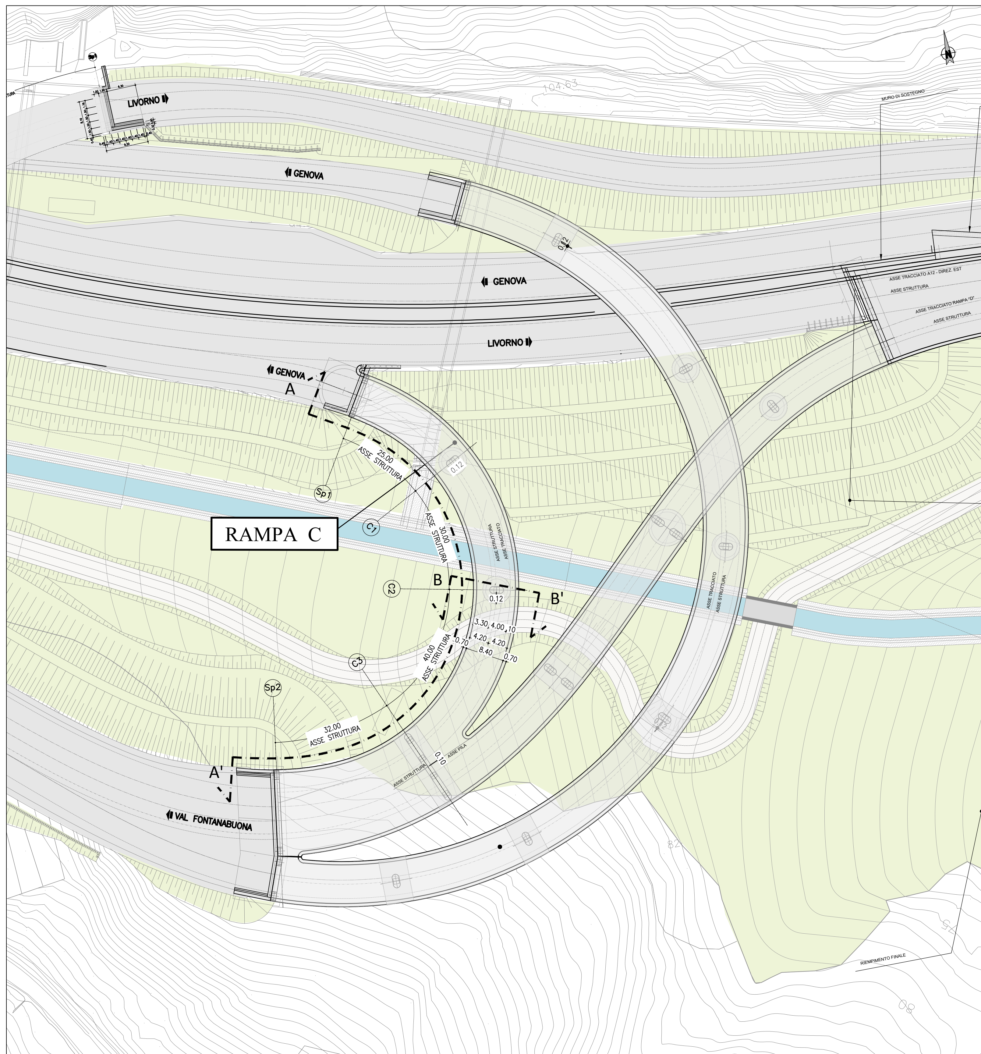
Planimetria di dettaglio dell'impronta a terra delle opere di fondazione - Scala 1:500
