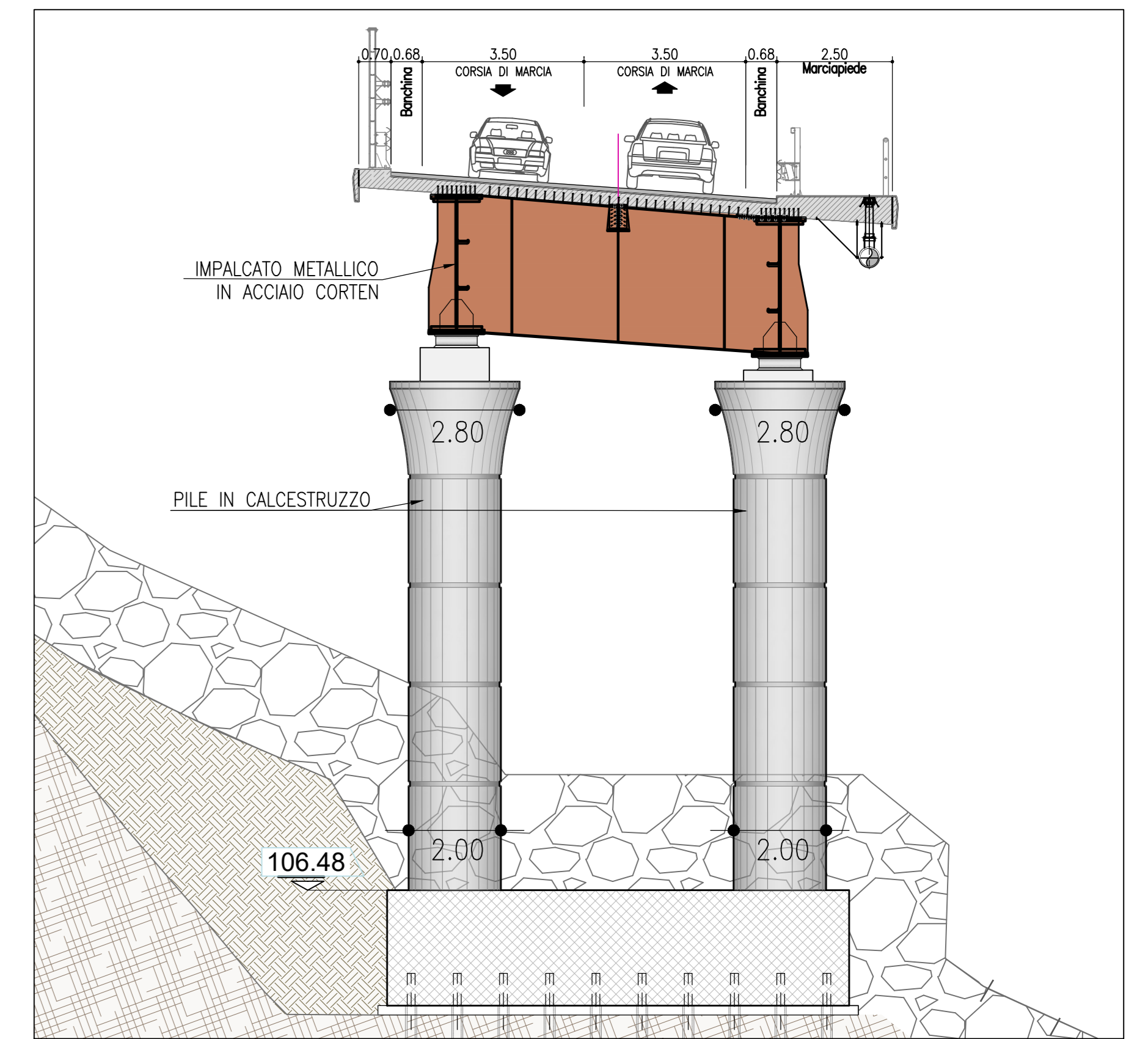
Sezione C-C' (Pila e Impalcato) - Scala 1:100
