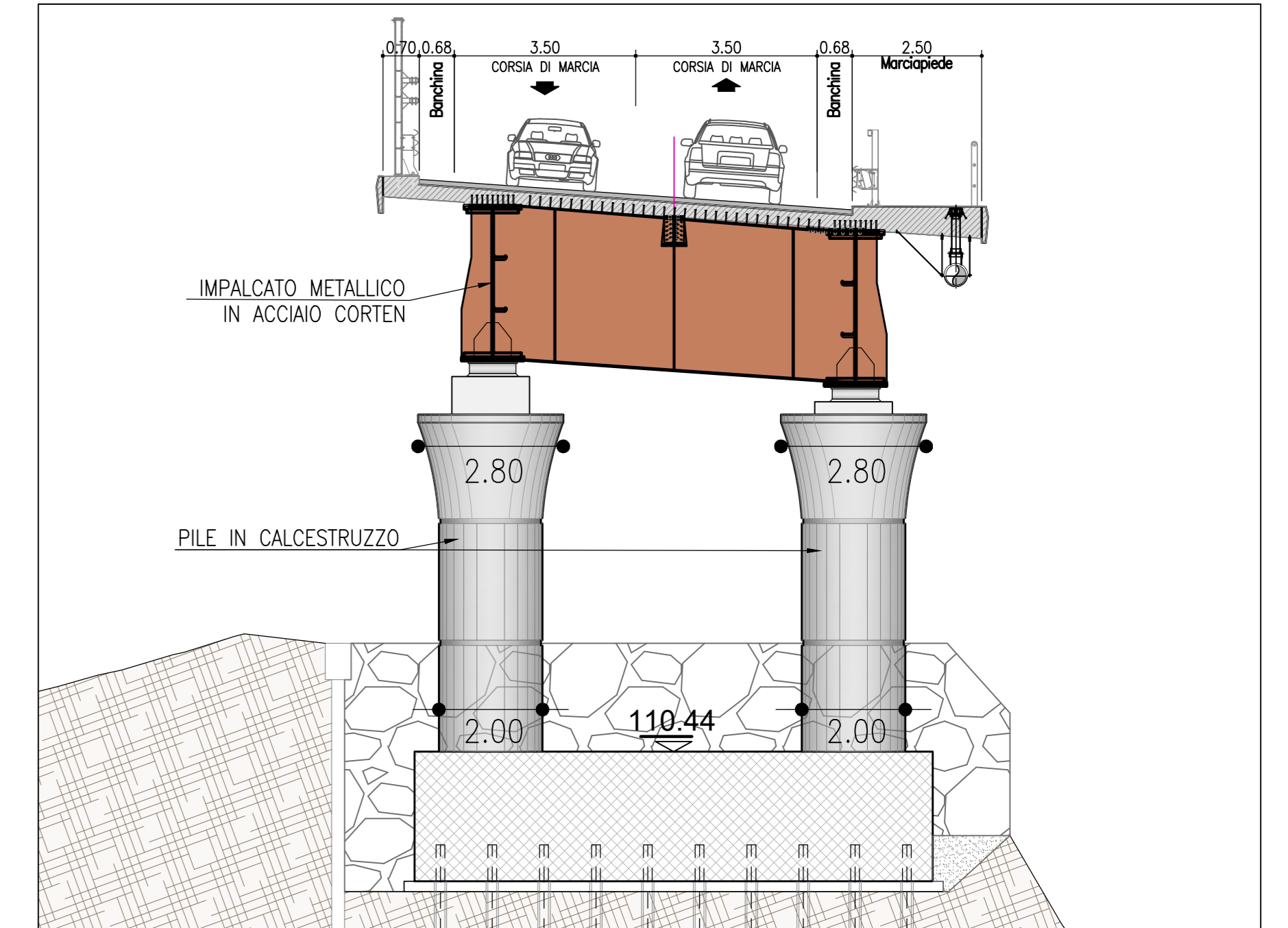
Sezione B-B' (Pila e Impalcato) - Scala 1:100
