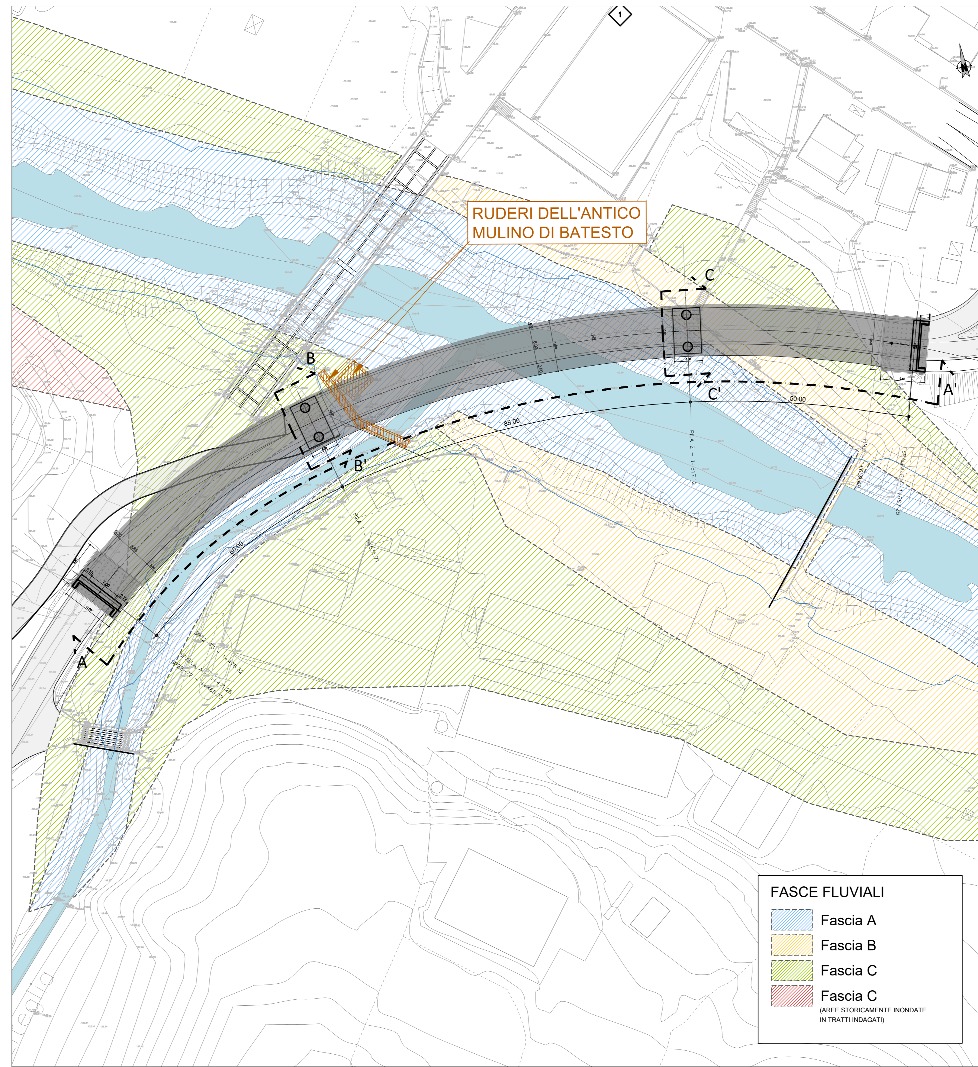
Planimetria di dettaglio dell'impronta a terra della opere di fondazione con le fasce di esondazione - Scala 1:500
