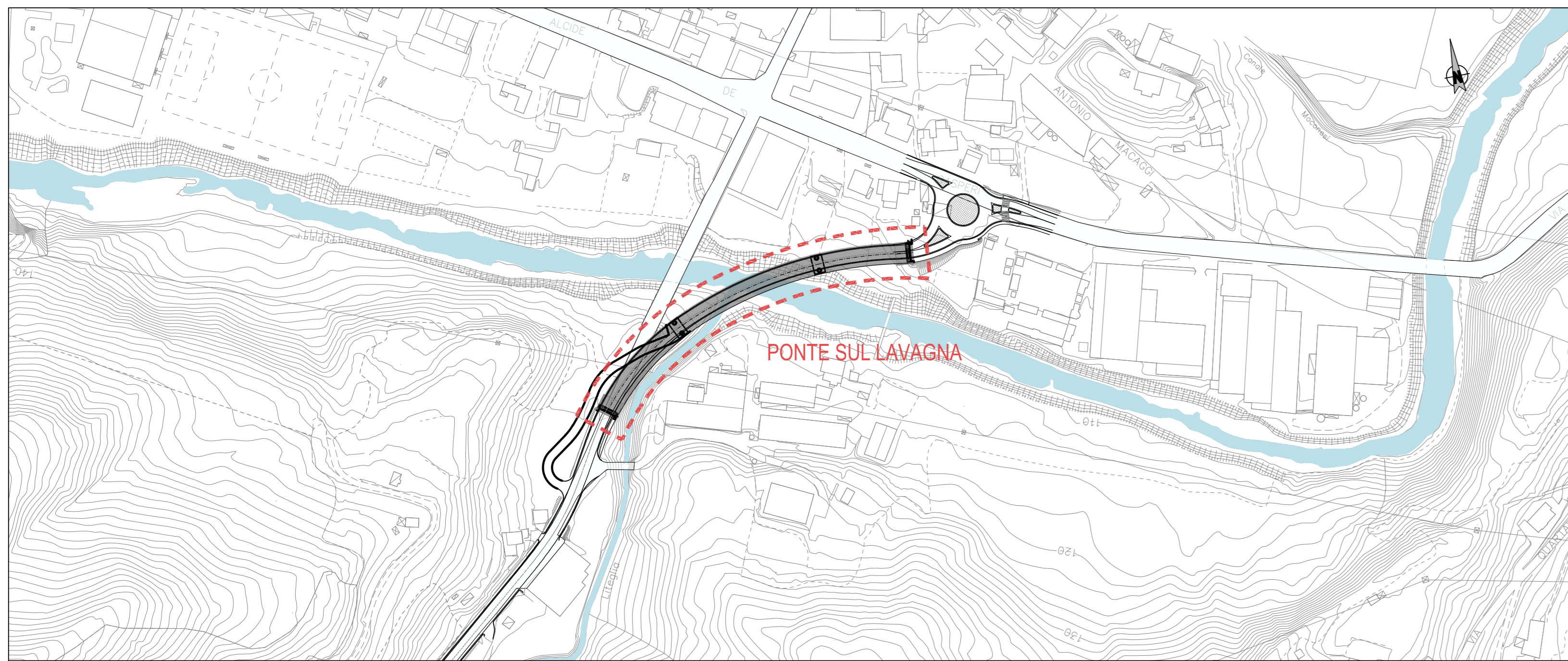
Planimetria di progetto del Viadotto sul Torrente Lavagna - Scala 1:2000
