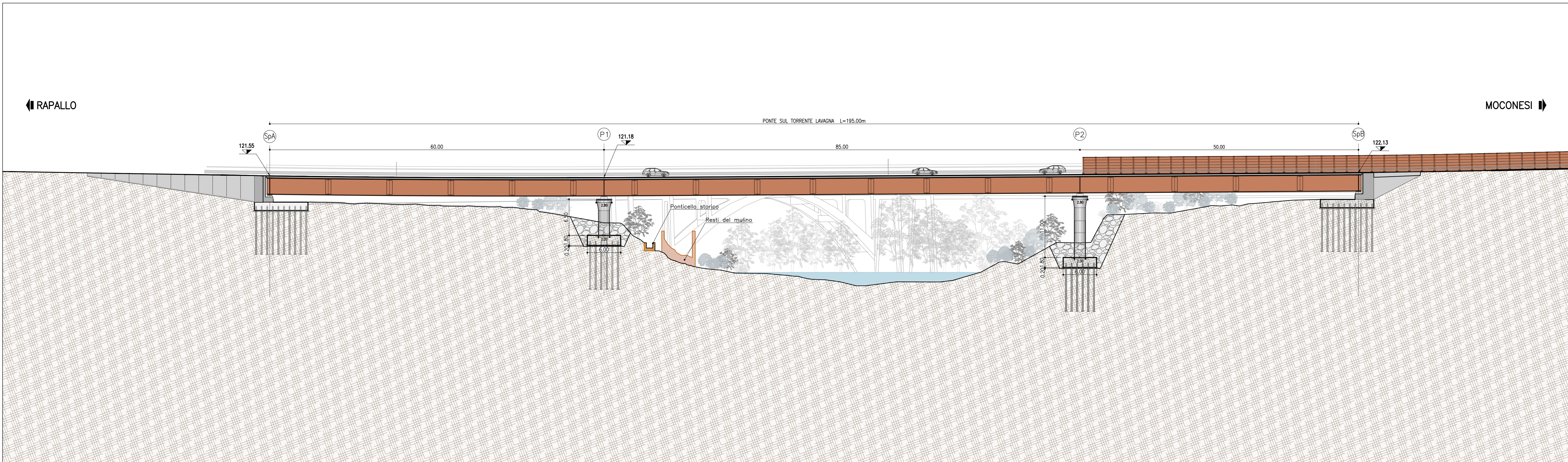
Prospetto A-A' (lato sud) - Scala 1:300
