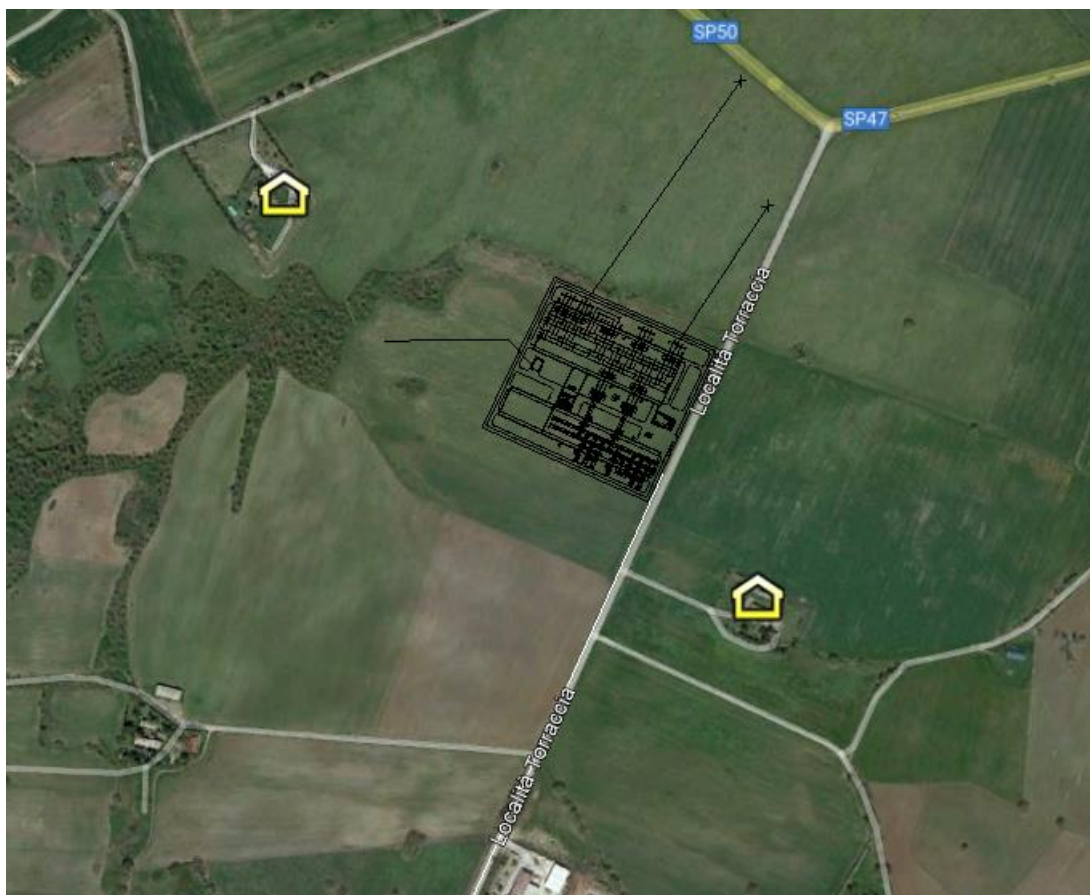
Figura 2 - Sottostazione
