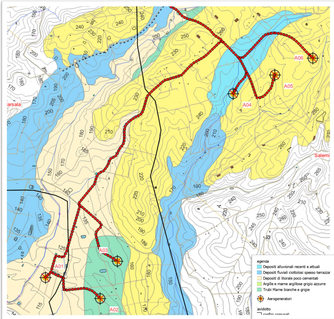
Figura 25 - Stralcio della Carta Geologica.
