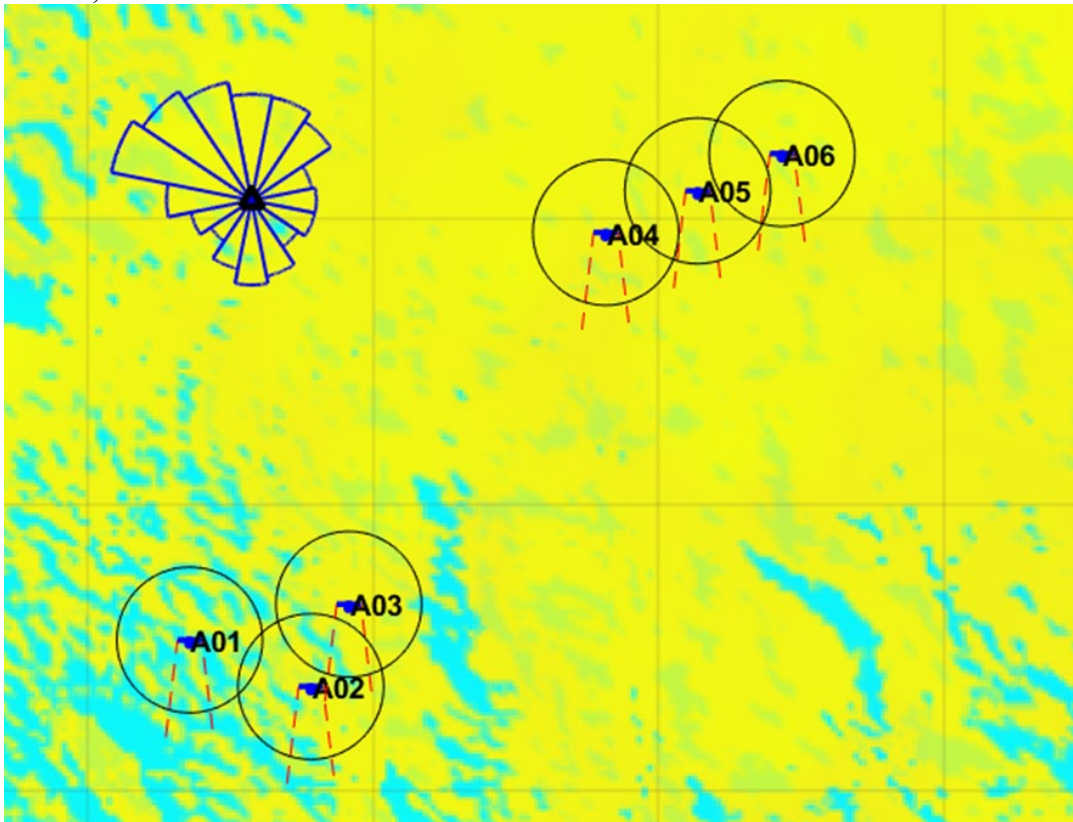
Figura 43 - Rugosità del sito del progetto CE PARTANNA II
