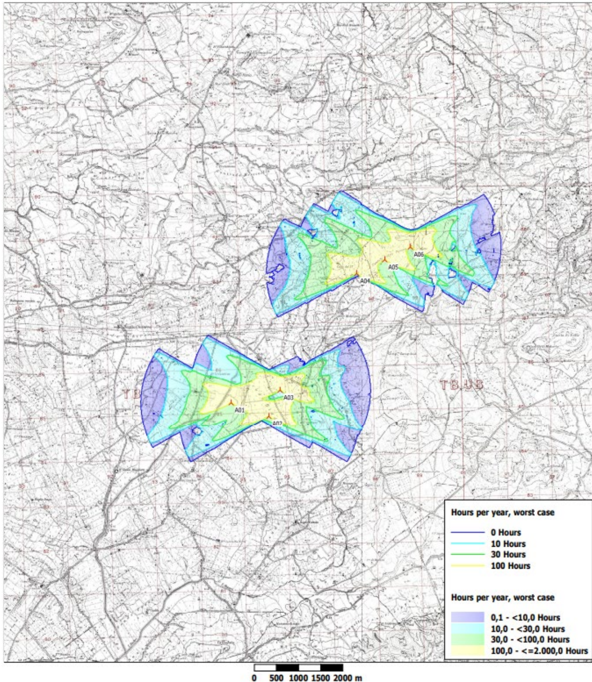
Figura 40 - Rappresentazione grafica dell'ombreggiamento delle turbine rispetto i ricettori
