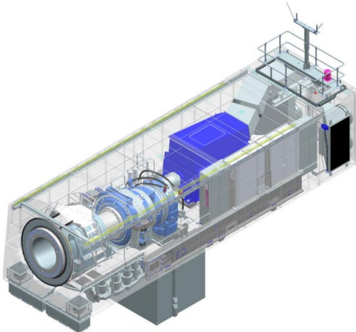
Figura 27 - Disposizione della navicella
