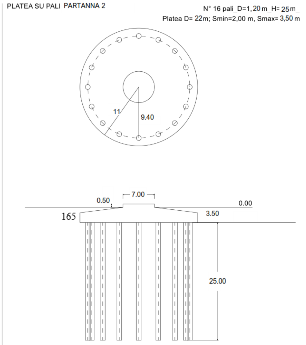
Figura 38 - Dettagli misure platea su pali.
