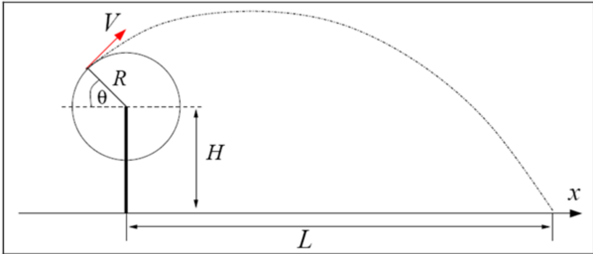
Figura 39 - Schema grafico di gittata
