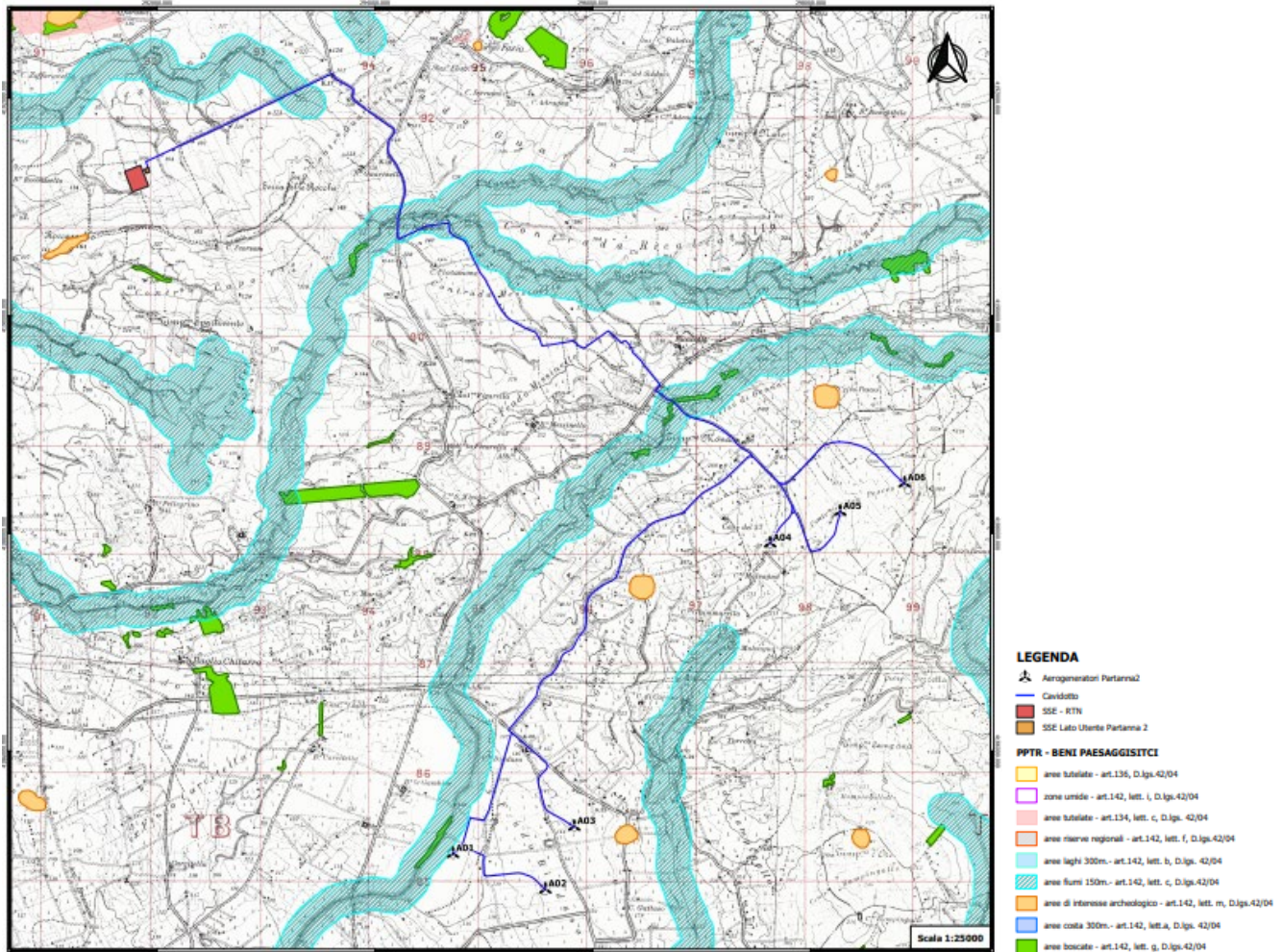
Figura 14 - Estratto elaborato grafico “Beni Paesaggistici – Piano Paesaggistico Prov.TP”
