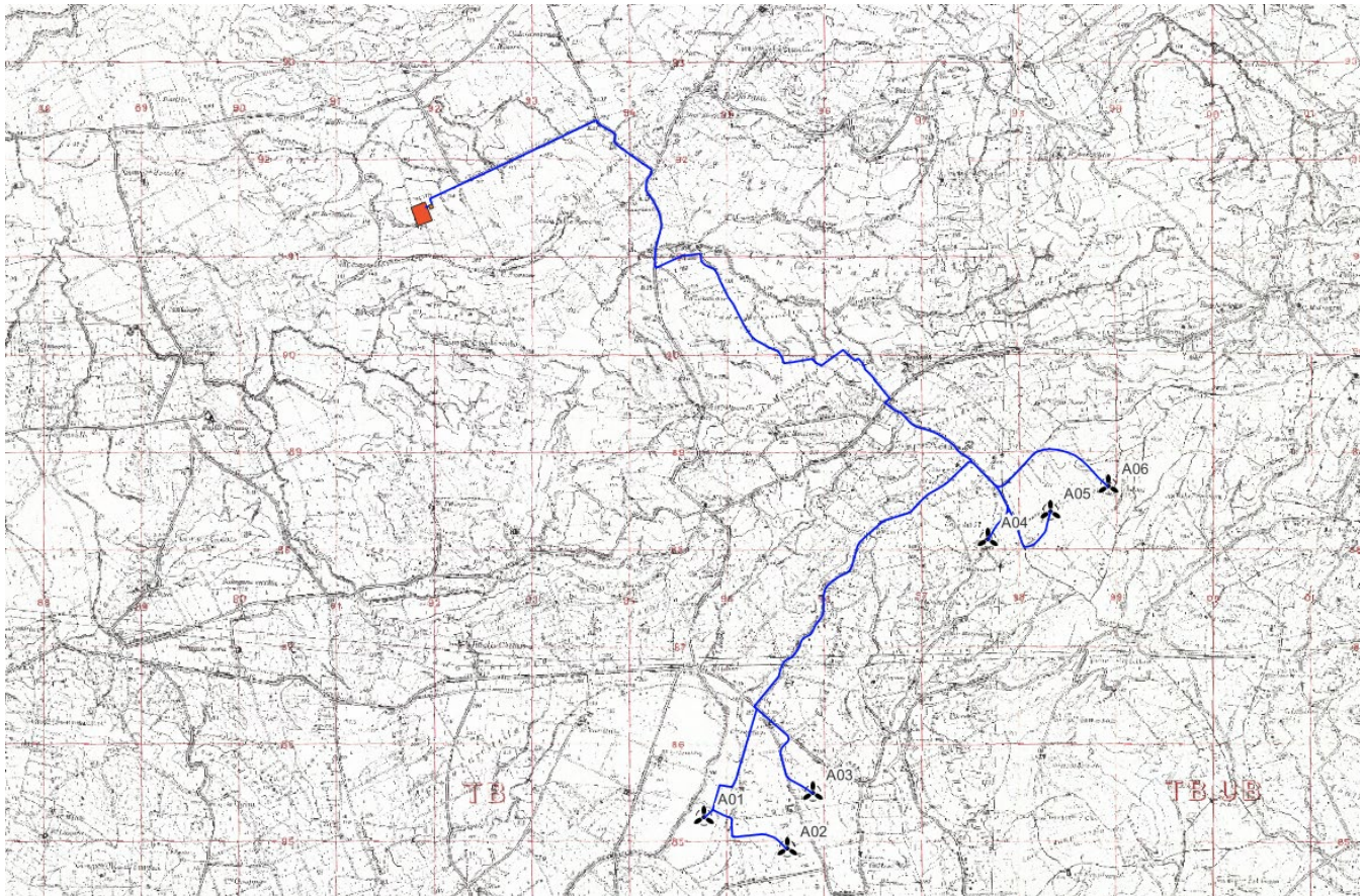
Figura 18 - Inquadramento area campo e sottostazione su IGM
