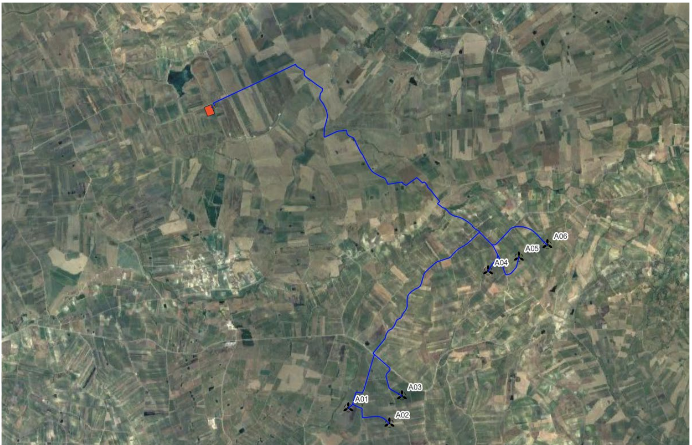
Figura 15 - Inquadramento area campo fotovoltaico su base ortofoto
