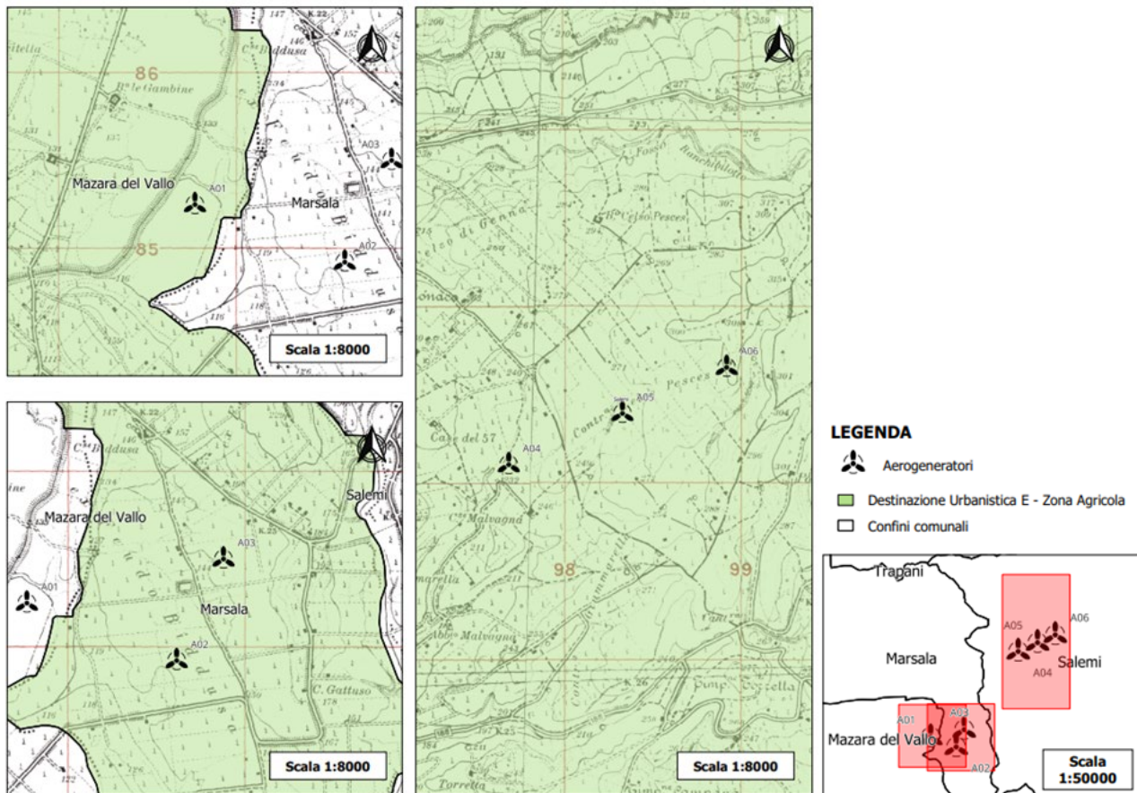
Figura 12 - Estratto PRG Comuni di Salemi, Mazara del Vallo e Marsala
