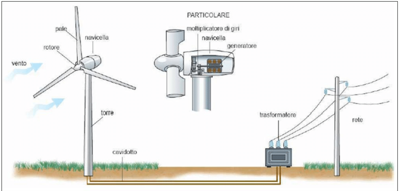
Figura 1 - Schematizzazione impianto eolico
