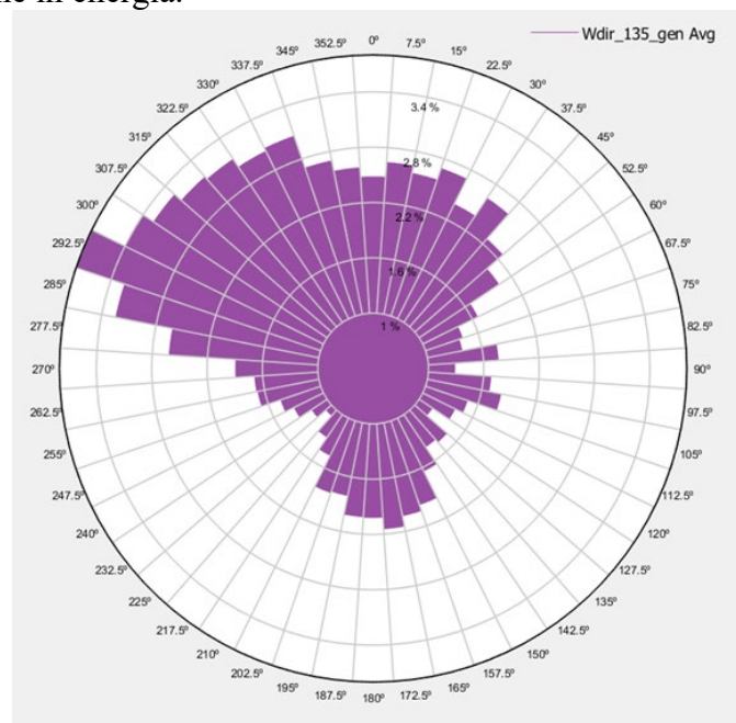
Figura 42 - Rosa dei venti del progetto CE PARTANNA II
