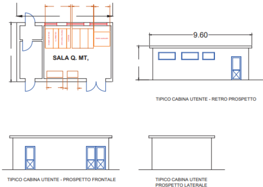
Figura 21 – Particolare SSE Lato Utente Partanna 2
