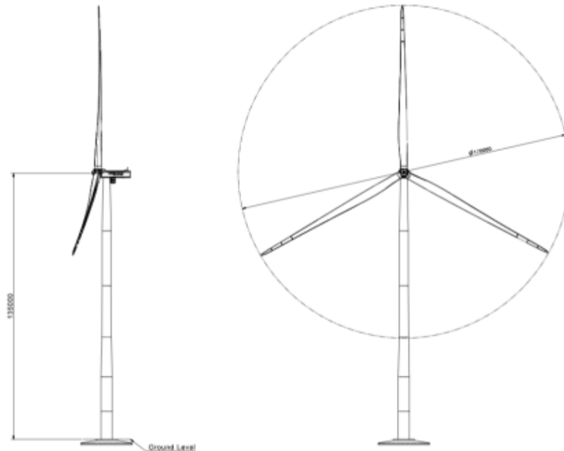
Figura 8 - SG 6.6-170 135 m
