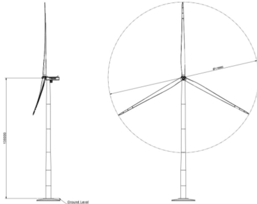
Figura 8 - SG 6.6-170 135 m
