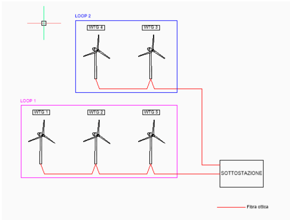
Figura 1 - Schema fibra ottica
