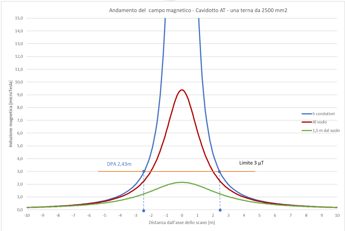
Figura 4 - Andamento del campo magnetico in funzione della distanza dall'asse dei conduttori in forma grafica relativa al cavidotto AT
