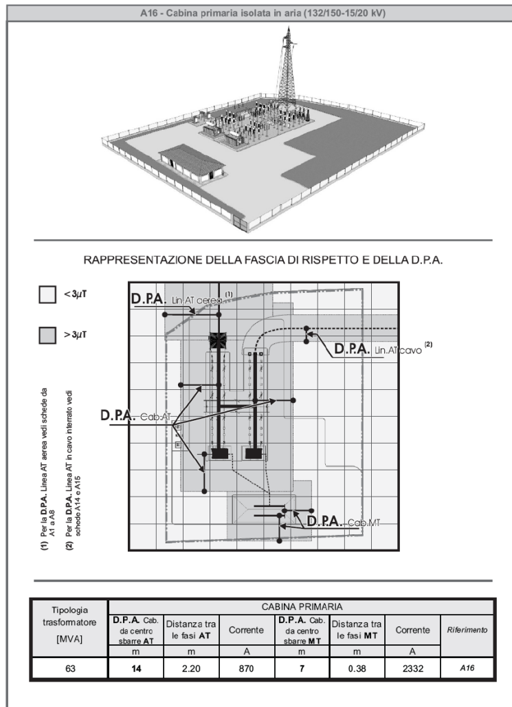
Figura 3 - Esempio di fasce di rispetto relative ad una cabina primaria
