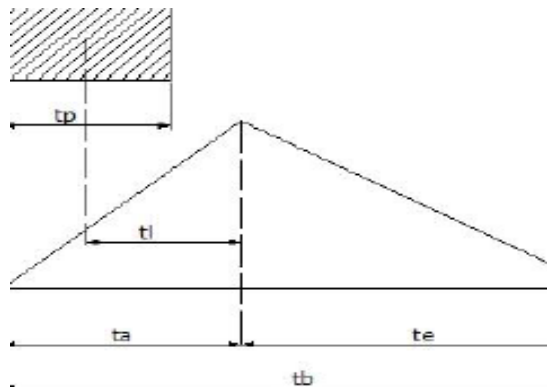
Figura 10 - Idrogramma di Mockus
