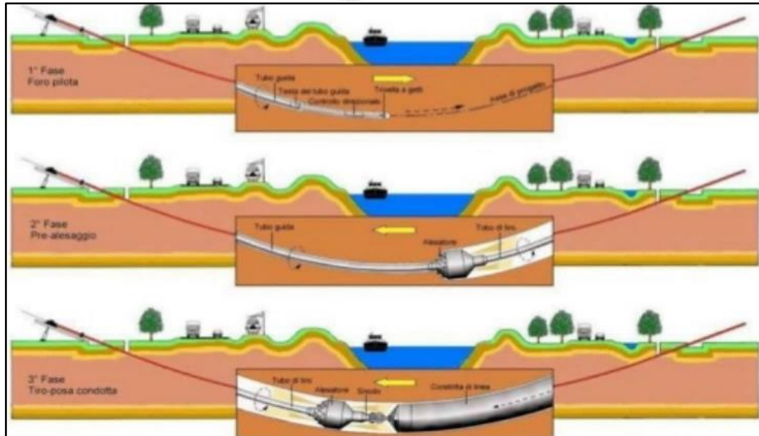
Figura 5 – Fasi di realizzazione della T.O.C.
