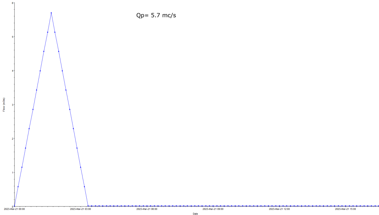
Figura 4 – Idrogramma di piena in input – Bacino 1
