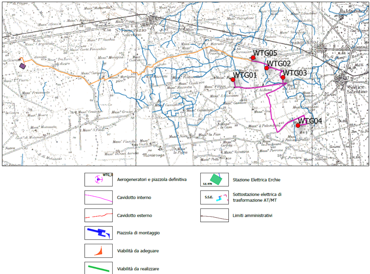
Figura 11 – Intersezioni tra il cavidotto e i reticoli idrografici
