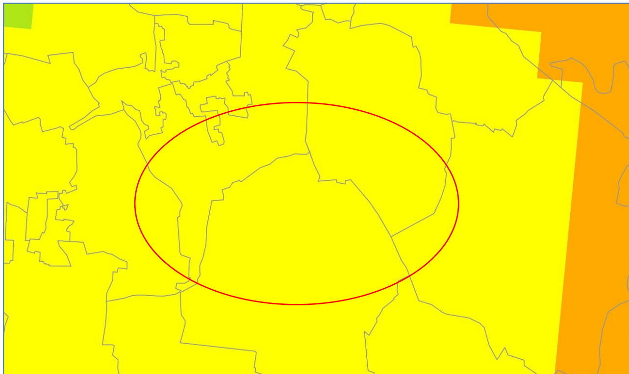
Figura 3 - velocità del vento a 100 m s.l.t.
