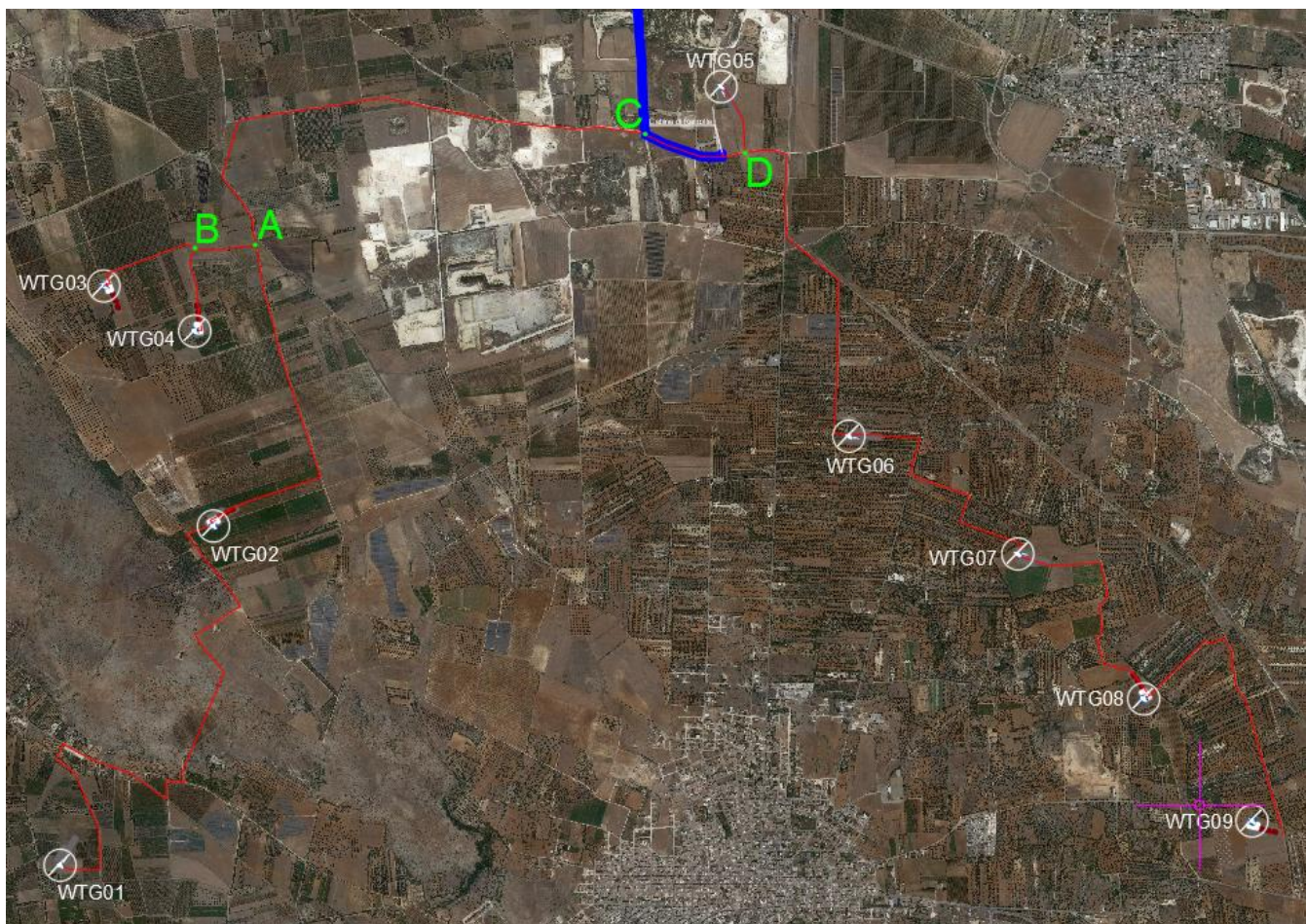
Figura 3 - Inquadramento su ortofoto del layout impianto
