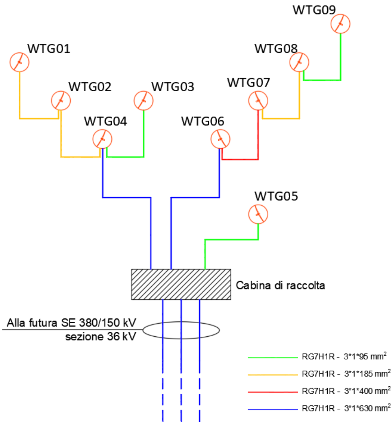
Figura 4 - Schema di connessione elettrica dell'impianto eolico in progetto
