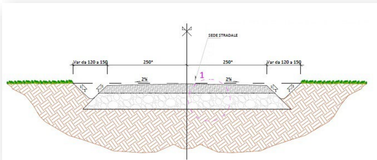
Figura 21 – sezione stradale tipo
