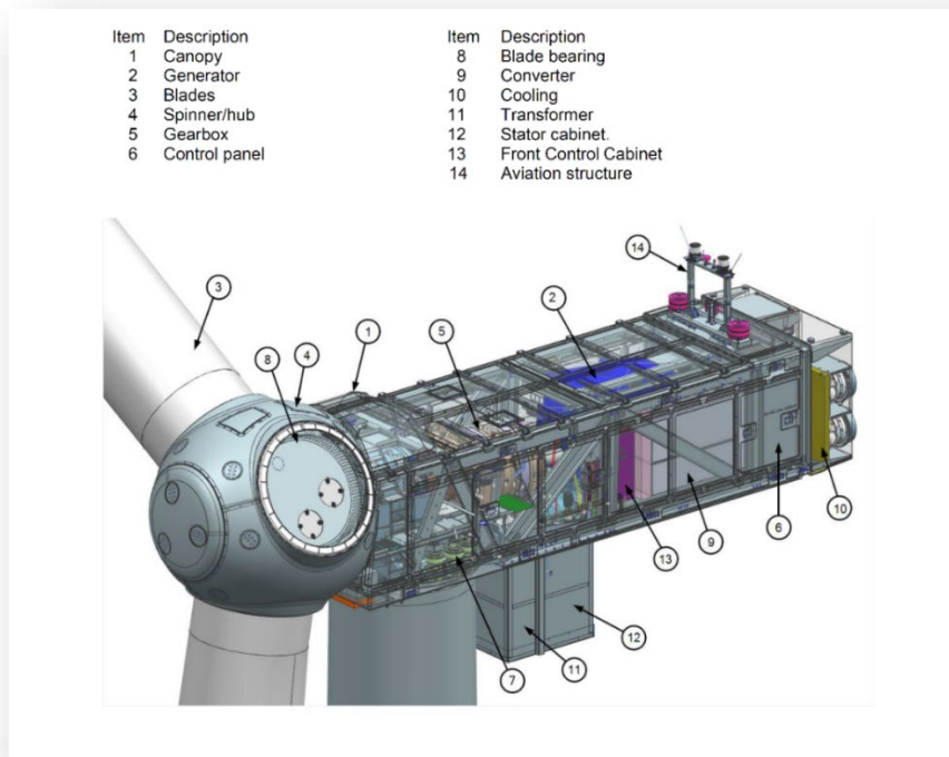
Figura 15 - Schema rappresentativo della navicella
