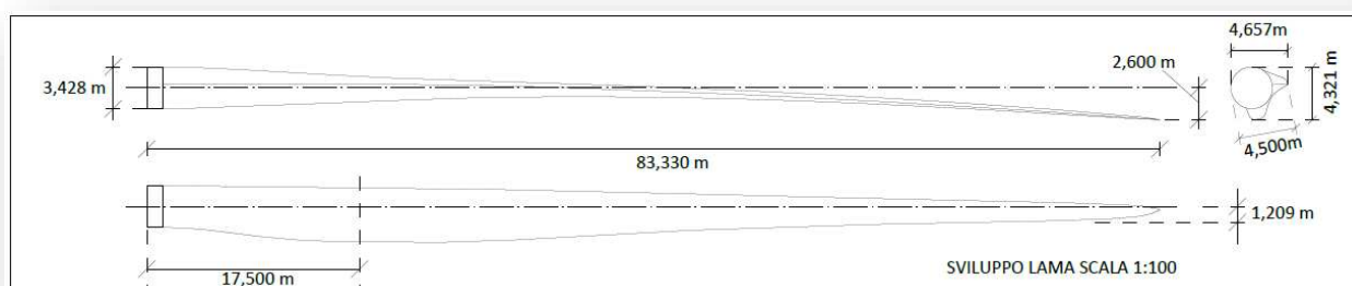
Figura 17 - Estratto elaborato Sezione tipo aerogeneratore
