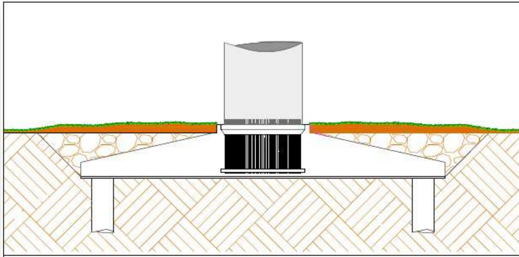
Figura 18 - Schema rappresentativo della fondazione tipo
