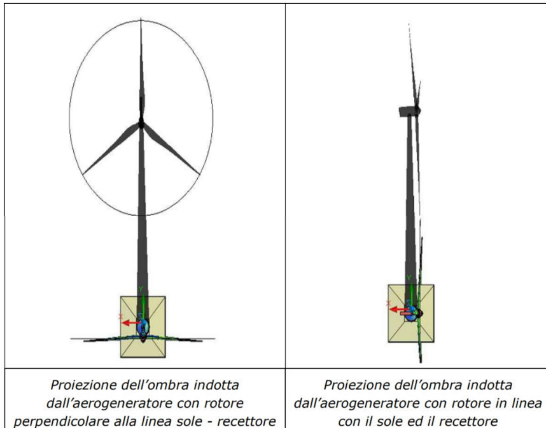
Figura 2 Rappresentazione della proiezione dell'ombra con rotore rispettivamente perpendicolare ed allineato con la direzione sole-recettore
