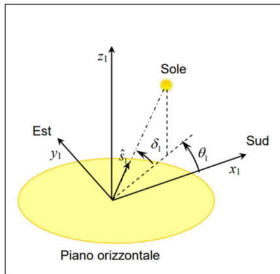
Figura 4 Coordinate solari locali
