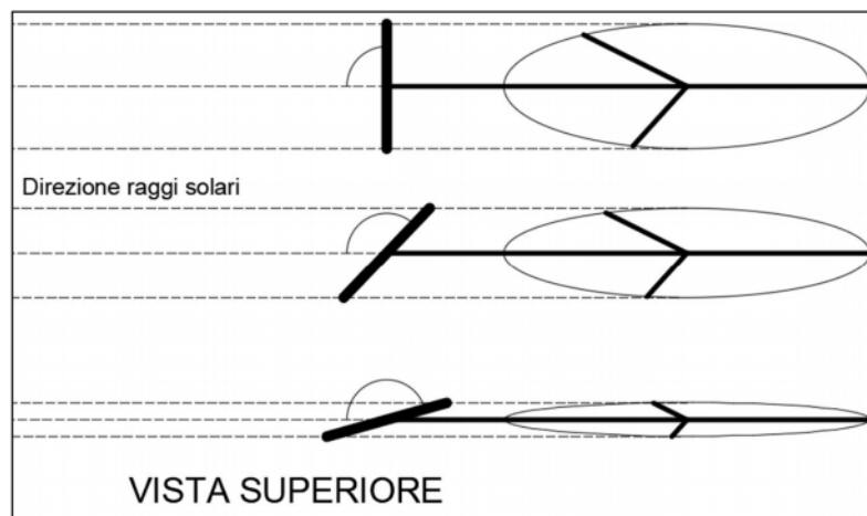
Figura 8 Effetto dell'angolo tra la direzione dei raggi solari ed il rotore sull'ampiezza dello shadow flickering
