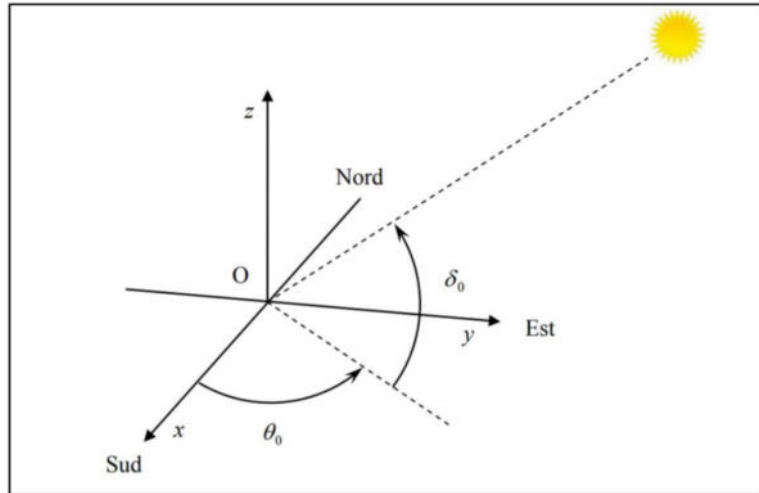
Figura 3 Coordinate solari astronomiche
