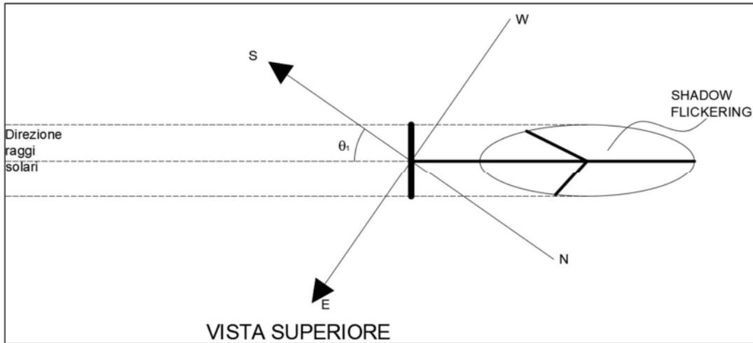
Figura 6 Vista superiore del fenomeno di shadow flickering
