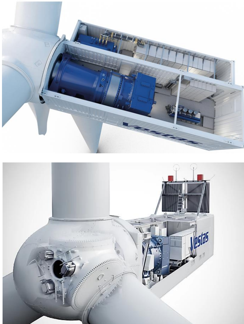
Figura 1 schema descrittivo della navicella WTG
