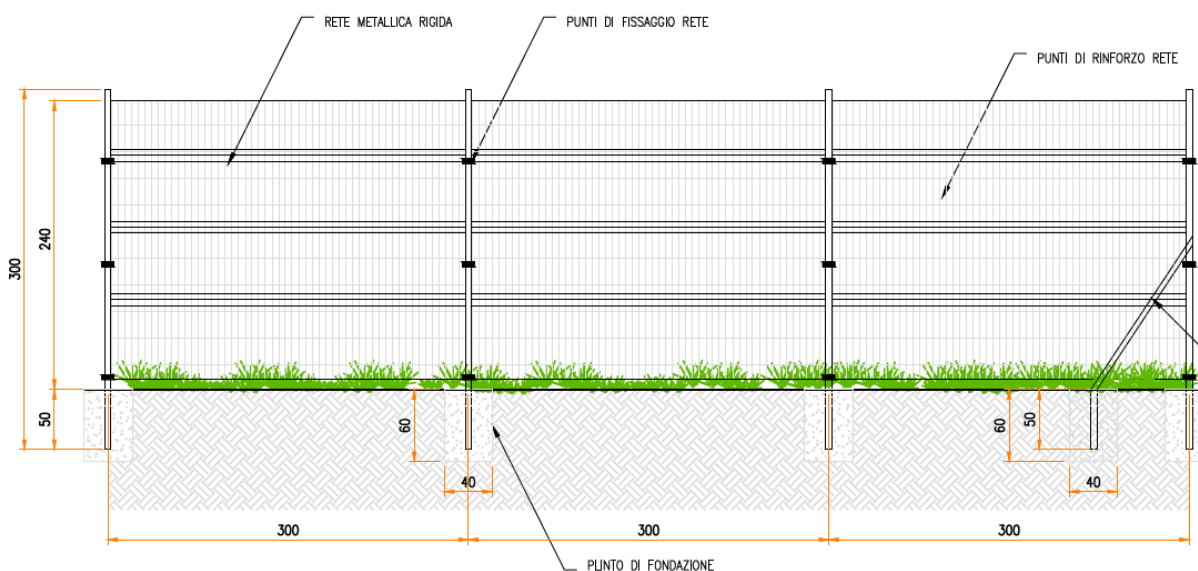
Figura 4.5: Tipico recinzione
