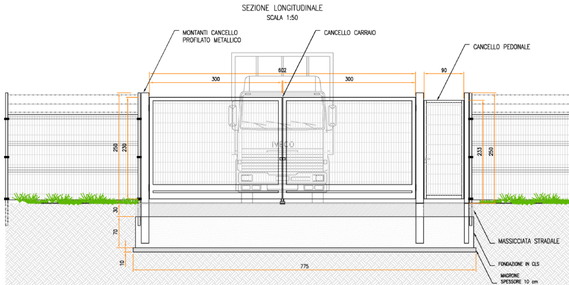
Figura 4.6: Tipo cancello
