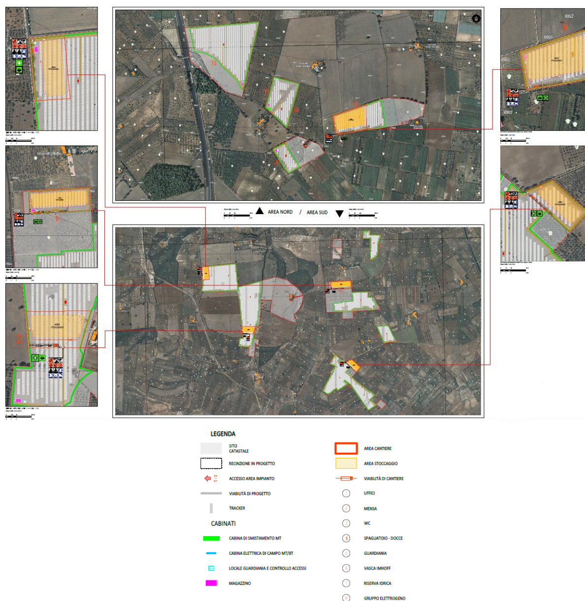
Figura 4.1: Stralcio della planimetria area cantiere
