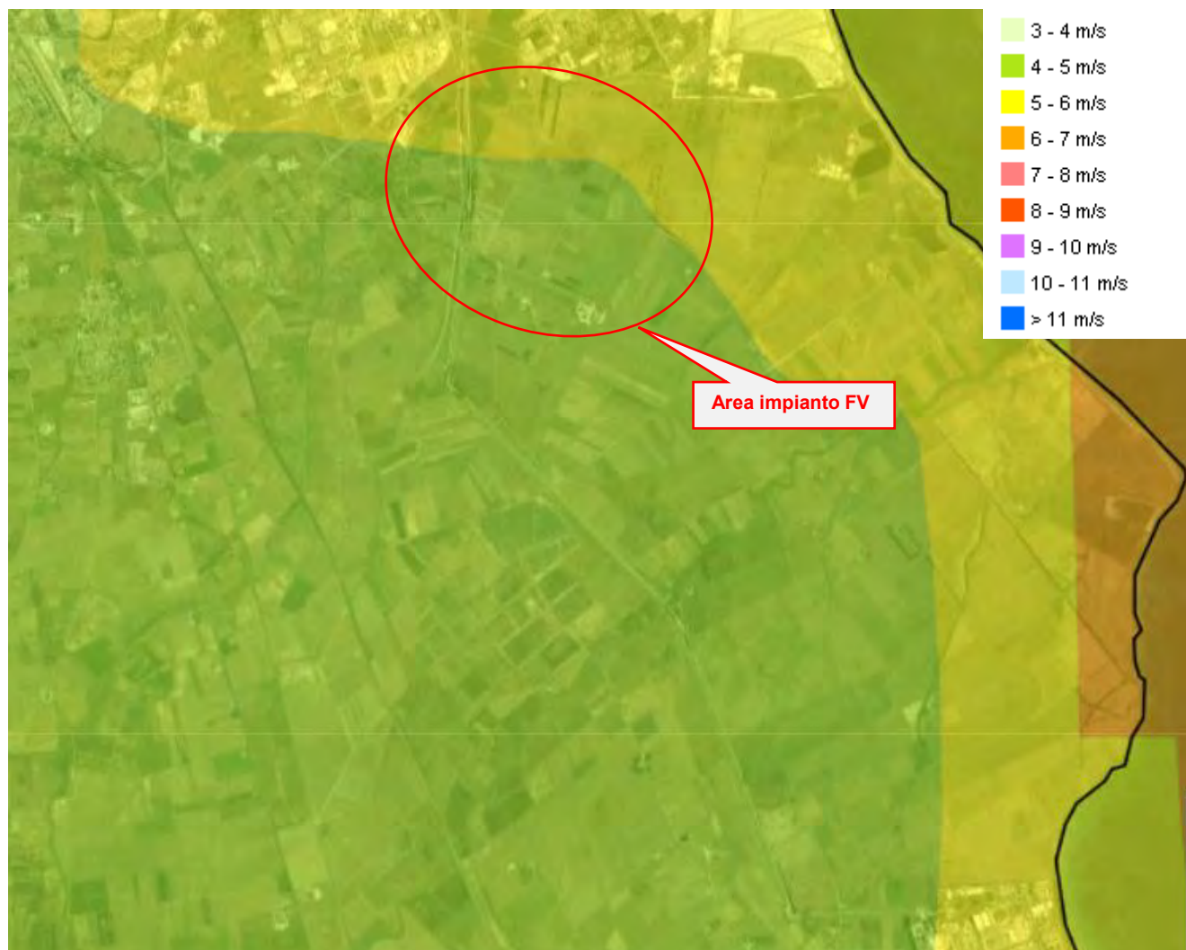
Figura 4-7: velocità del vento nel territorio di Brindisi, fonte http://atlanteoelico.rse-web.it/
