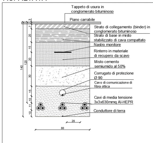
Figura 3-2 Sezioni tipo di posa del Cavidotto interrato
