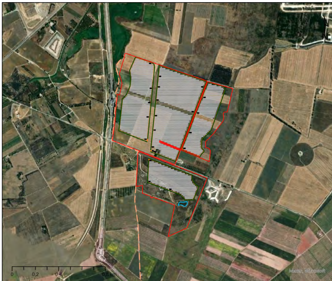
Figura 11: Ortofoto con vista dell'impianto fotovoltaico
