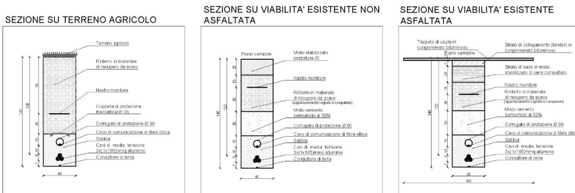
Sezione tipo scavo trincea cavidotto MT (1 terza)
