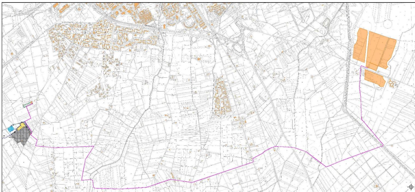
Inquadramento generale percorso cavidotti interni ed esterni
