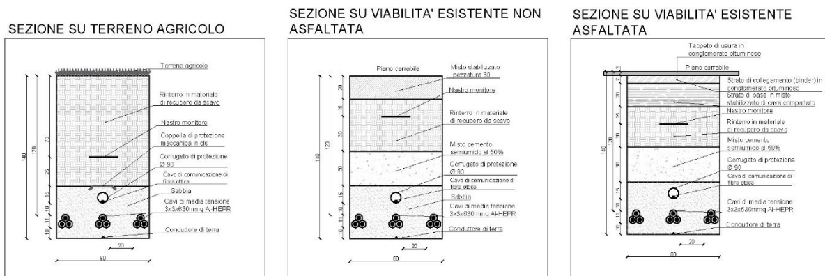
Sezione tipo scavo trincea cavidotto MT (2 terna)
