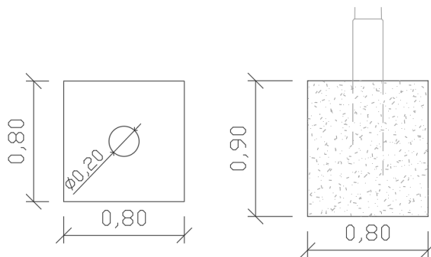
Figura 1 - Particolare costruttivo dello scavo dei pali di illuminazione e videosorveglianza
