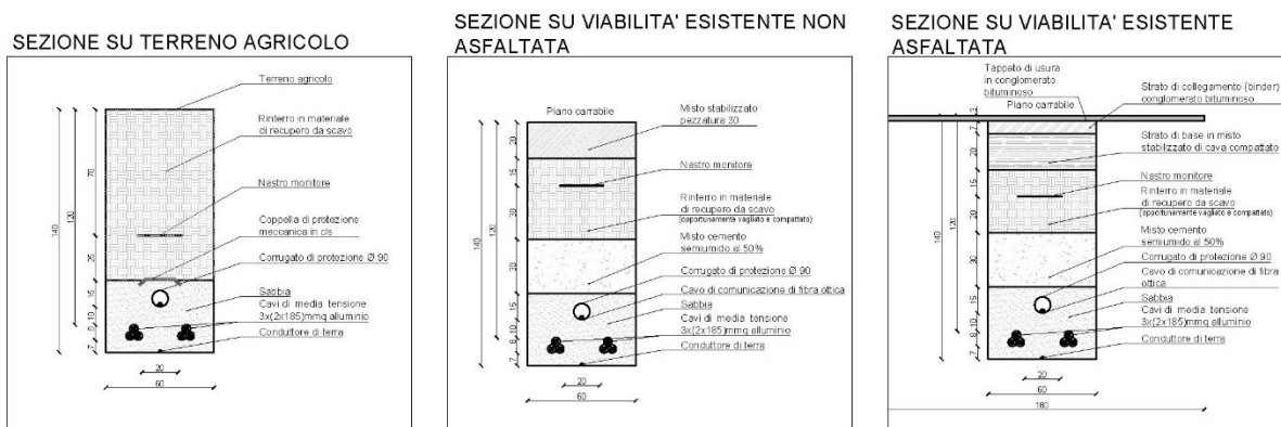
Sezione tipo scavo trincea cavidotto MT (2 terza)
