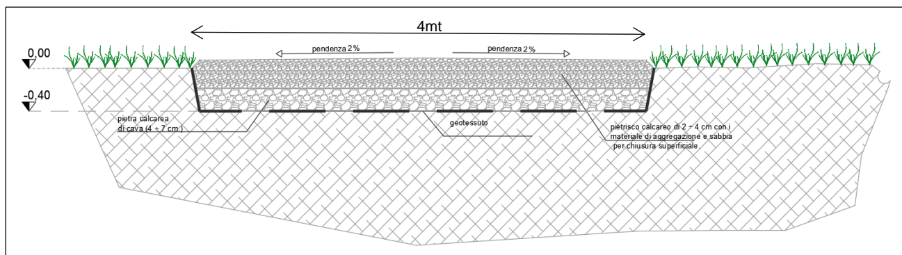
Sezione tipo viabilità interna
