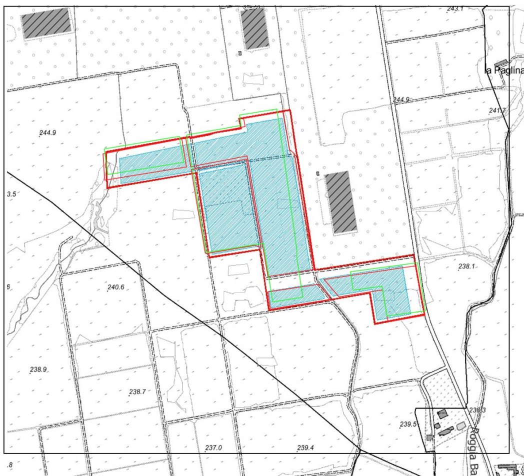
Figura 4: Inquadramento di dettaglio su C.T.R. (immagine fuori scala); in rosso sono individuate le aree in proprietà e l'area recintata nel layout originale, in verde l'area recintata nel nuovo layout, in azzurro le aree in cui si prevede la realizzazione dell'impianto fotovoltaico nel layout originale.
