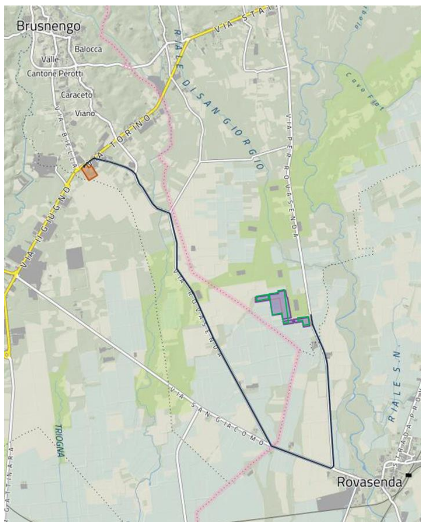
Figura 2: Inquadramento delle opere in progetto; in viola la recinzione dell'impianto fotovoltaico nel layout originale e in verde la recinzione nuovo layout in nero la linea di connessione interrata e in rosso la stazione elettrica (fonte: www.geoportale.piemonte.it ).
