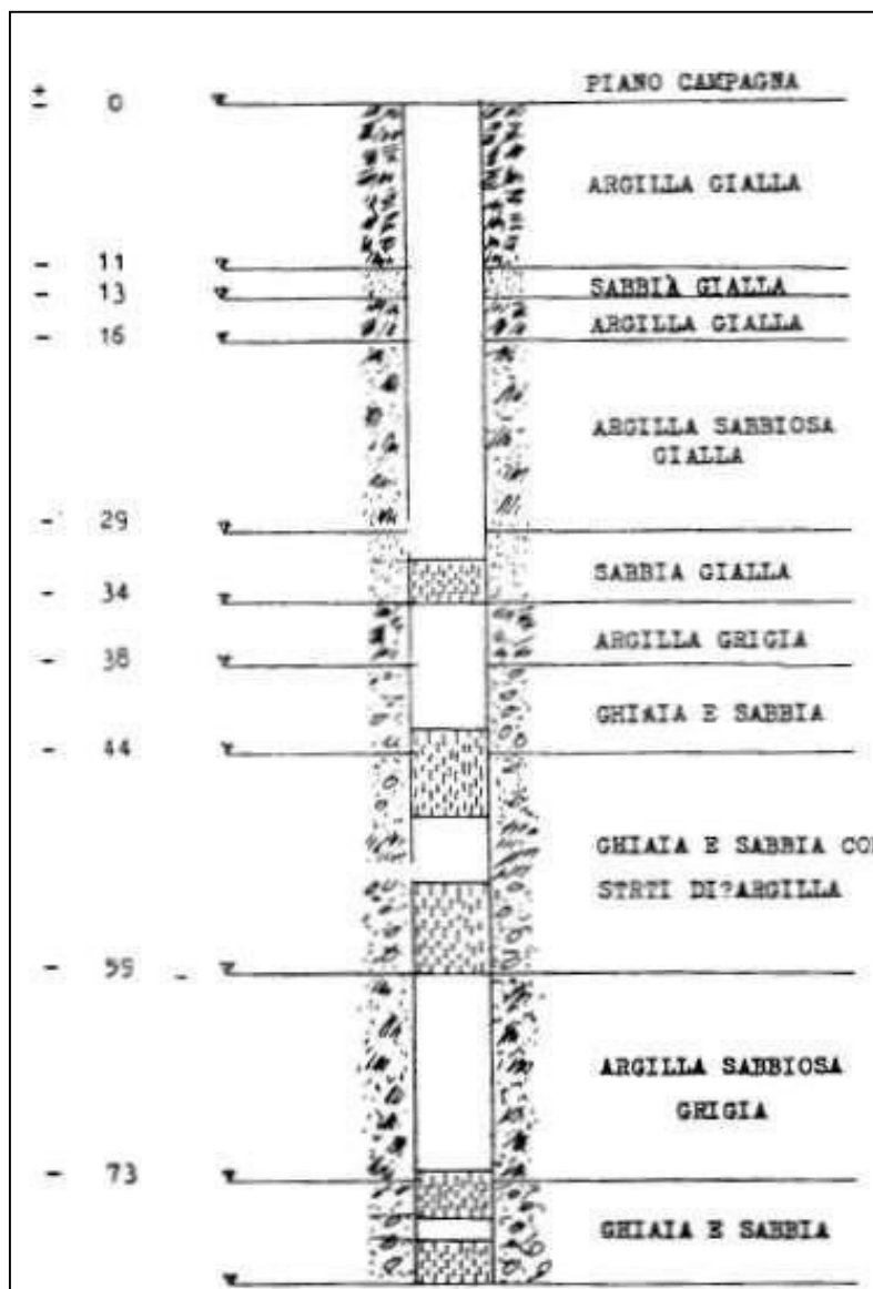
Figura 29: Profilo stratigrafico di un pozzo idrico presente nei pressi dell'area
