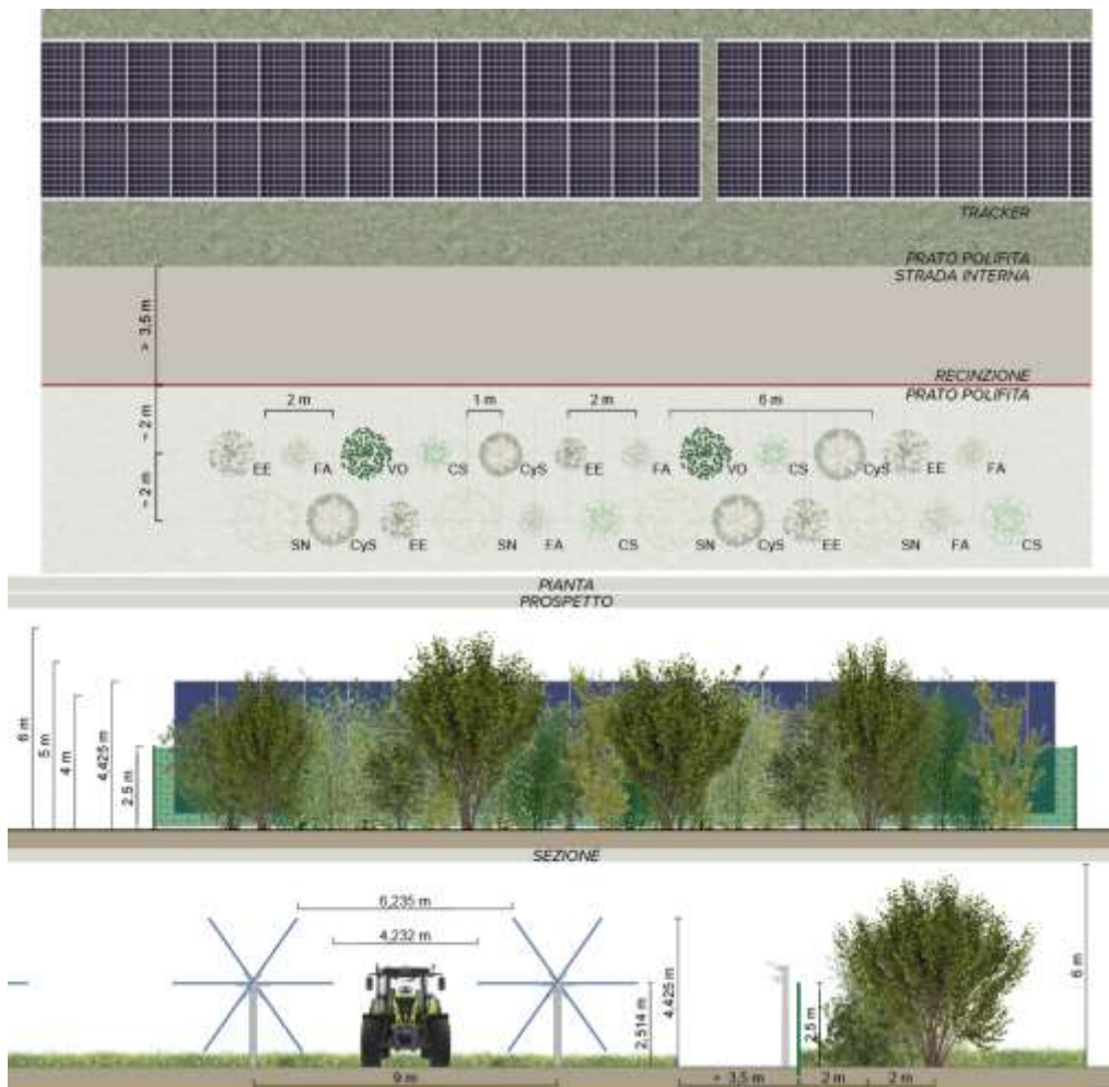
Figura 25 Sesto di impianto, prospetto e sezione delle fasce vegetate “Tipo 4”
