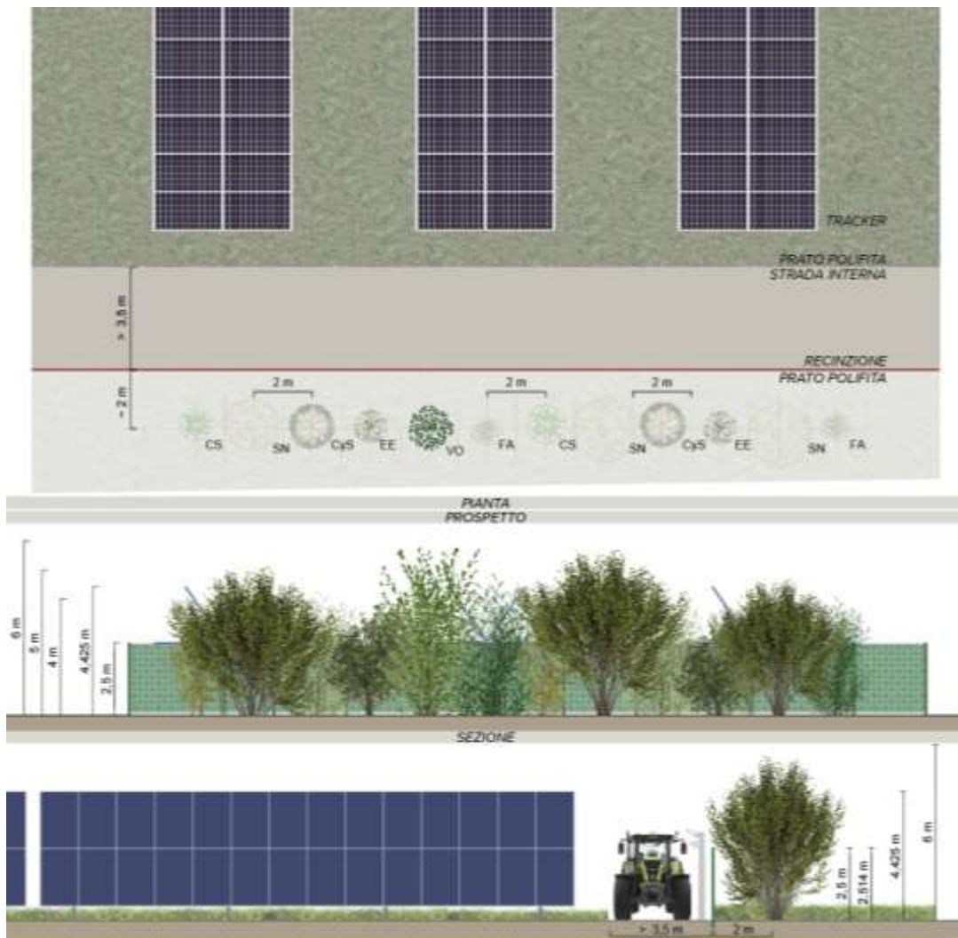
Figura 27 Sesto di impianto, prospetto e sezione delle fasce vegetate "Tipo 5"
