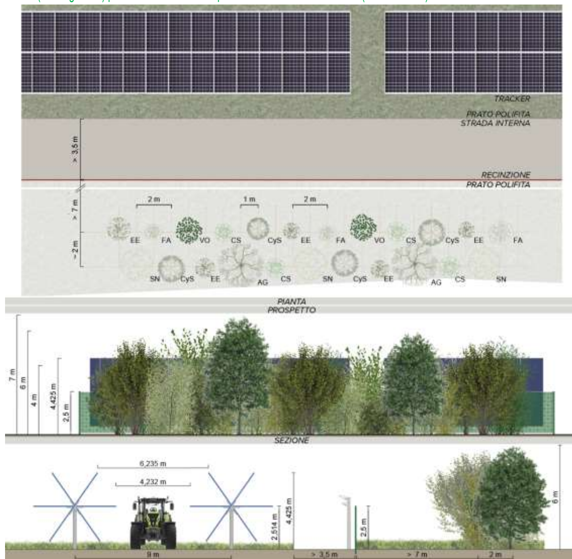
Figura 19 Sesto di impianto, prospetto e sezione delle fasce vegetate "Tipo 1"
