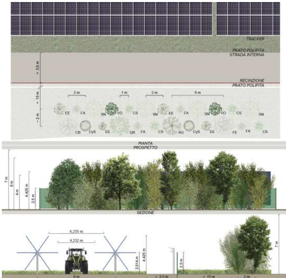
Figura 23 Sesto di impianto, prospetto e sezione delle fasce vegetate "Tipo 3"
