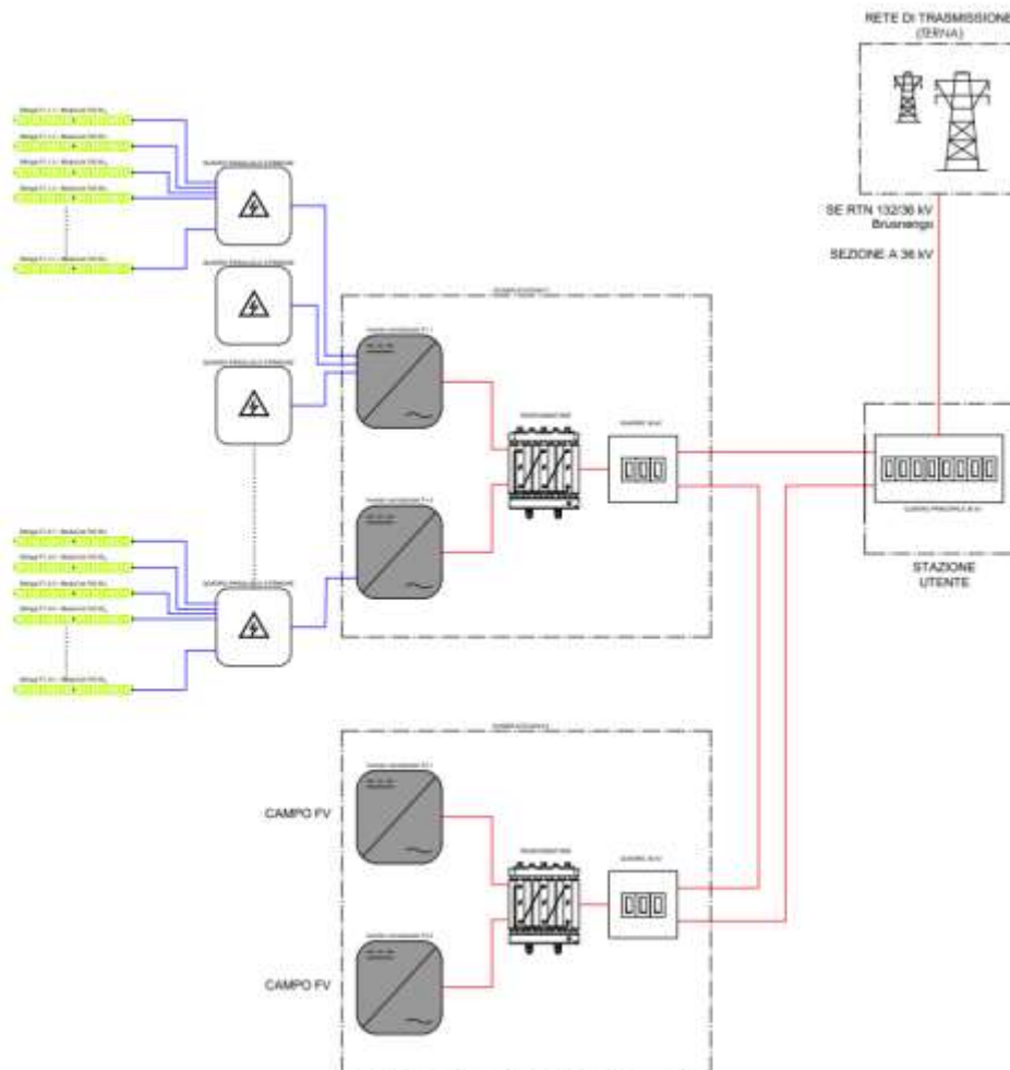
Figura 6 Schema a blocchi dell'impianto
