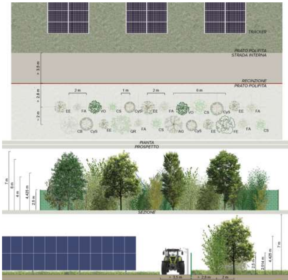
Figura 21 Sesto di impianto, prospetto e sezione delle fasce vegetate "Tipo 2"
