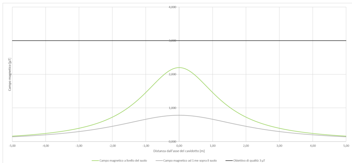
Figura 3: Campo magnetico a livello del suolo con indicazione dell'obiettivo di qualità
