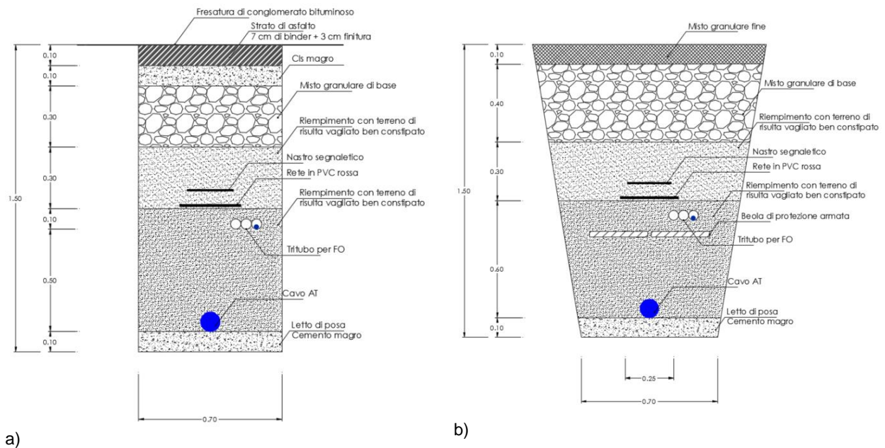
Figura 2: Modalità di posa cavidotto a 36 kV su strada asfaltata (a) o strada in terra battuta (b)
