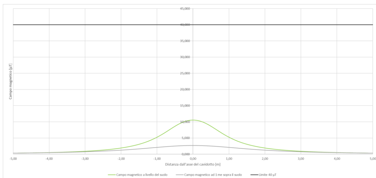
Figura 1: Campo di induzione magnetica generato da 400 A DC su 3 linee interrate a 80 cm
