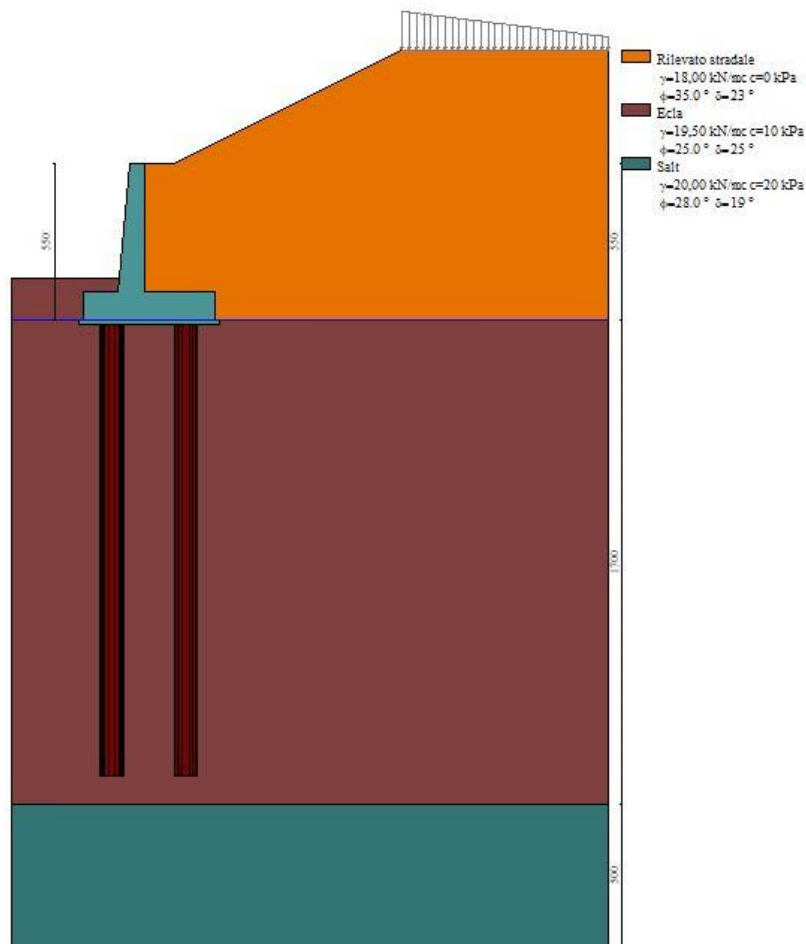
Modello di calcolo muro su PALI
