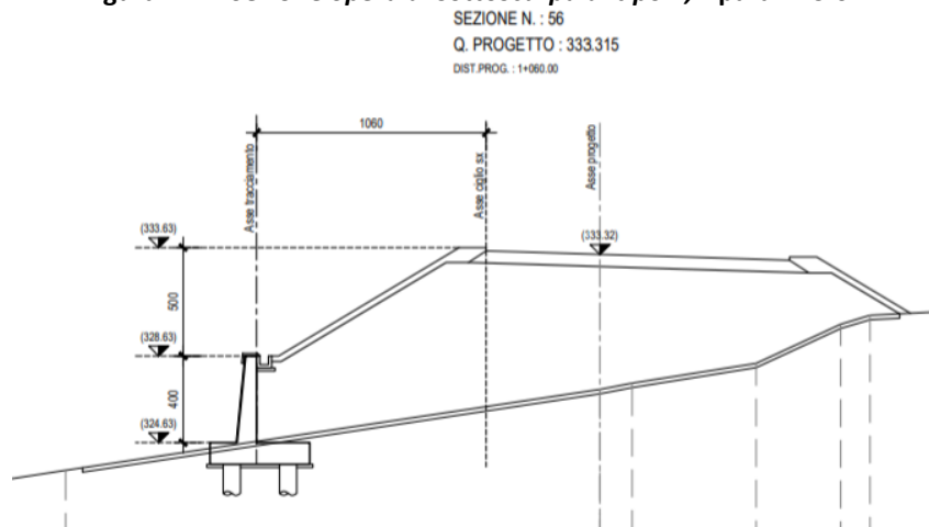
Figura 2.3 – Sezione opera di sottoscarpa di tipo 2, Hparam=4.0 mUNITA' DI MISURA
