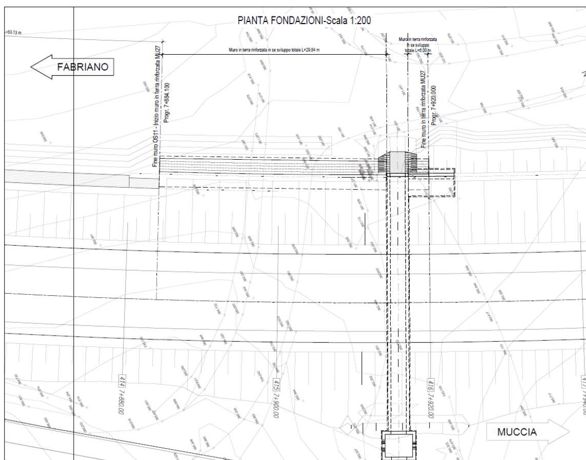
Figura 1 – Pianta dell'opera
