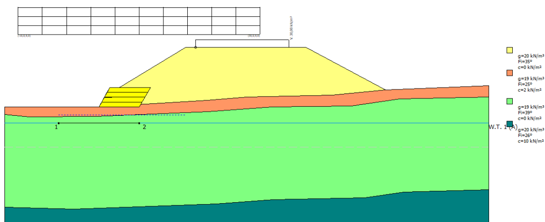
Figura 4 - Modello di calcolo
