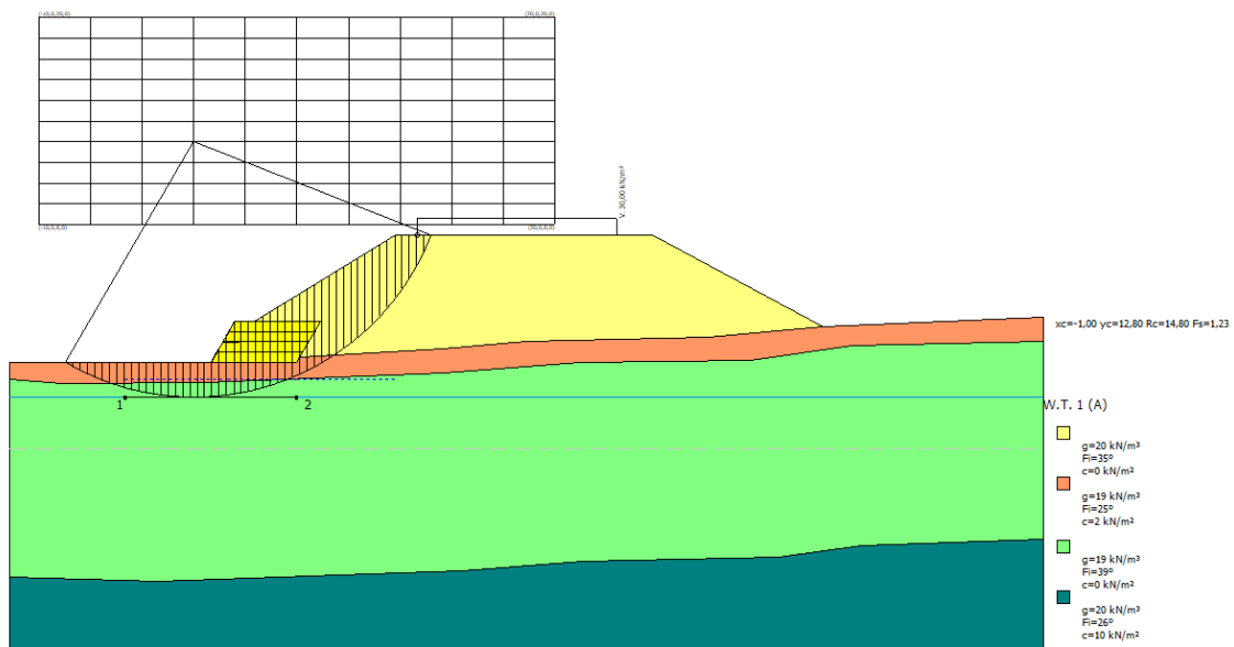
Figura 7 - Risultati analisi di stabilità globale – Condizioni sismiche
