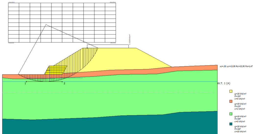
Figura 6 - Risultati analisi di stabilità globale – Condizioni statiche
