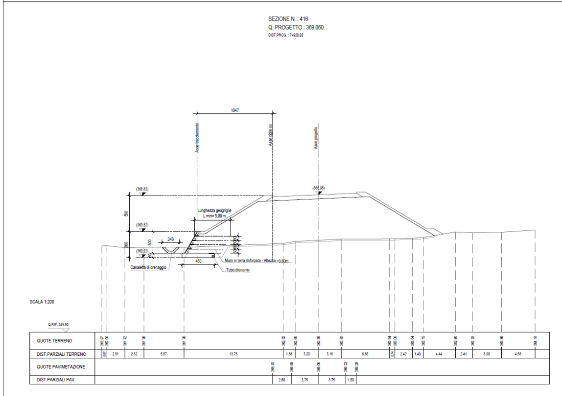
Figura 3 – Sezione generica MU0027
