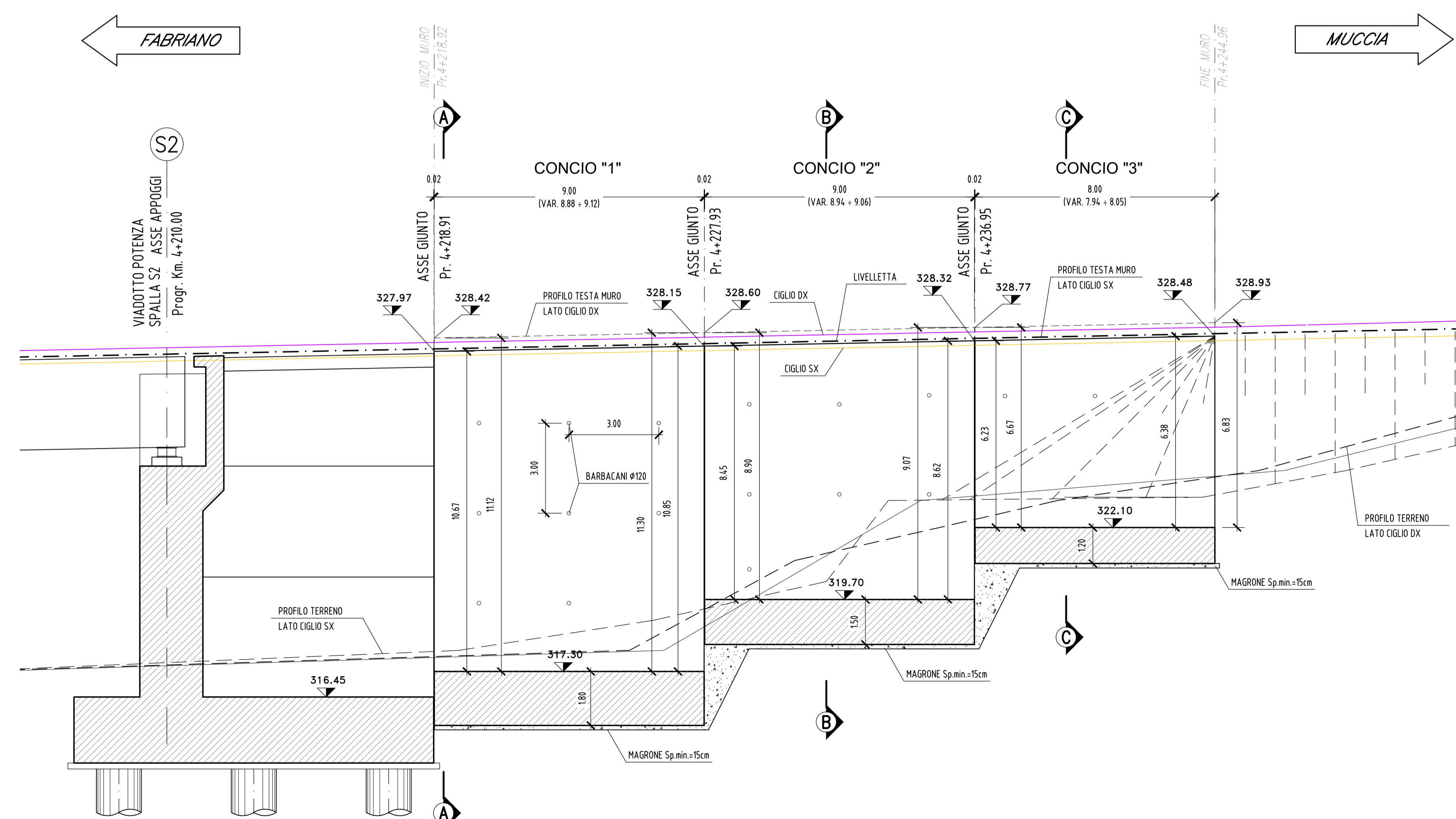
SEZIONE LONGITUDINALE "X-X" IN ASSE TRACCIAMENTO Scala 1:100
