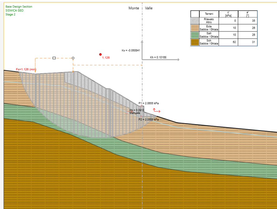
Condizioni Sismiche: Fase definitiva – Superficie Critica di Scorrimento massima H=3.00 m
