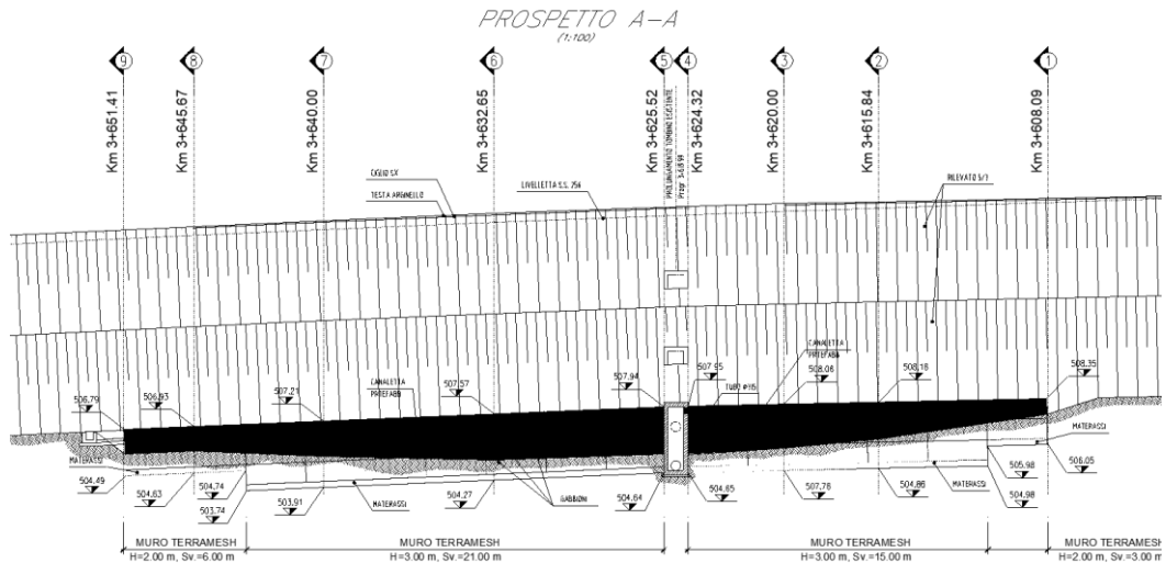
Profilo muro
