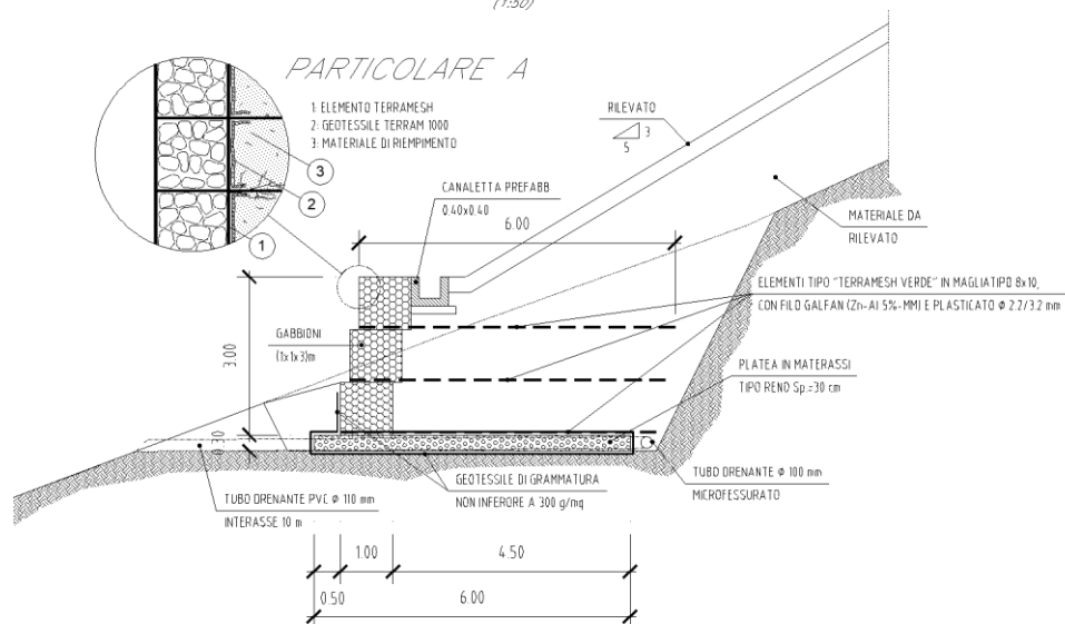
Sezione muro in terramesh System: H = 3.00 m
