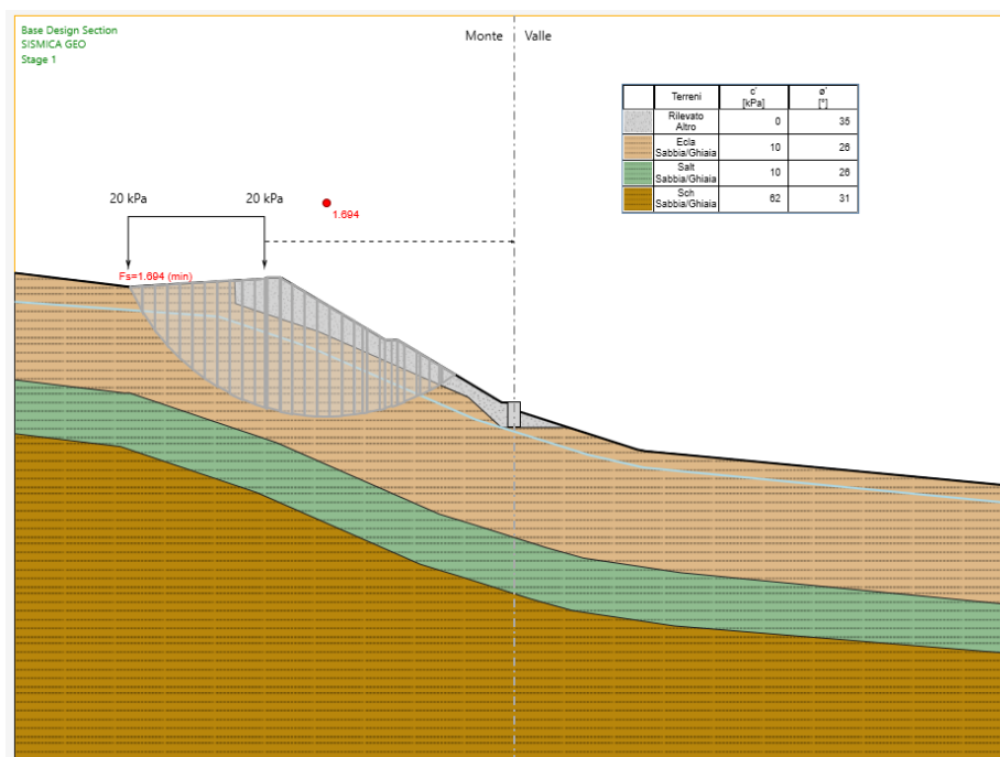
Condizioni Statiche: Fase di esercizio – Superficie Critica di Scorrimento massima muro H=2.00 m
