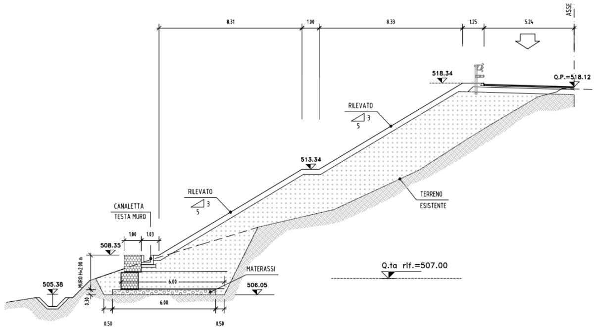
Sezione muro in terramesh System: H = 2.00 m
