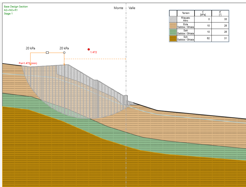
Condizioni Statiche: Fase di esercizio – Superficie Critica di Scorrimento massima muro H=3.00 m
