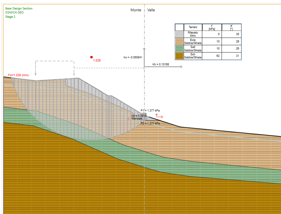
Condizioni Sismiche: Fase definitiva – Superficie Critica di Scorrimento massima H=2.00 m
