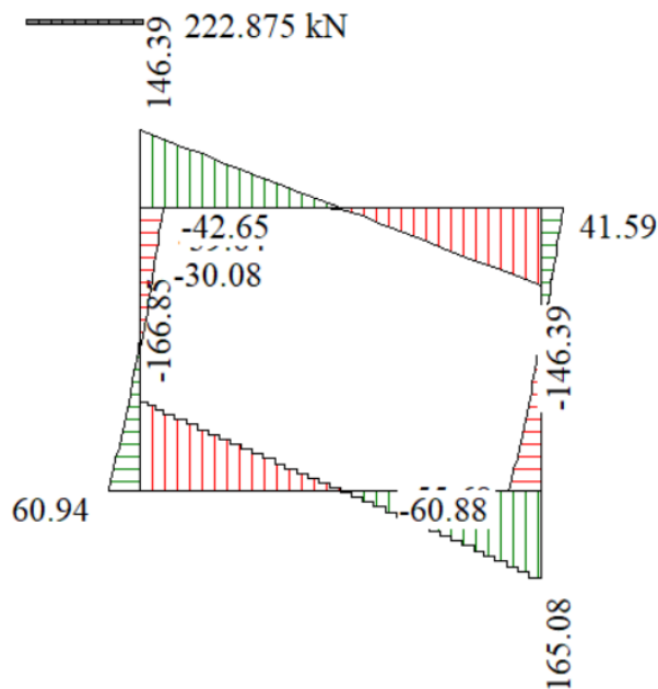
Involuppo diagrammi del taglio– SLE
