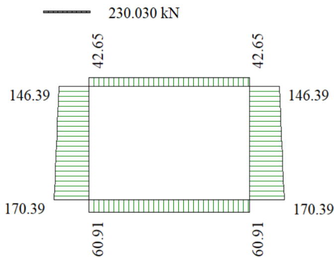
Involuppo diagrammi dello sforzo normale – SLE
