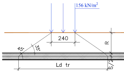
DIFFUSIONE TRASVERSALE CARICHI STRADALI Q1 (Longitudinale all'opera)
