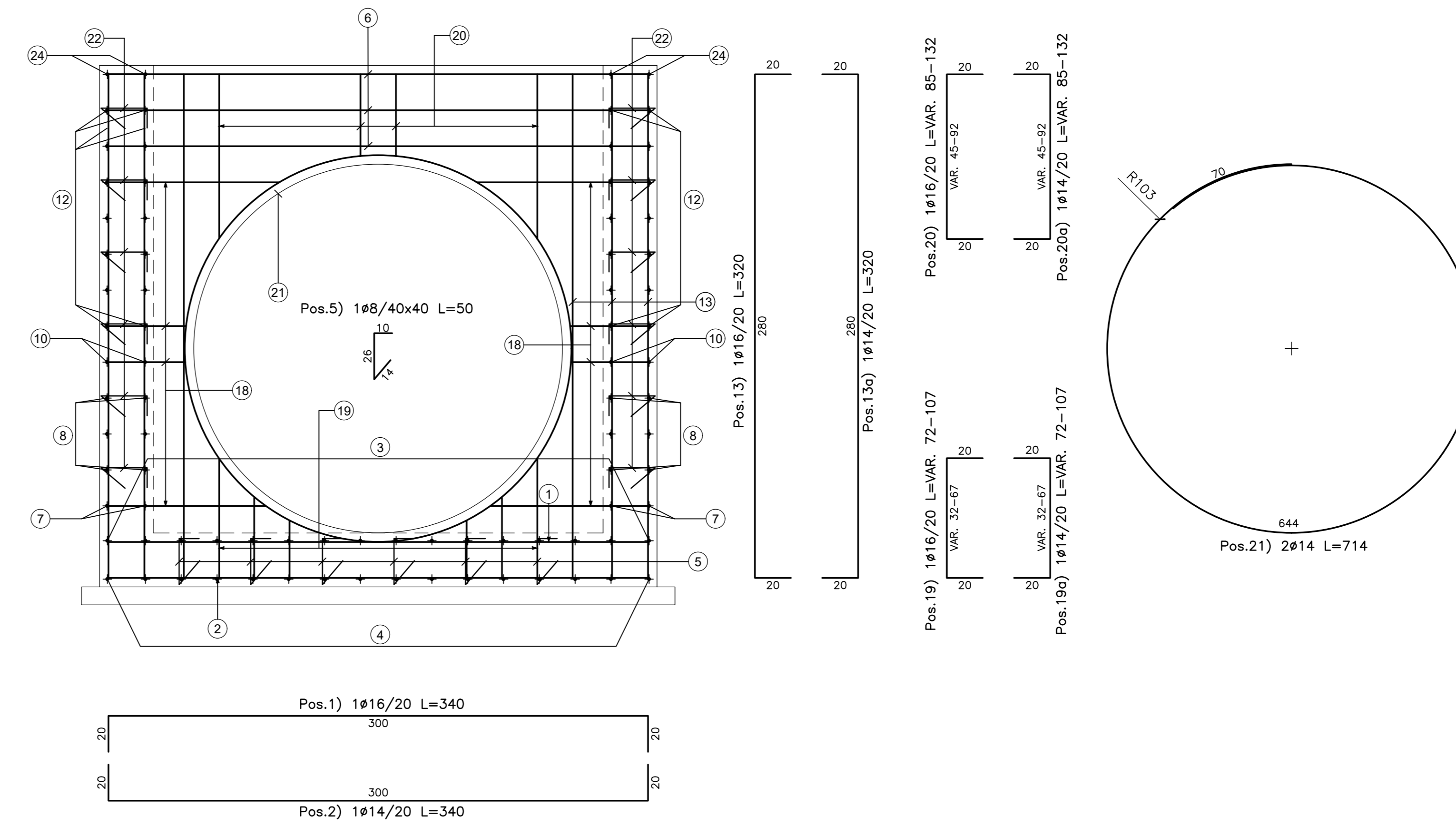
VISTA A-A Scale 1:20
