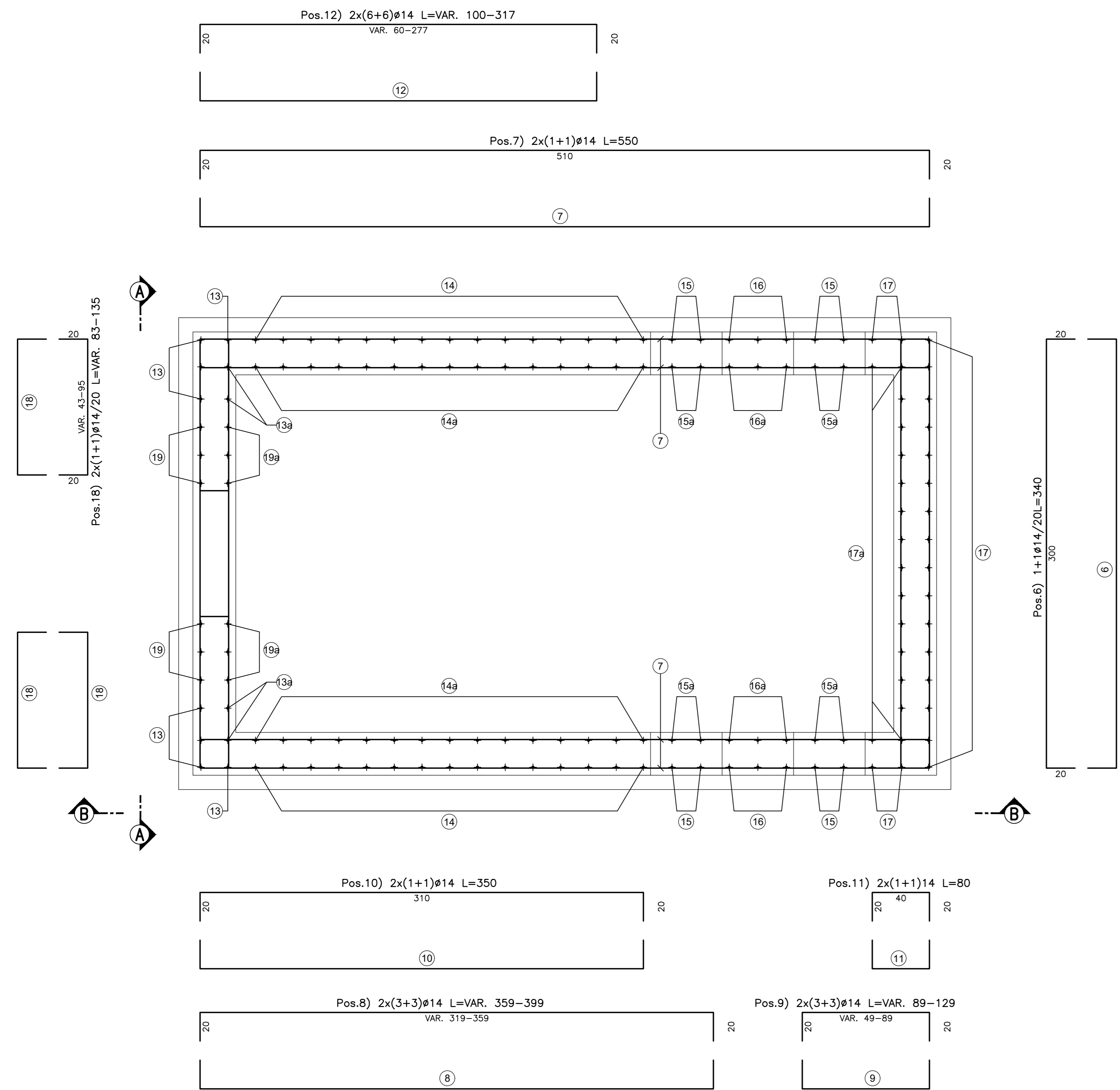
PIANTA SPICCATO Scale 1:20
