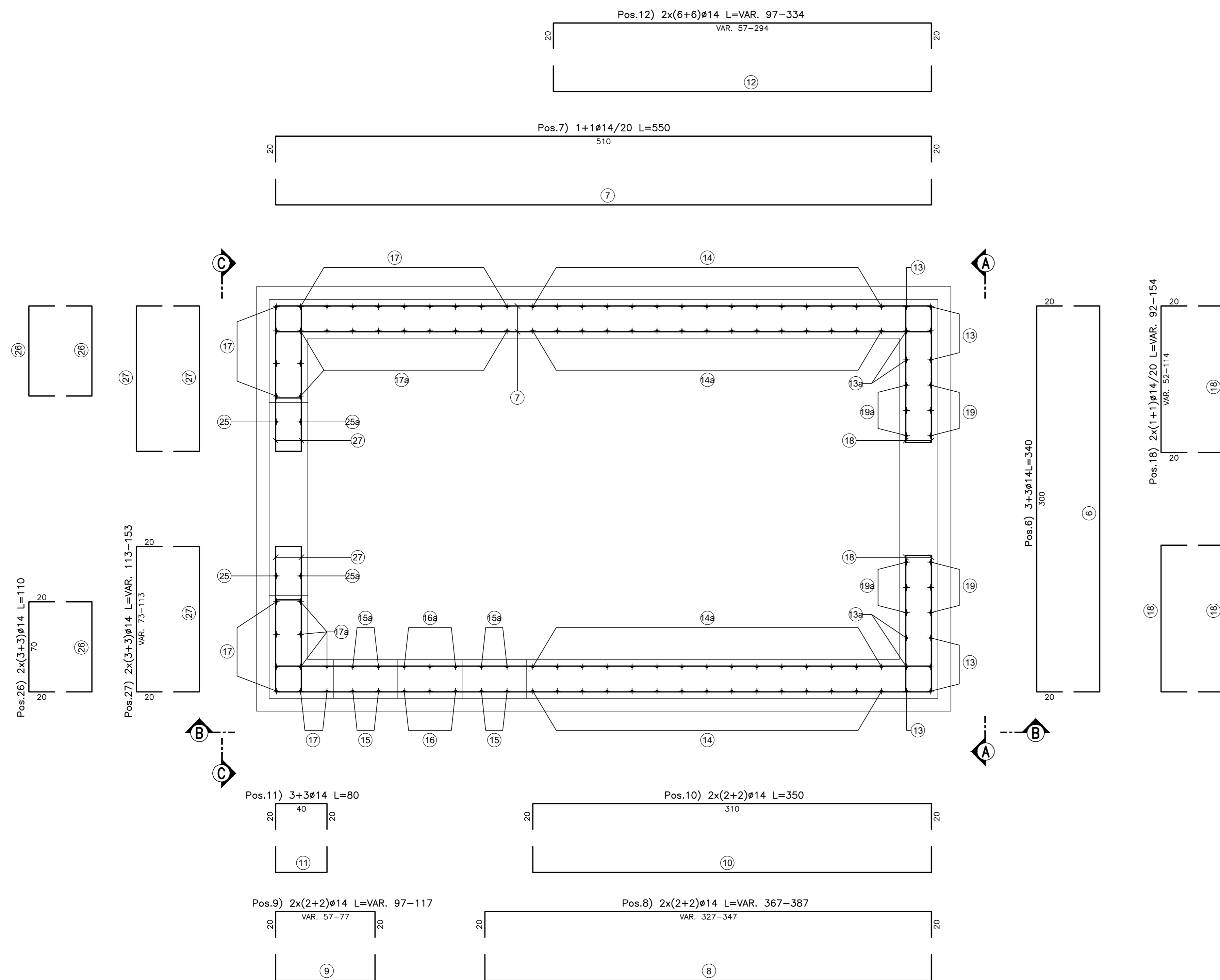
PIANTA SPICCATO Scala 1:20
