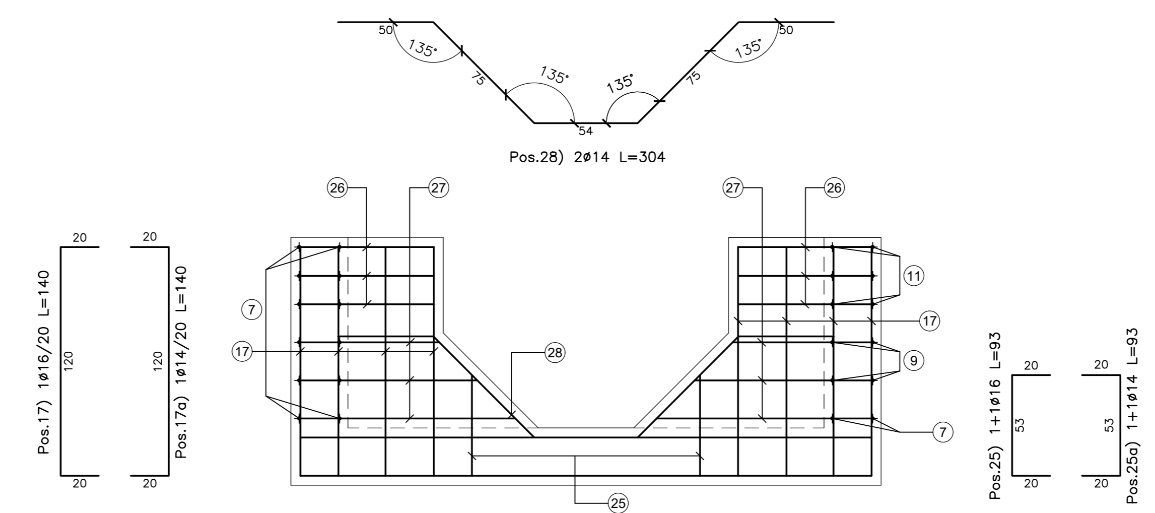
VISTA C-C Scala 1:20
