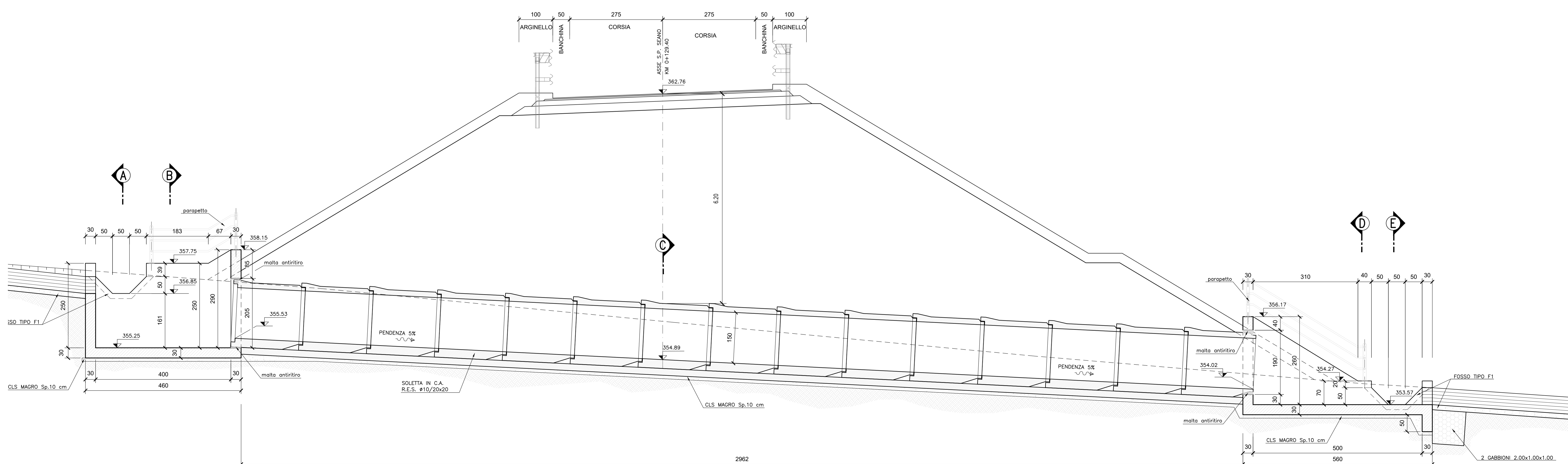
SEZIONE F-F Scala 1:50
