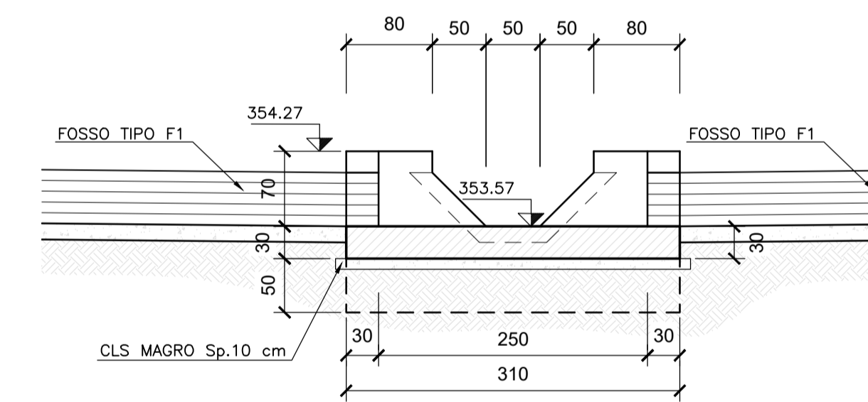
SEZIONE E-E Scala 1:50
