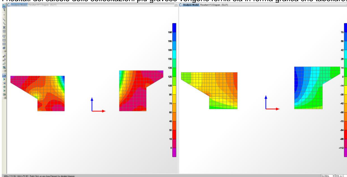
Diagramma dei momenti e dei tagli che tendono le fibre orizzontali – SLU
