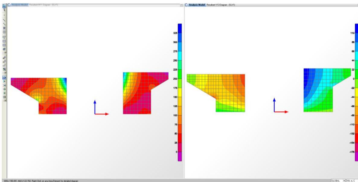
Diagramma dei momenti e dei tagli che tendono le fibre orizzontali – SLV
