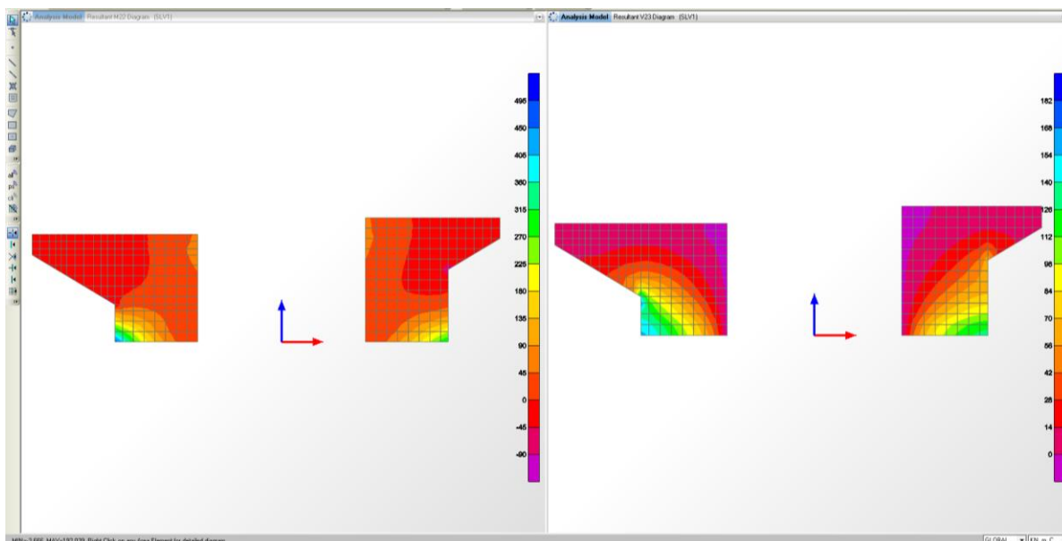
Diagramma dei momenti e dei tagli che tendono le fibre verticali – SLV
