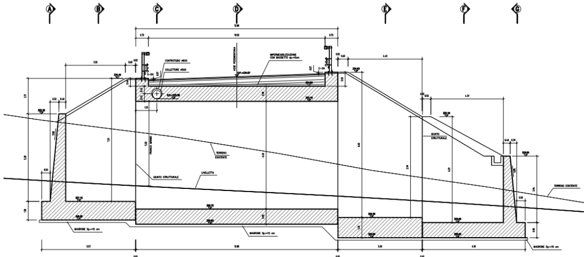
Figura 1.2 – Profilo
