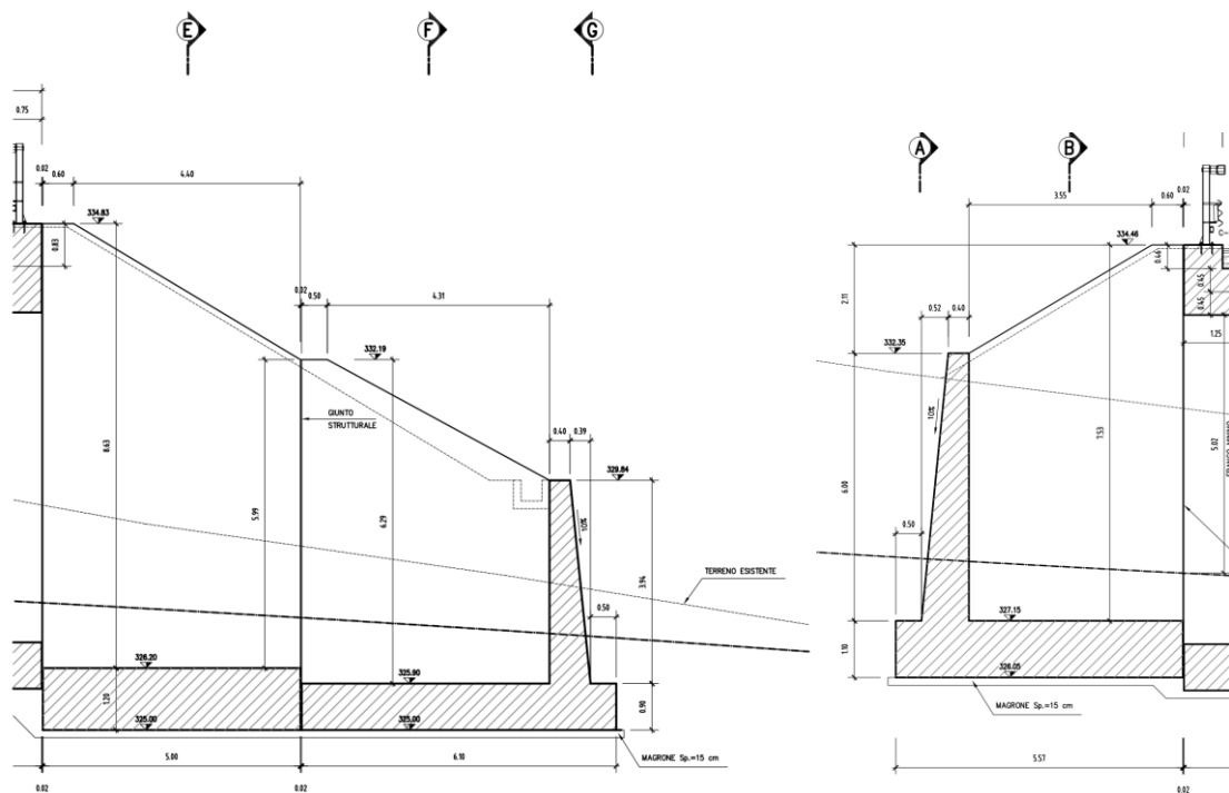
Figura 1.4 – Sezioni trasversali (Concio 1, 2 e 3)
