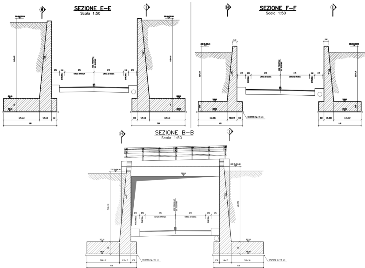
Figura 1.3 – Sezioni trasversali
