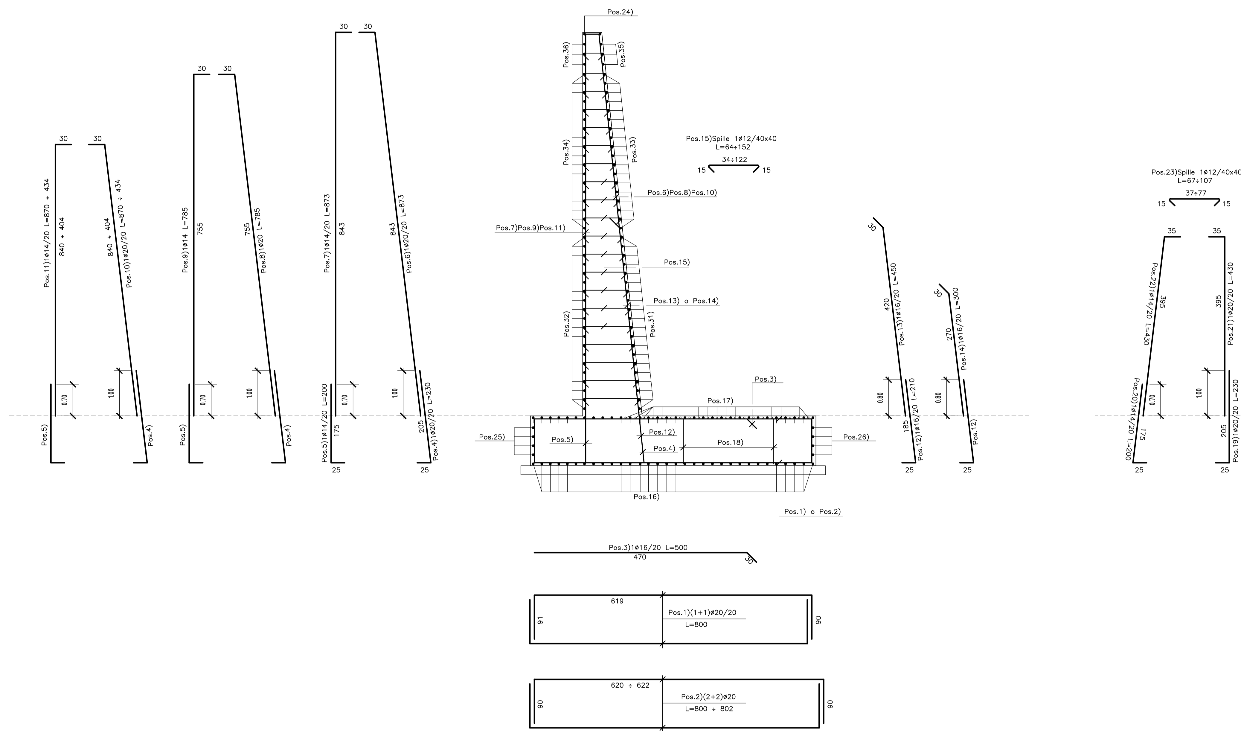
SEZIONE "1-1" Scala 1:50
