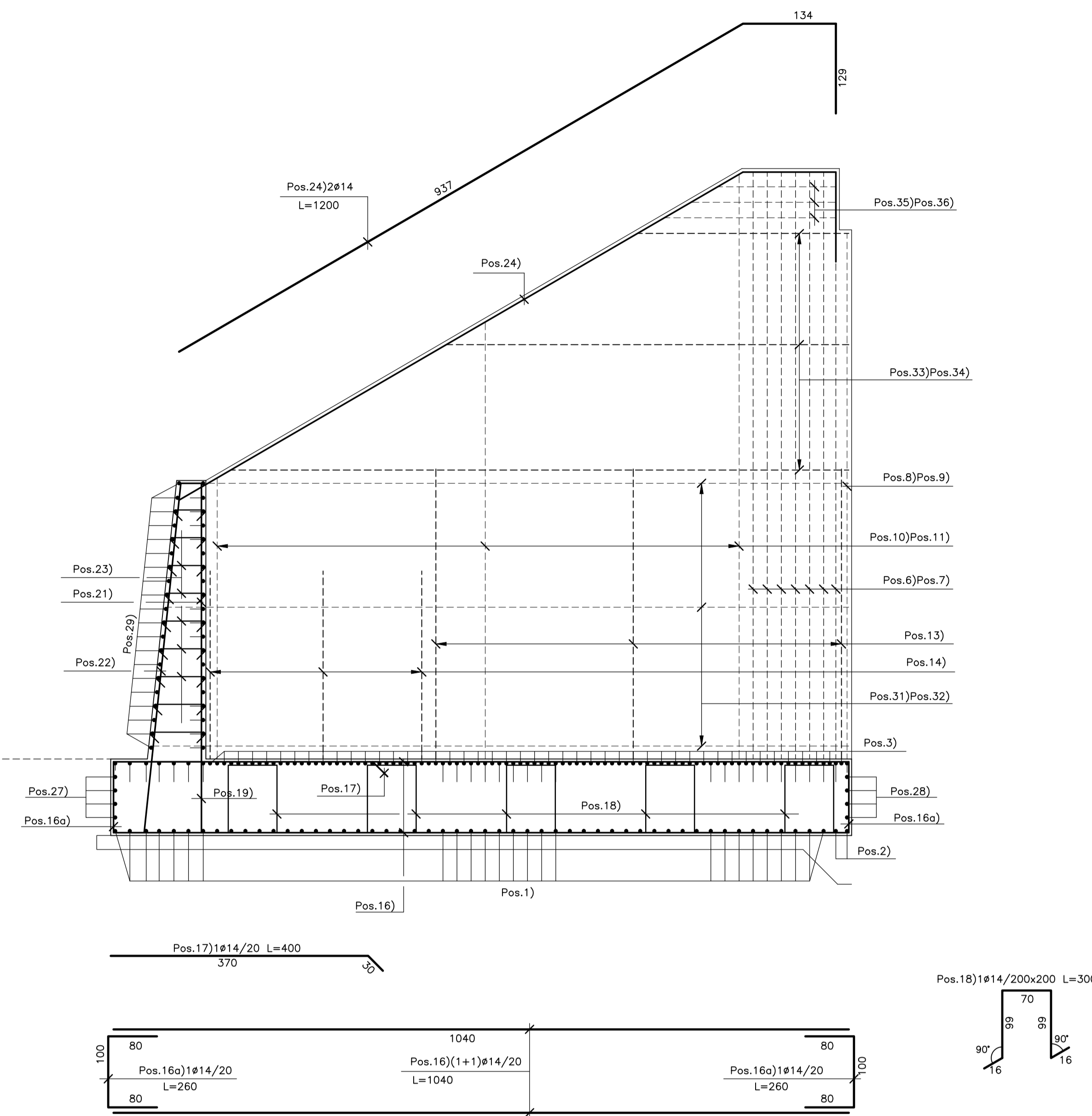
SEZIONE "2-2" Scala 1:50
