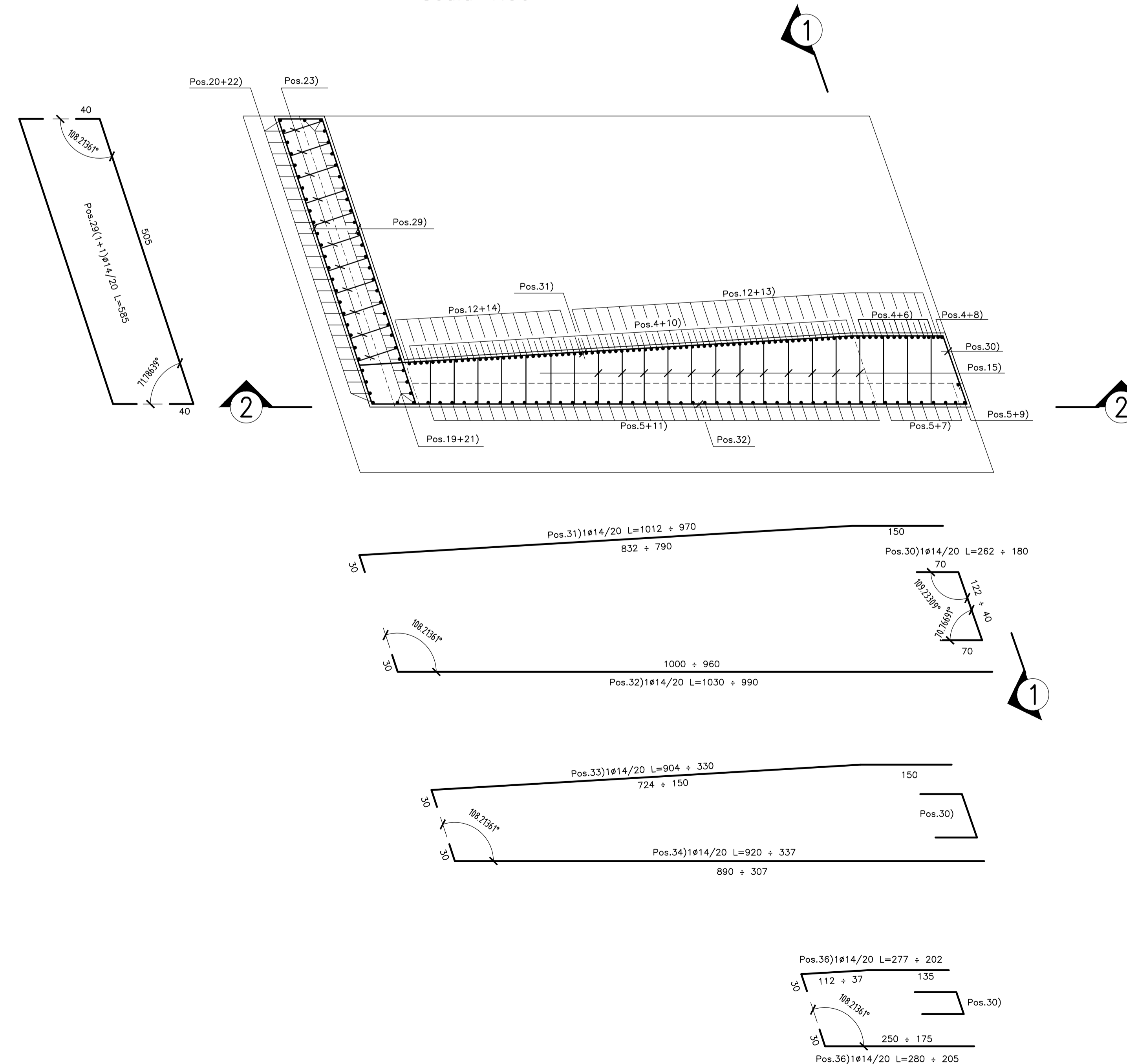
PIANTA ALLO SPICCATO Scala 1:50
