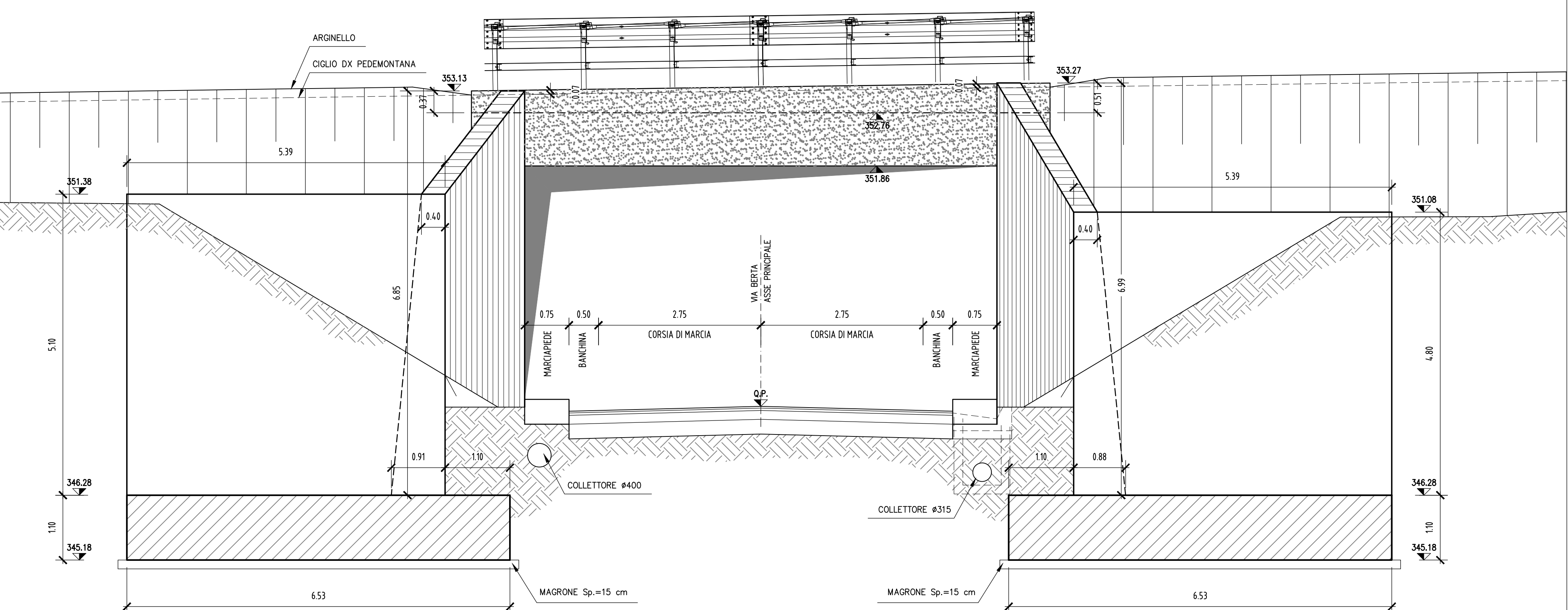
PROSPETTO A-A Scala 1:50
