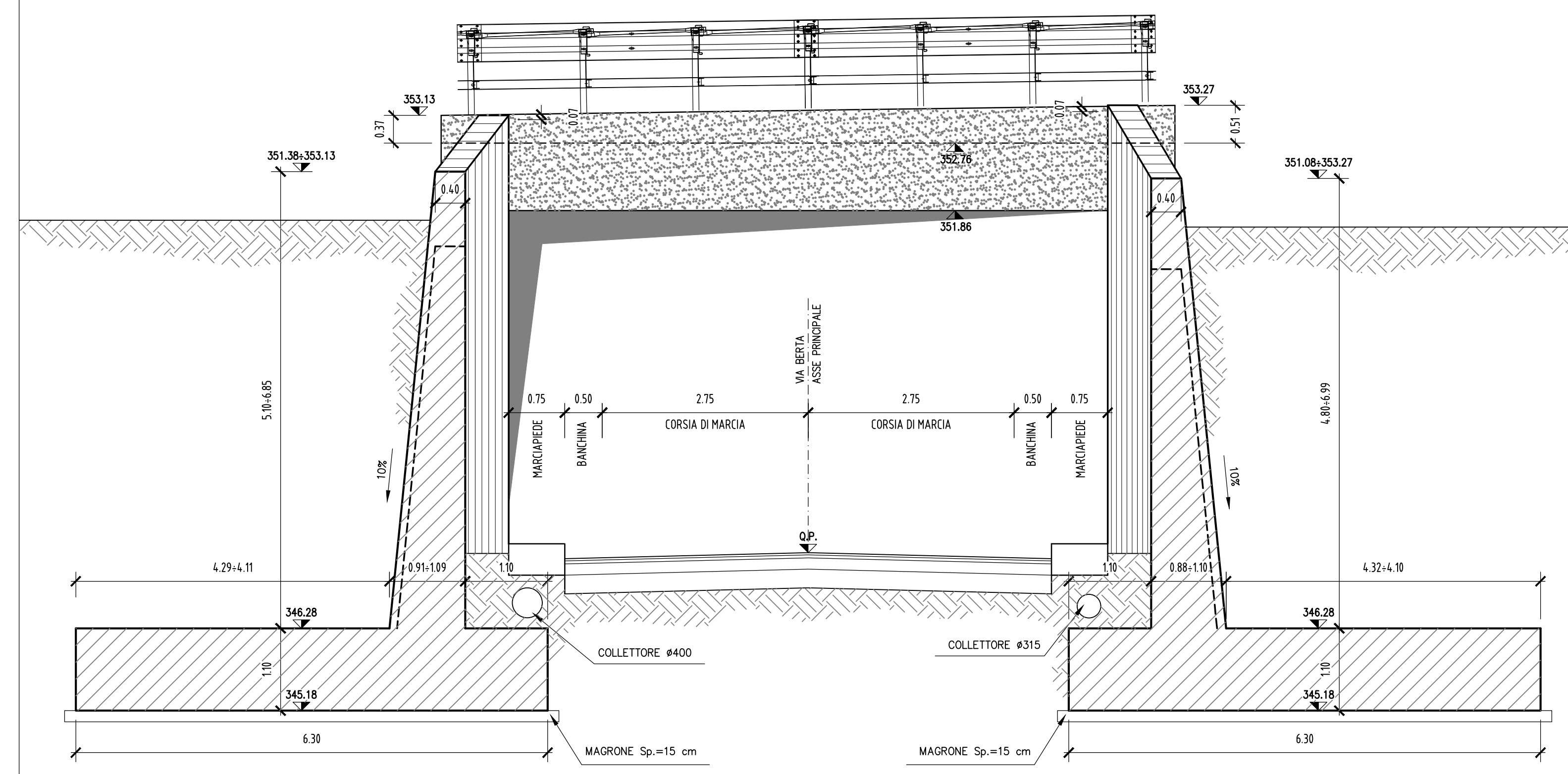
PROSPETTO B-B Scala 1:50
