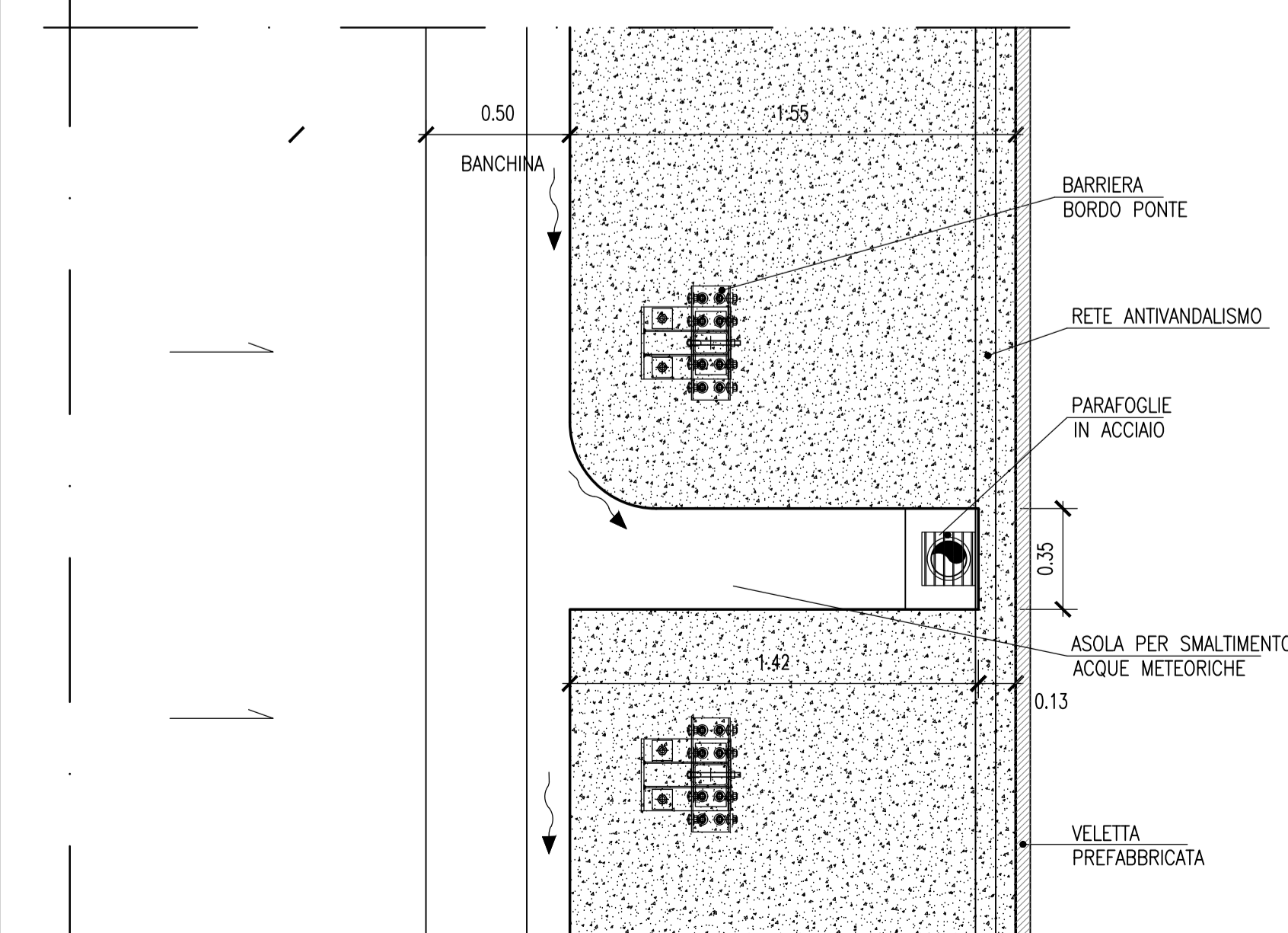
PIANTA Scala 1:20
