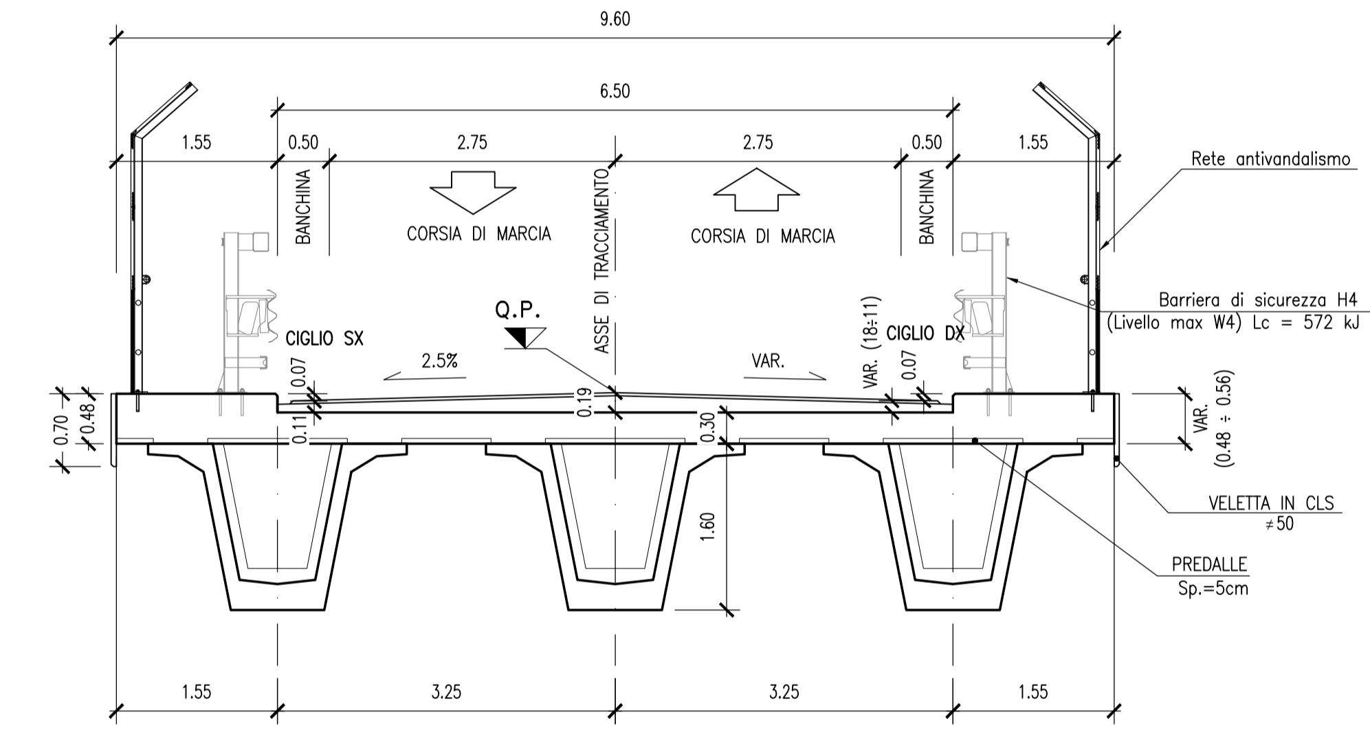
SEZIONE TIPO IMPALCATO Scala 1:50
