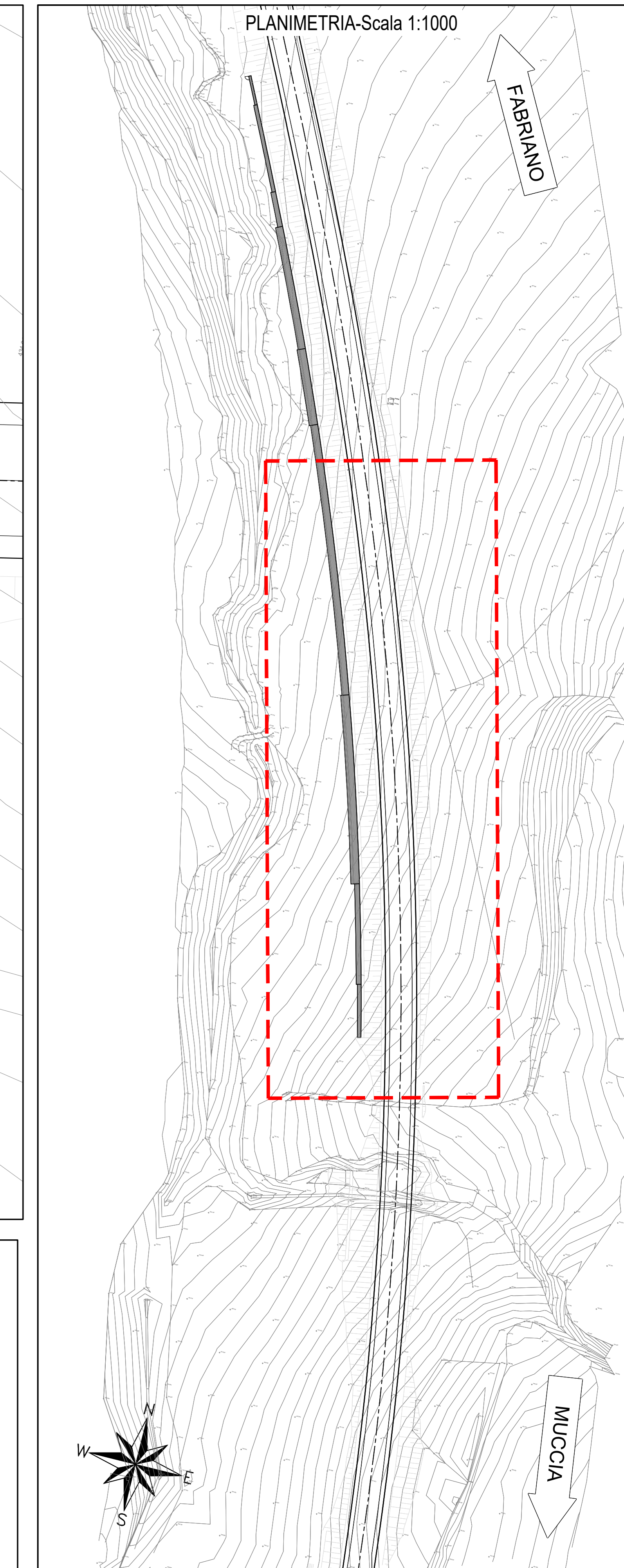
PLANIMETRIA-Scala 1:1000
