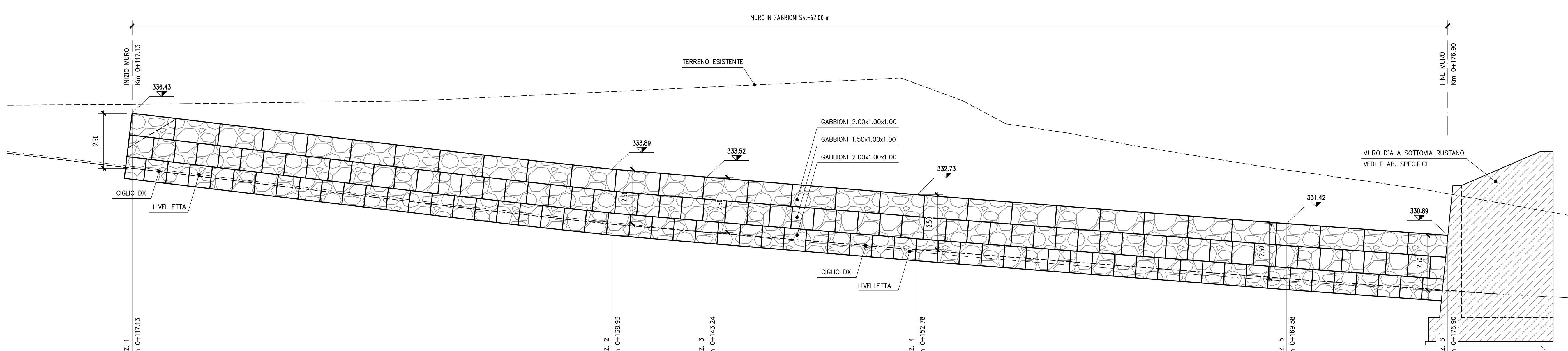
SEZIONE LONGITUDINALE MURO IN GABBIONI Scala 1:100
