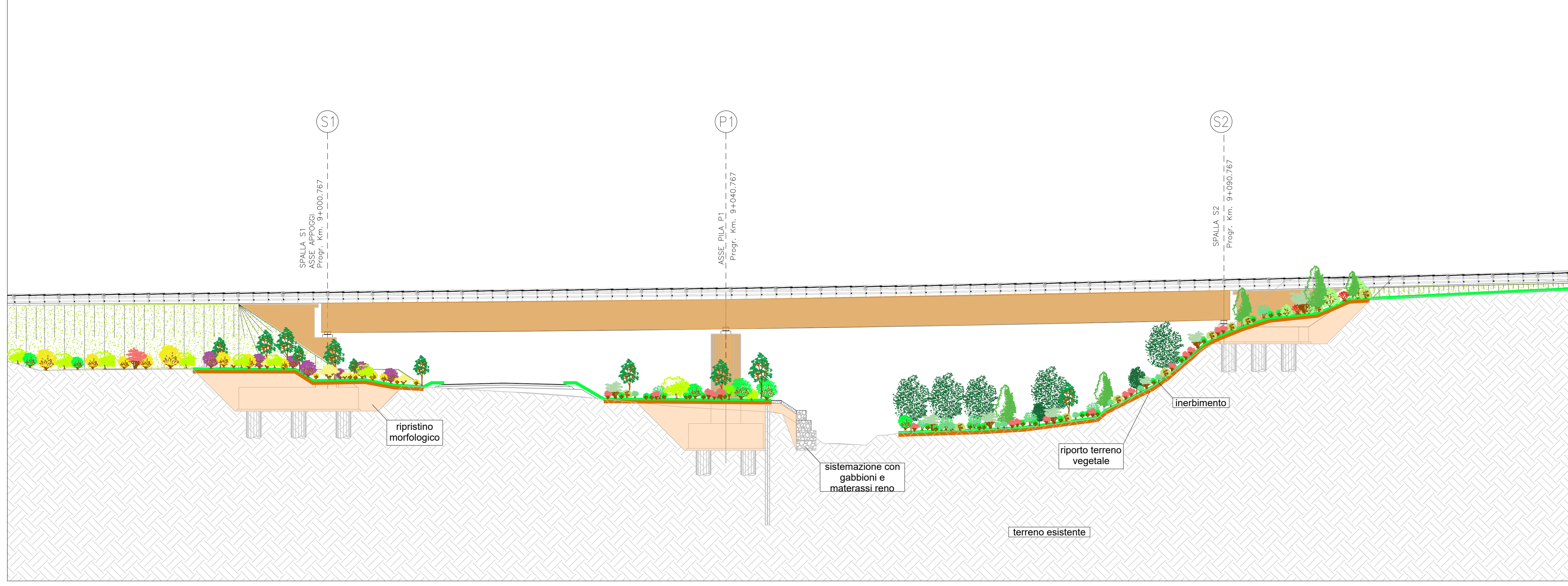
B Vista longitudinale Viadotto Cesara Scale: 1:200
