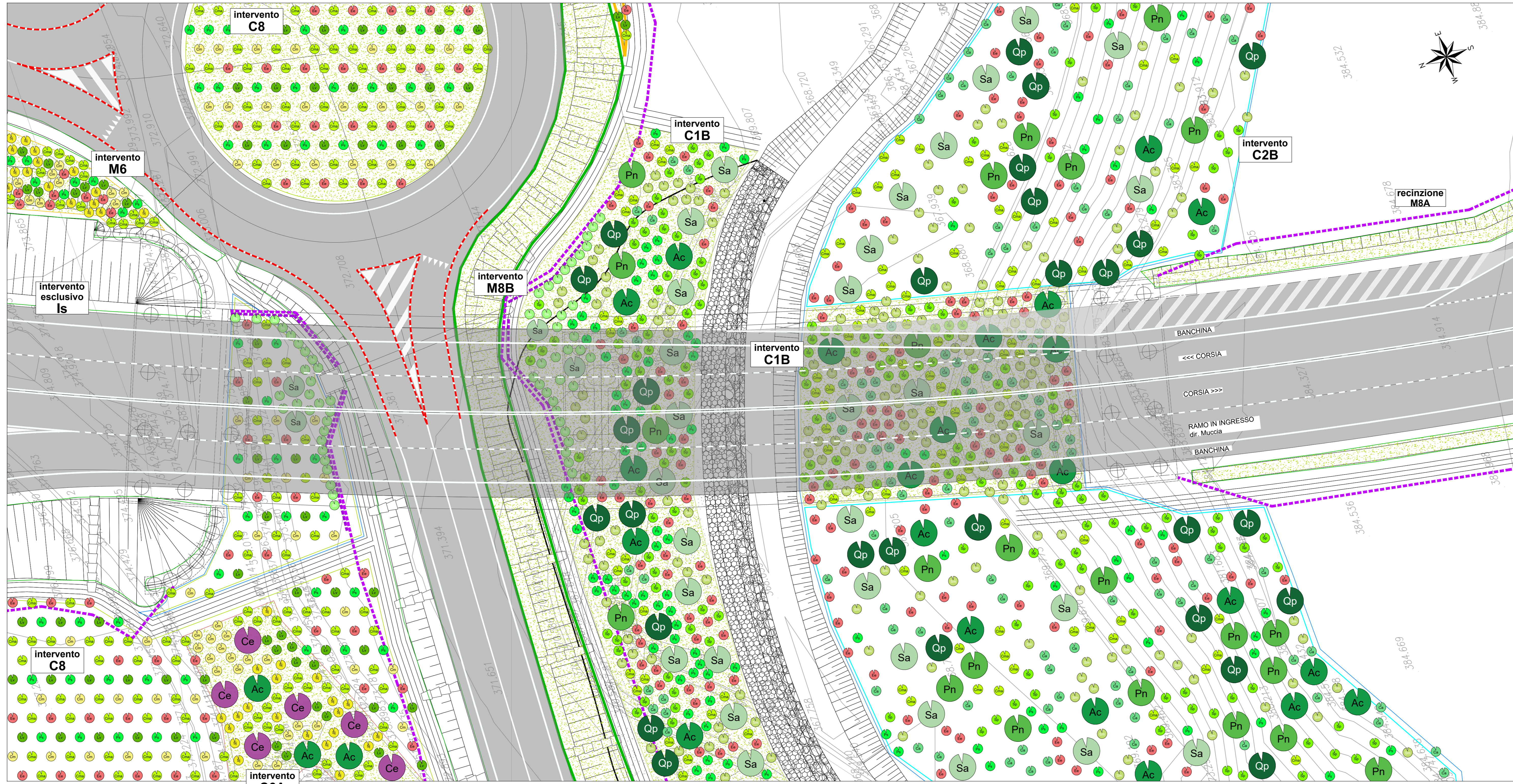
A Planimetria Viadotto Cesara Scale: 1:200
