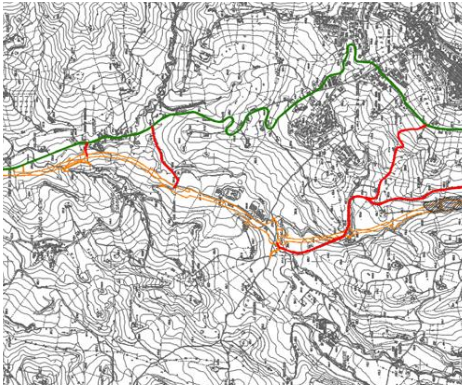
Viabilità di cantiere - 2/3
