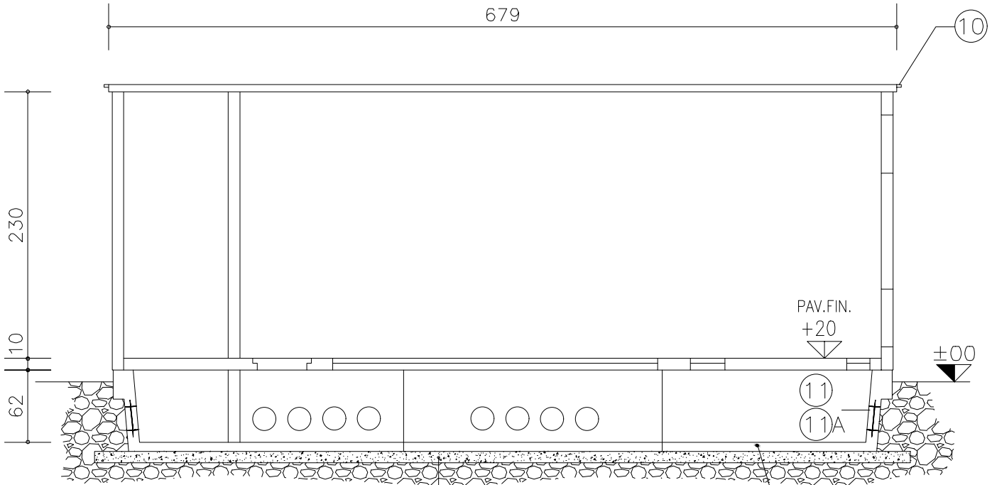
SEZIONE X-X
