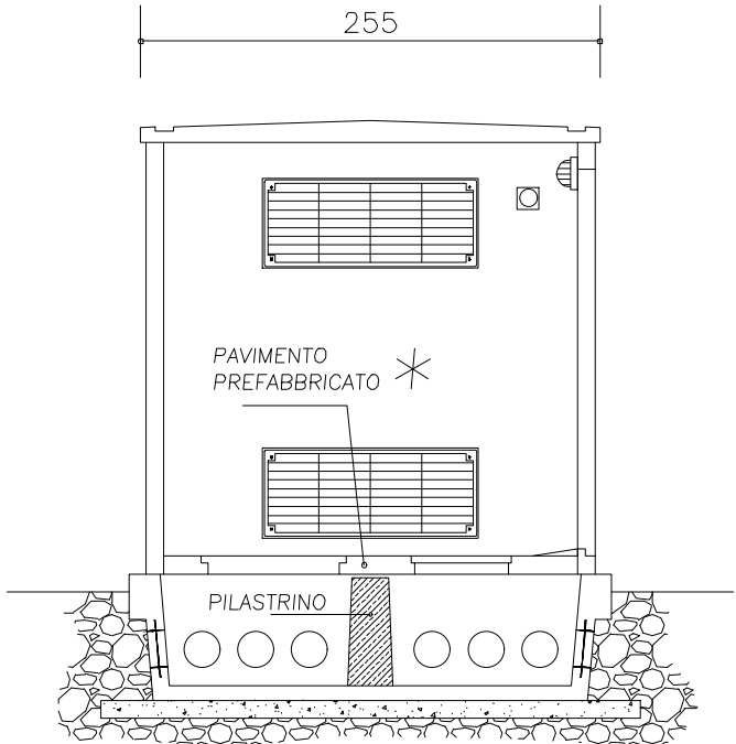
SEZIONE Y-Y
