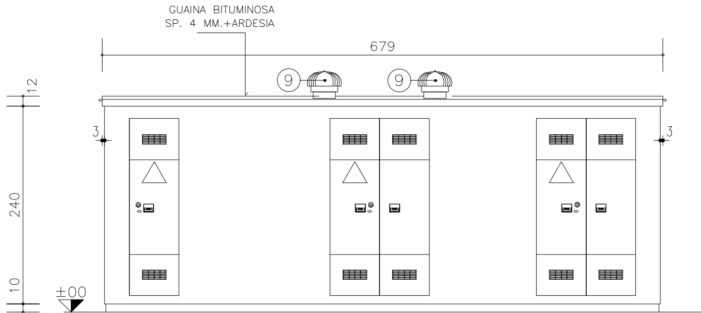
PROSPETTO A
