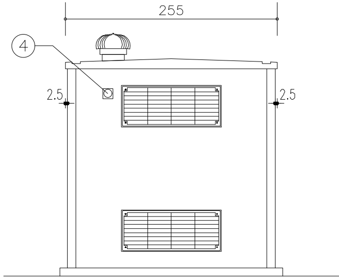
PROSPETTO B
