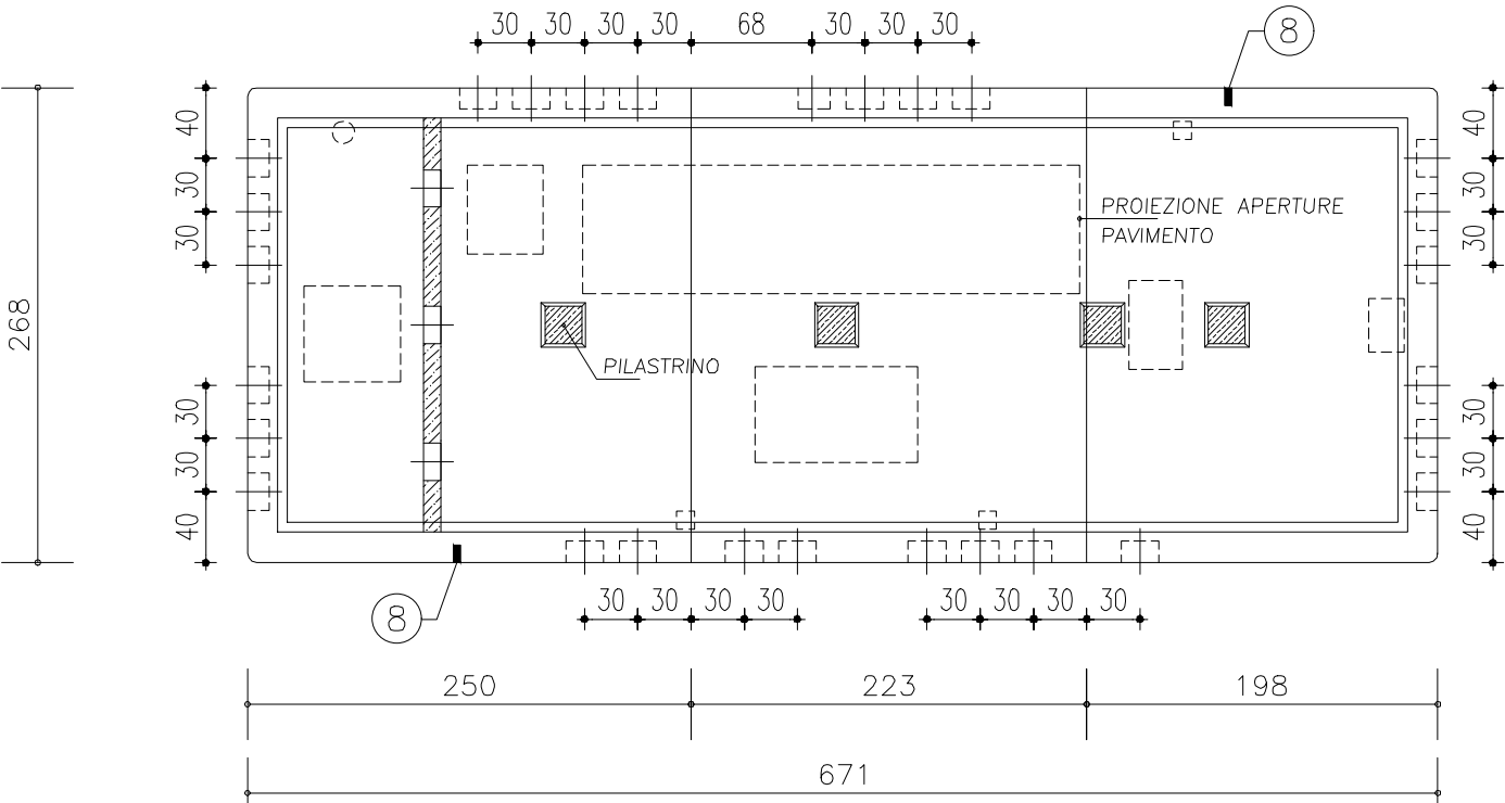
PIANTA VASCA
