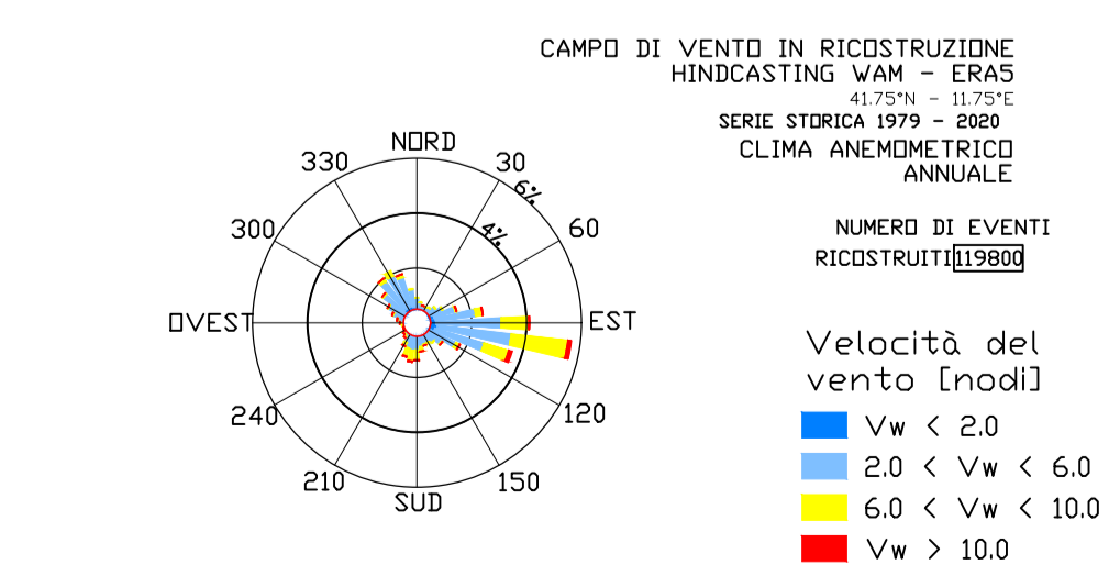
DISTRIBUZIONE DIREZIONALE DEGLI STATI DI VENTI
