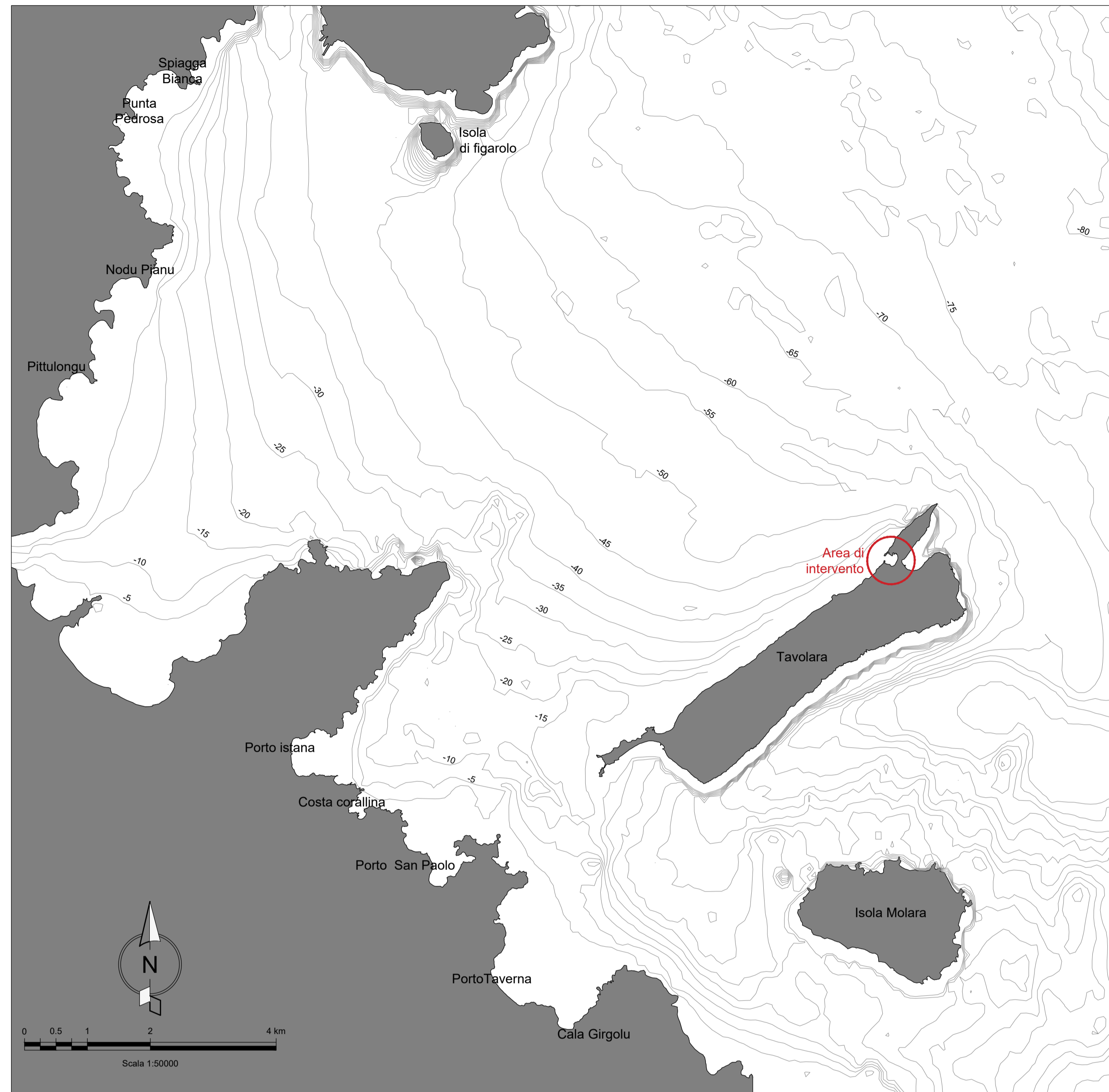
FETCH EFFICACI ISOLA TAVOLARA
