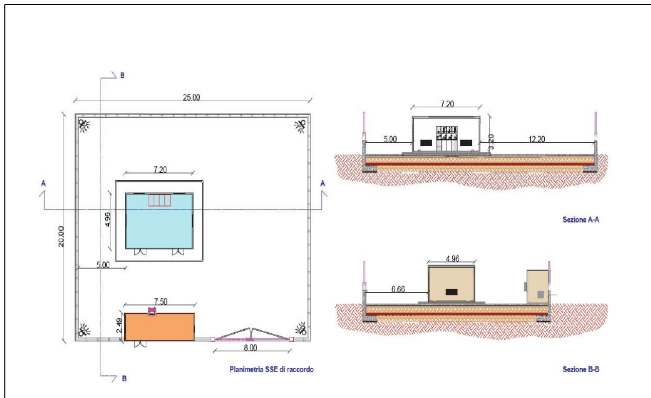
Figura 6.1. – S.S.E. di Consegna.
