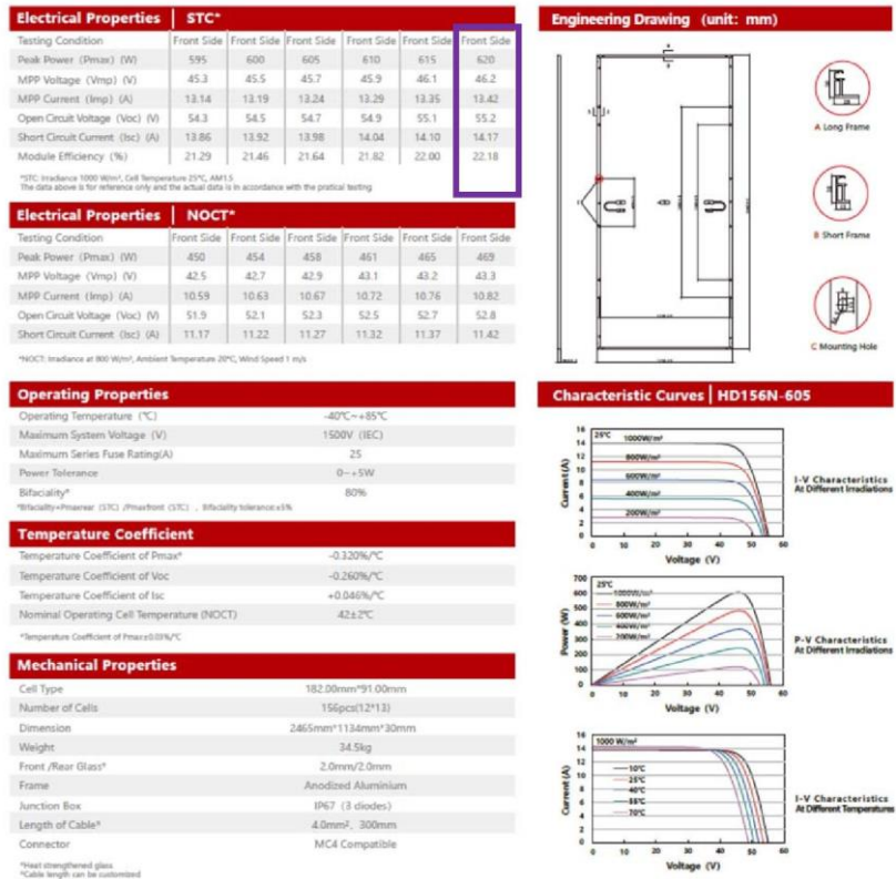
Figura 6.2. – Moduli Fotovoltaici Impianto.
