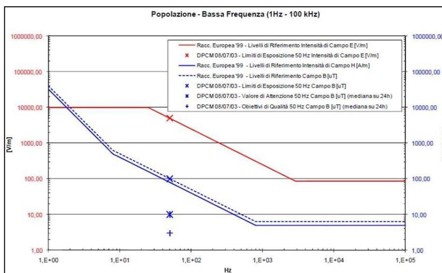
Figura 3.12. – Livelli esposizione Bassa Frequenza (1Hz – 100 kHz).
