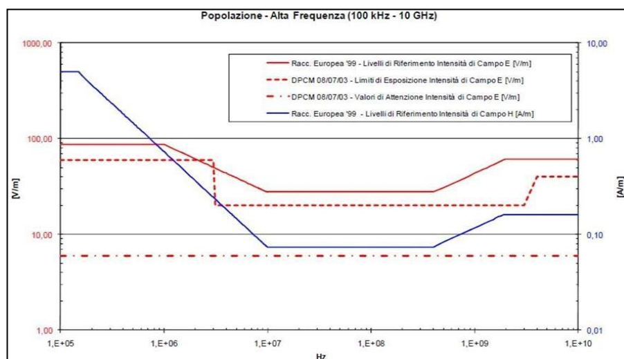
Figura 3.13. – Livelli esposizione Alta Frequenza (100Hz – 10 GHz).
