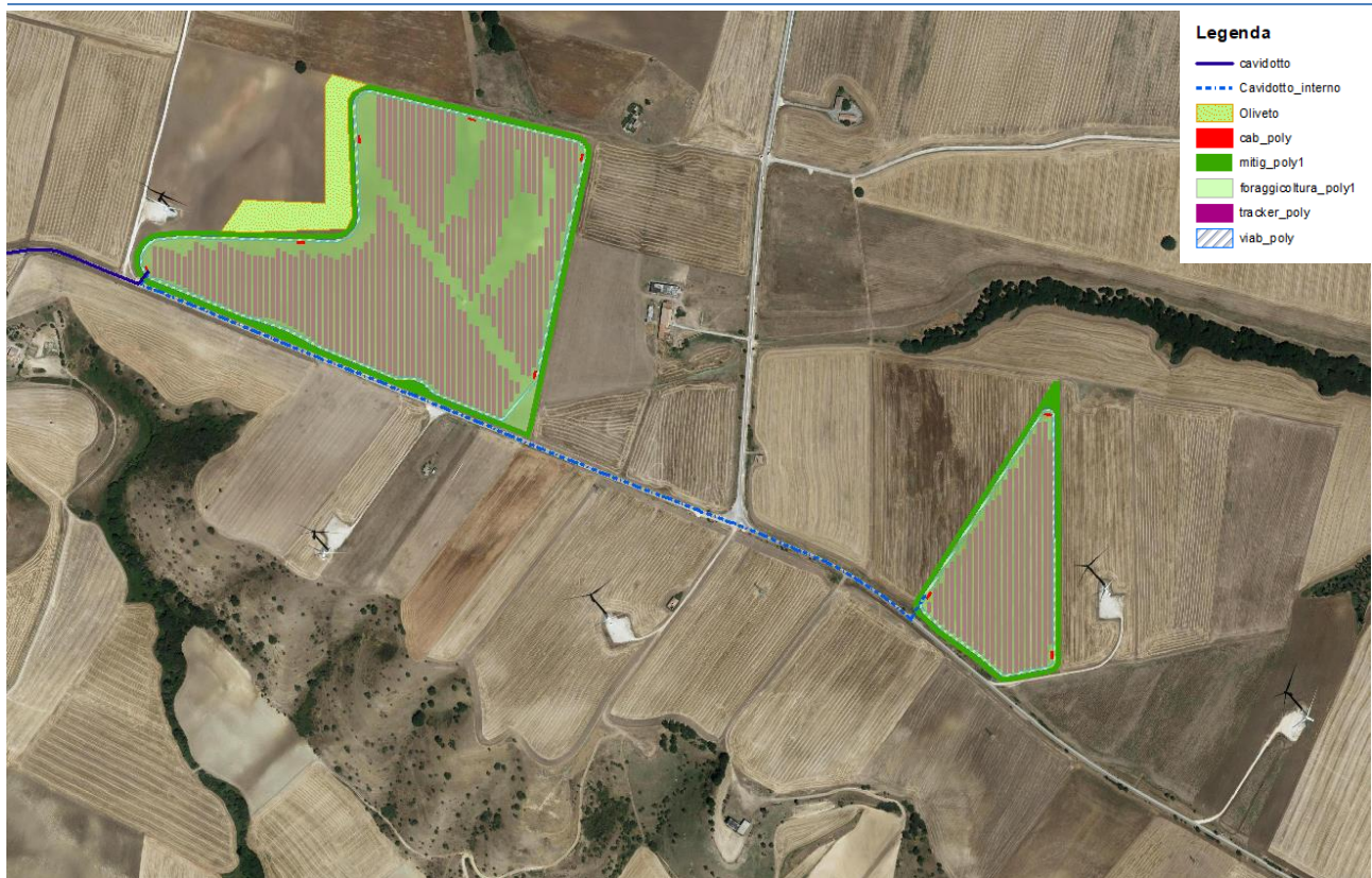
Figura 3.1. – Area di interesse dell’Impianto Agrivoltaico.
