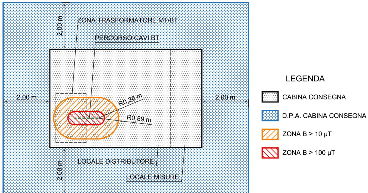
Figura 2 - Zone induzione magnetica cabina di consegna
