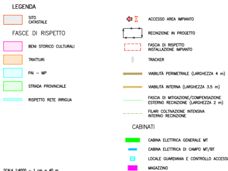
Figura 2.3: Layout di progetto.
