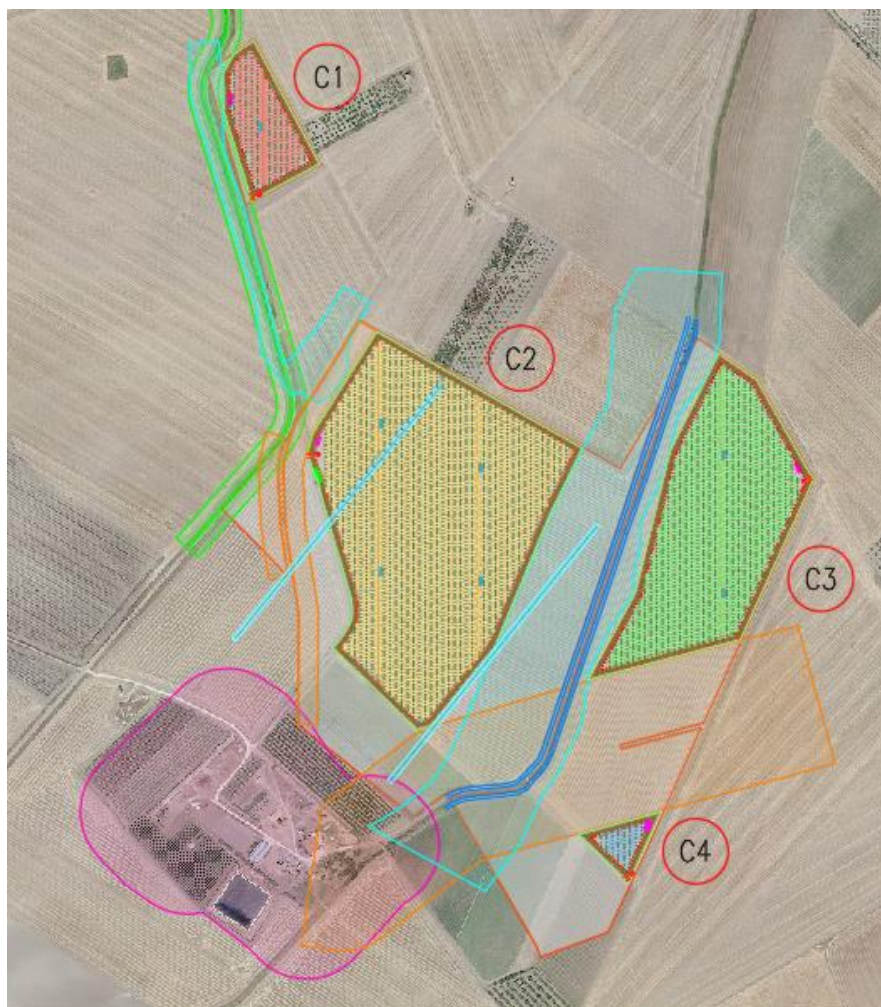
Figura 3.3: Layout di progetto area Sud
