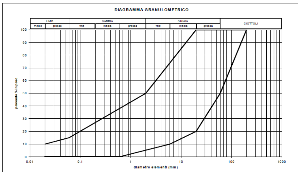
Figura 3.4: fuso granulometrico per materiale da rilevato
