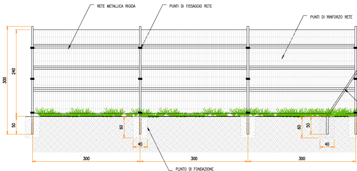
Figura 3.5 - Particolare recinzione
