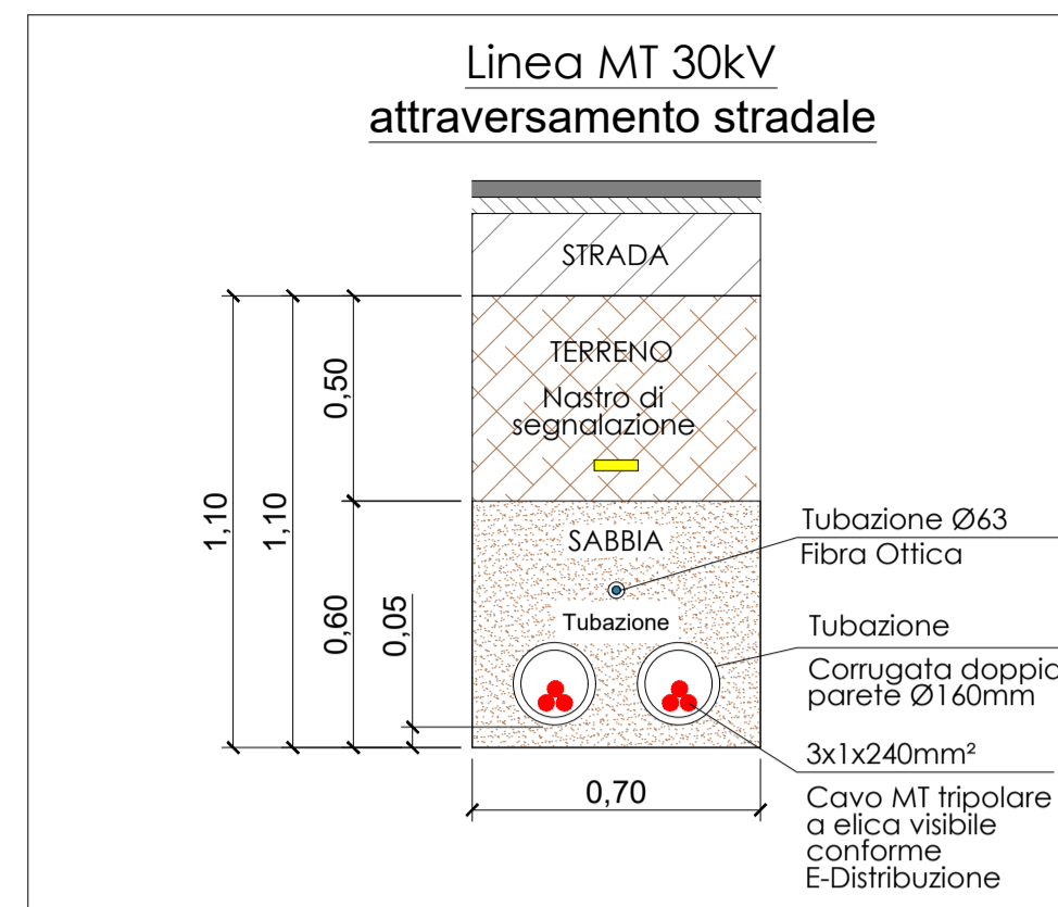
Particolari D,E,F passaggio cavi di Media Tensione- scala 1:20
