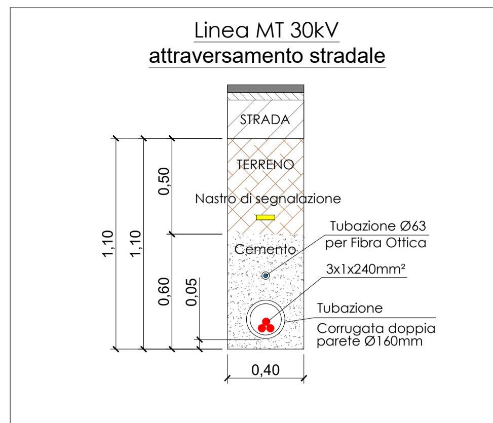
Particolare A passaggio cavi di Media Tensione- scala 1:20
