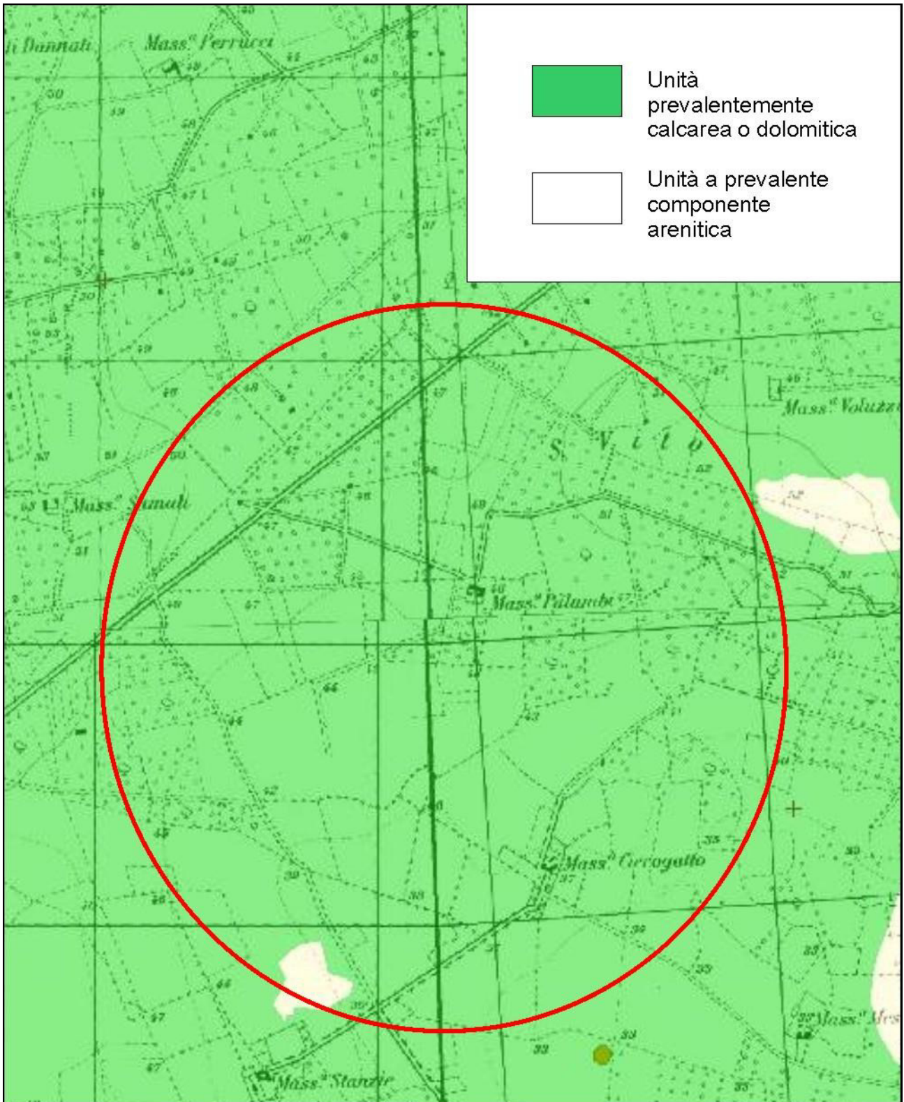
Figura 2. Inquadramento geologico dell'area in esame (Estratto dalla Carta Idrogeomorfologica della Regione Puglia – Fogli 511 e 512, scala 1:25.000).
