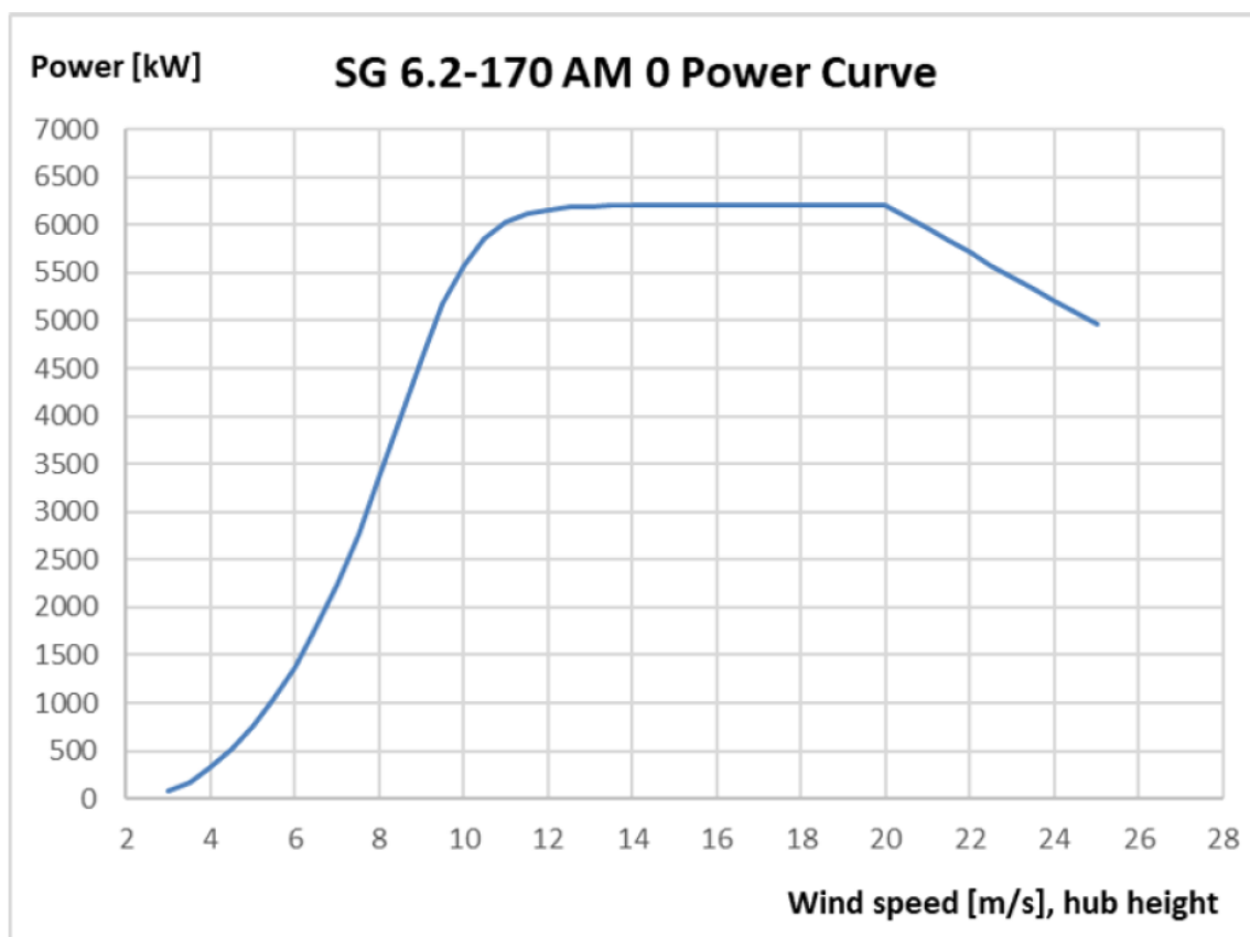
Figura 2.3 – Curva di potenza generatore tipo SG 6.2-170 da 6,2 MW
