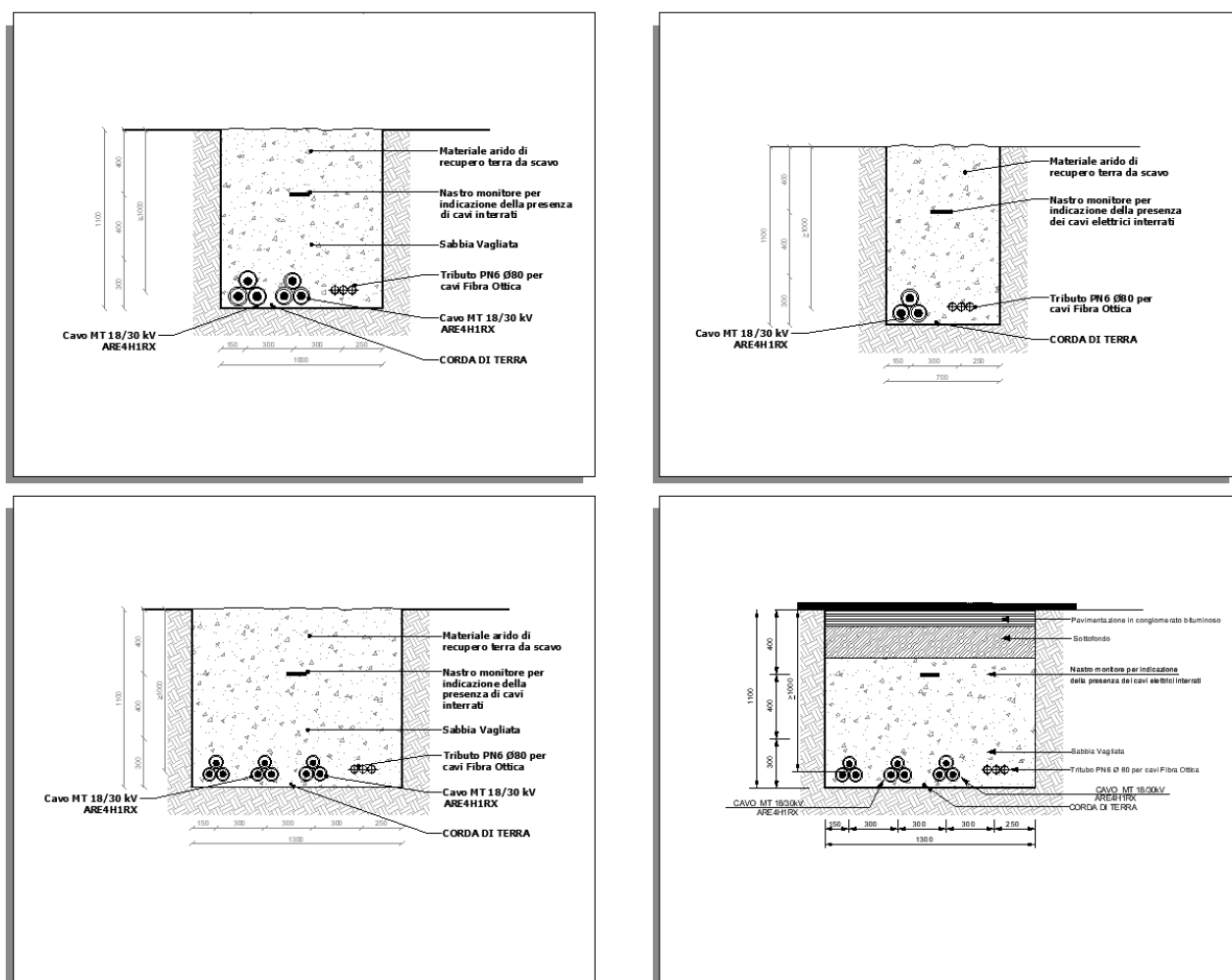
Figura 3.3 – Tipico modalità di posa Cavo MT 30 kV
