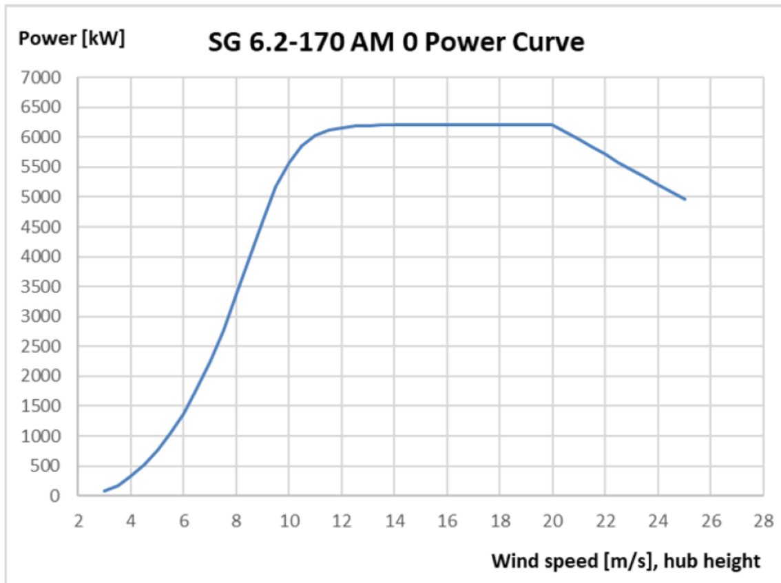
Figura 6.1 – Curva di potenza generatore tipo SG 6.2-170
