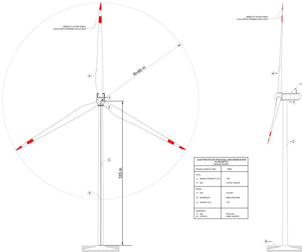
Figura 6.3 – Aerogeneratore tipo SG 6.2-170 altezza al mozzo (1) 125m, e diametro rotore (2) di 170m
