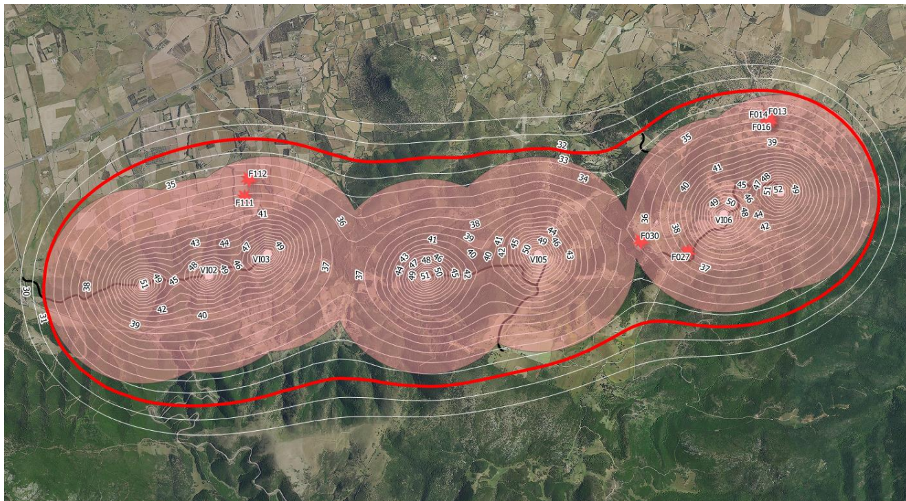
Figura 2.5 – Campo sonoro generato dall'impianto. In rosso l'isofonica dei 32 dBA, attestata ad una distanza indicativa di 1.000 m dalle postazioni eoliche in progetto
